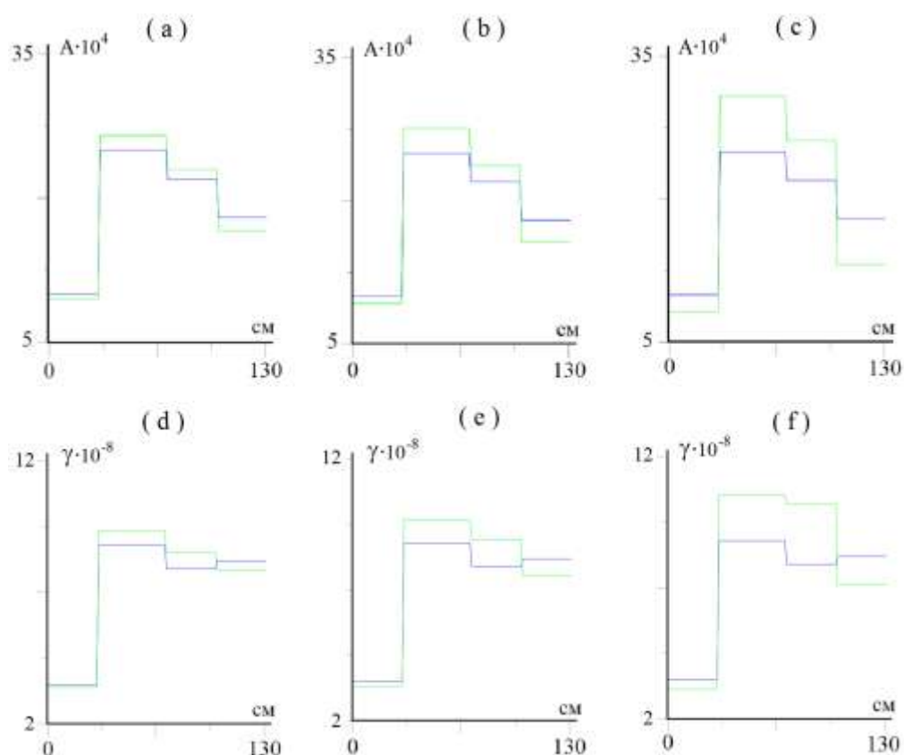
3-расм. а)-с) A , d)-f) \gamma параметрларнинг тикланиши, тескари масала берилганларининг хатолиги а), d) 3%, b), e) 5% ва c), f) 10%. Аниқ қийматлар кўк чизиқ билан, тикланган қийматлар яшил чизиқ билан берилган.
