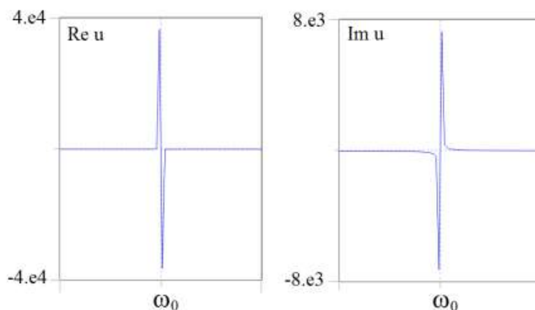
Рис. 1. Поведение величины u(0, p) при изменении параметра \omega в окрестности \omega_0 .
