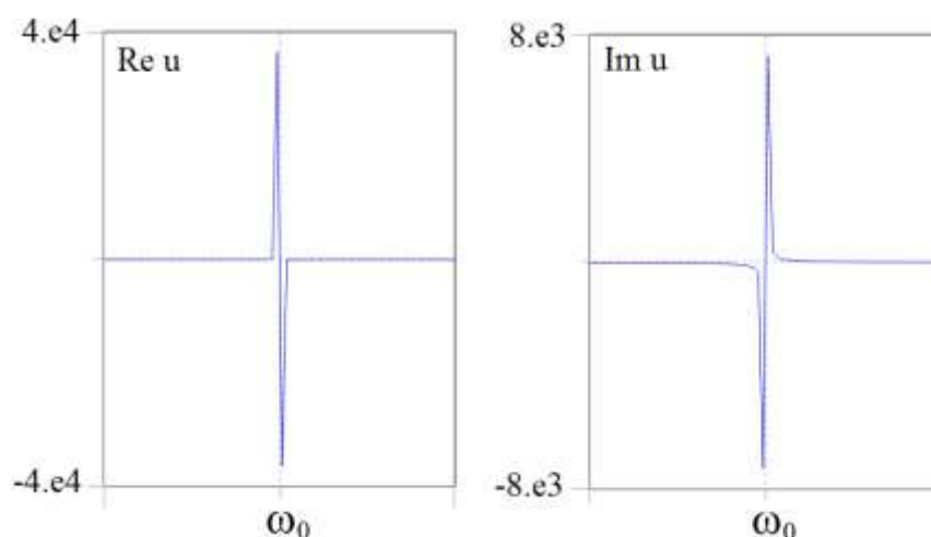
1-расм. \omega параметр \omega_0 атрофида ўзгарганда u(0, p) микдорнинг ҳолати.
