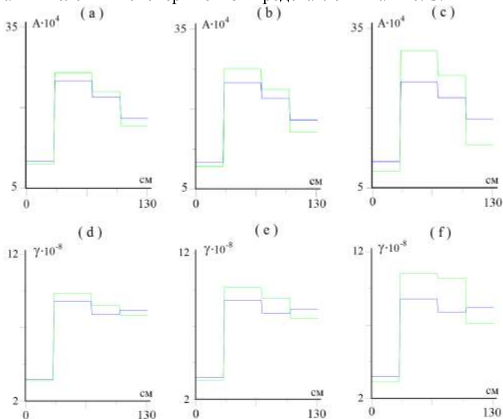
Рис. 3. Примеры восстановления параметров а)-с) A , d)-f) \gamma ; ошибка в данных обратной задачи а), d) 3%, b), e) 5% и c), f) 10%. Точное значение дано синей линией, восстановленное – зелёной.
