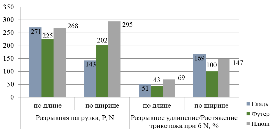
Рис. 13. Гистограмма показателей разрывной нагрузки и удлинения
