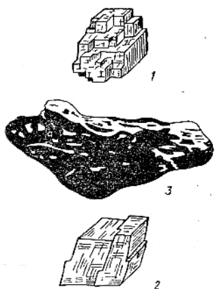
2.4-рaсм. Минералларнинг бирикиш тури
