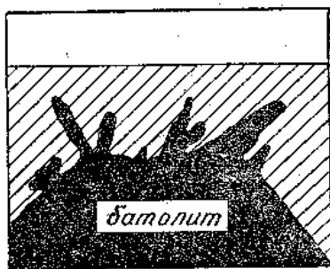
3.1-расм. Магматик жинс-ларинг магмадан шосил боелиш схемаси: 1-чушурликдаги 2-ер устига чикиб колганлари.
