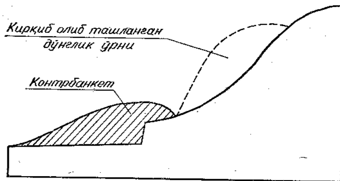
6.4 – расм. +ияликларни яссилаб ва контрбанкет +уриб уларнинг мустацкамлигини ошириш схемаси.
