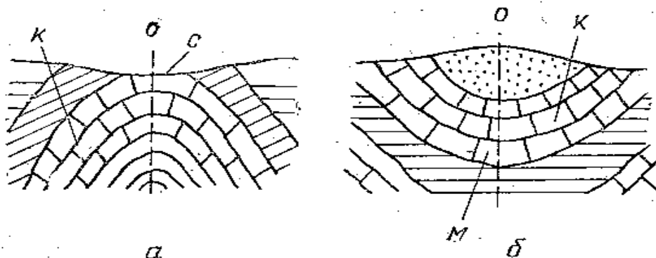
7- rasn. Букилмалар ва уларнинг элементлари: а-антиклинал; б-синклинал; К-карбонат; О-букилмалар ўқи; С-аграв; М-мульда.
