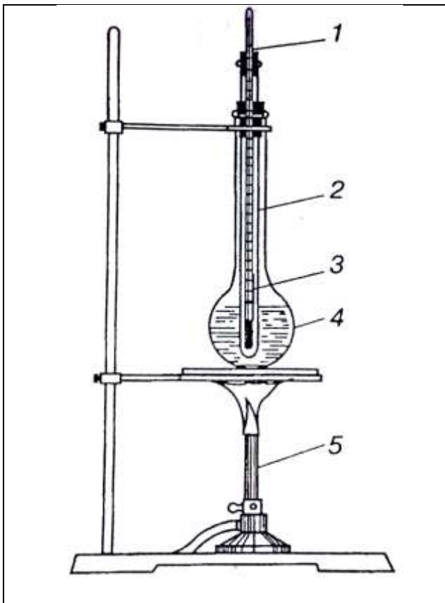
1-rasm. Suyuqlanish haroratini o'lchashga mo'ljallangan qurilma.
