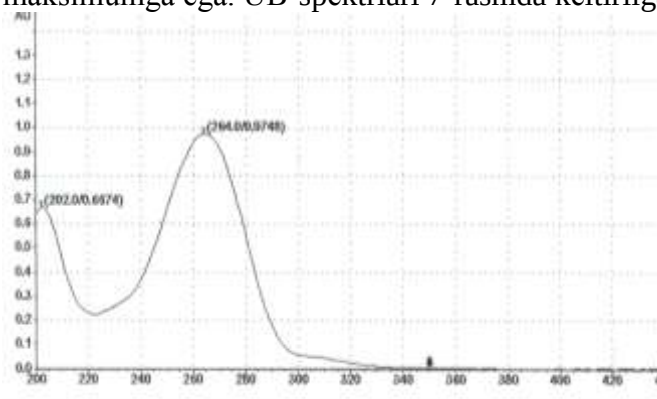
7-rasm. Atsetozalamidning etil spirtidagi UB spektrlari.
