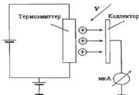
Рис. 2. Сирт ионлашув детектори (СИД)нинг ишлashi tizimi.
