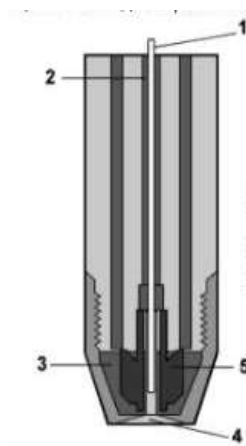
2-rasm. Suyuq membranli elektrod 1-ichki solishtiriluvchi elektrod Ag/AgCl 2- suvli eritma, bo'lakcha ichki qismi to'ldirilgan 3- suyuq organik ionalmashinuvchi 4-organafil membrana 5- membrana prkladkasi
