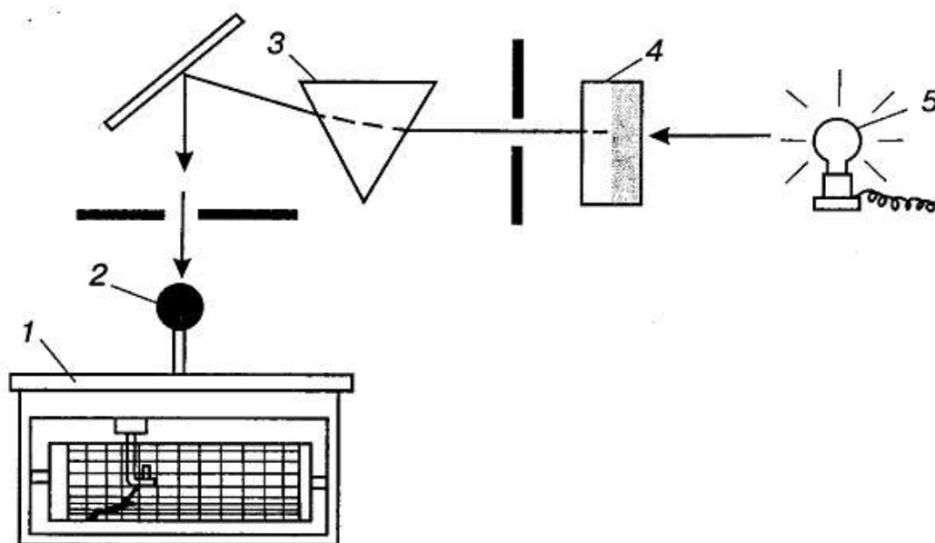
1-rasm. IQ-spektrometr tuzilishi: 1-yozuvchi qurilma, 2-detektor, 3-natriy xloriddan iborat prizma, 4-tekshiriluvchi prizma, 5-infra qizil nur manbai
