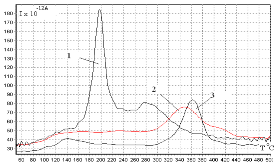
TDSIS usulida olingan spektral natijalari: geksamidin(1), barbital(2) va fenobarbital (3).
