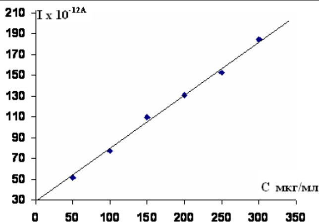
Geksamidinning TDSIS tahlil sharoitlaridagi cho'qqi balandligi va eritma konsentratsiyasiga bog'liqlik chizmasi
