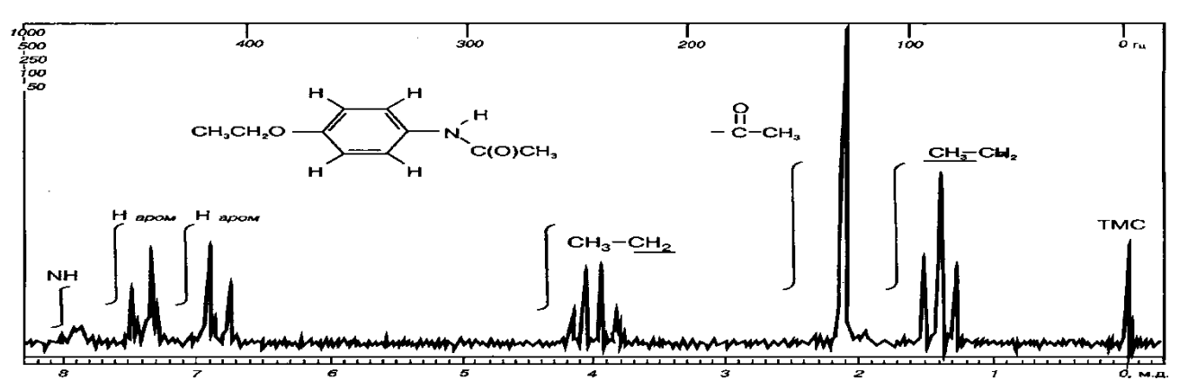
1-rasm.YAMR-spektrometr
