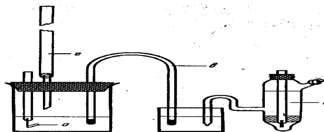
Rasm 10. Potensiometrik titrlashda elektrodning joylashish chizmasi
