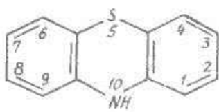
Фенотиазин
