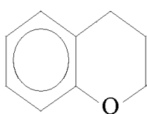
Хроман
