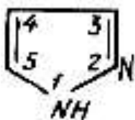
Pirazol
