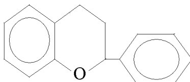
2-фенилхроман
