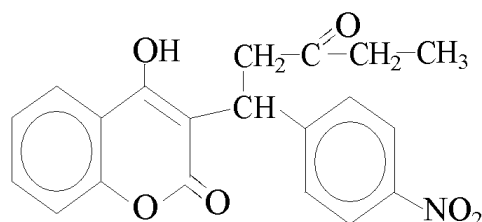
— Nitrofarinum
