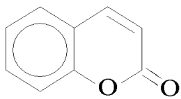
кумарин
