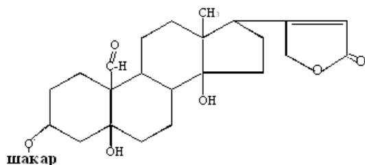
- strofantidin
