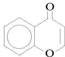
хромон
