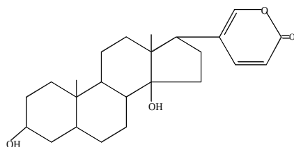
Stsillyarenin
