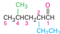
2-etil-4-metil pentanal
