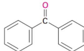
benzofenon
