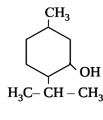
ментол
