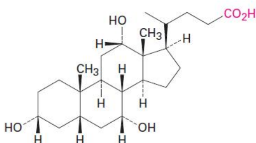
Xoli kislota
