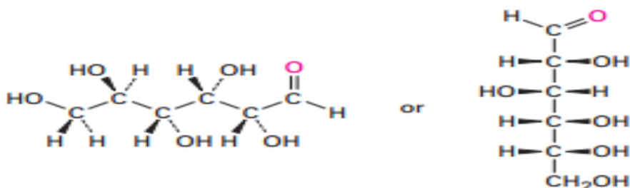
glyukoza(dekstroza)
