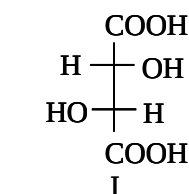
(+)-vino kislota
