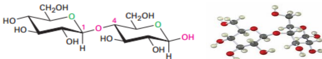
sellobioza
