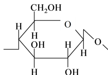
Sellyuloza elementlar
