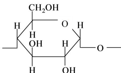
Kraxmal elementlar
