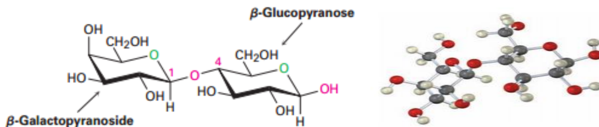
laktoza
