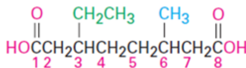
3-etil-6-metiloktan dikislota
