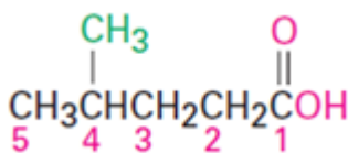
4-metilpentan kislota
