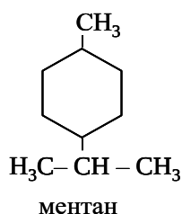
ментан
