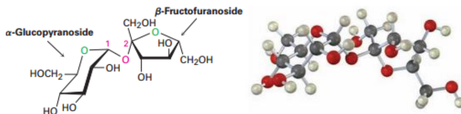
Saxaroza
