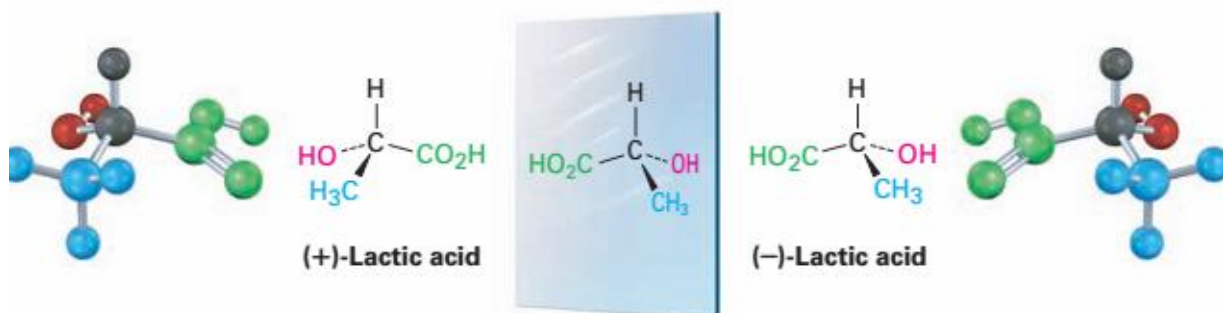
(+)-sut kislotasi
