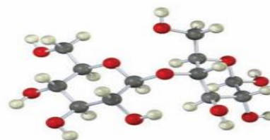
maltoza
