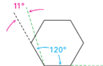
Cyclohexane siklogeksan
