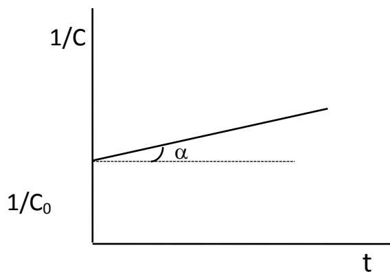
Ikkinchi tartibli reaksiya konsentratsiyasining teskari qiymatining vaqtga bog'liqlik grafigi 10.4 –rasm
