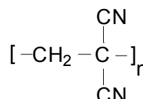
polivinilidentsianid
