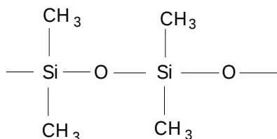
siloksanlar
