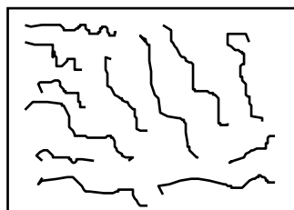
Amorf holat
