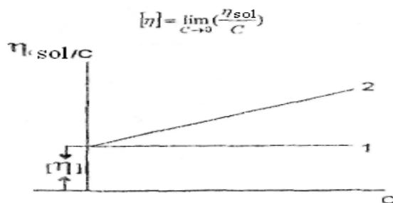
1 - rasm. Eritma keltirilgan qovushoqligini konsentratsiyaga bog'liqlik grafigi:
