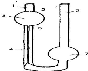
2-rasm. Ostvald viskozimetrining tuzilishi.
