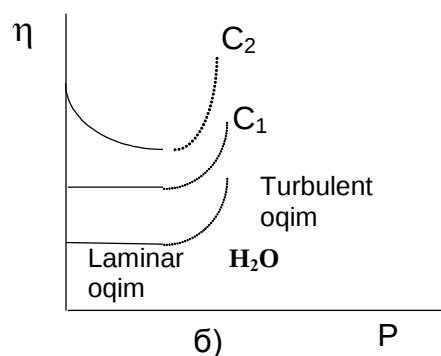
18.1 – rasm. b) Suvning va YuMB eritmasi-ning dinamik qovushqoqlik koef-fitsientini berilayotgan kuchlanishga bog'liqligi.
