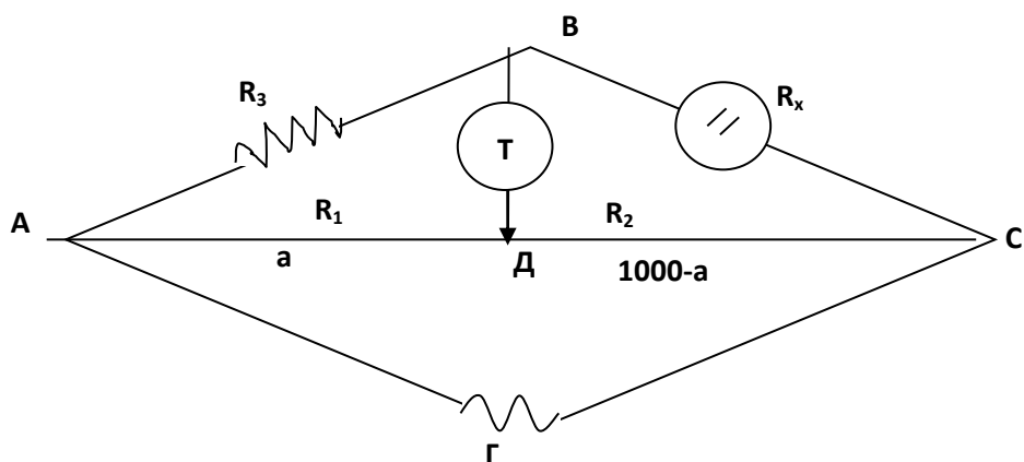
Rasm 2. Kolraush ko'prigi sxemasi.
