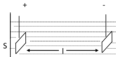
Yaxshi o'tkazgichlar
