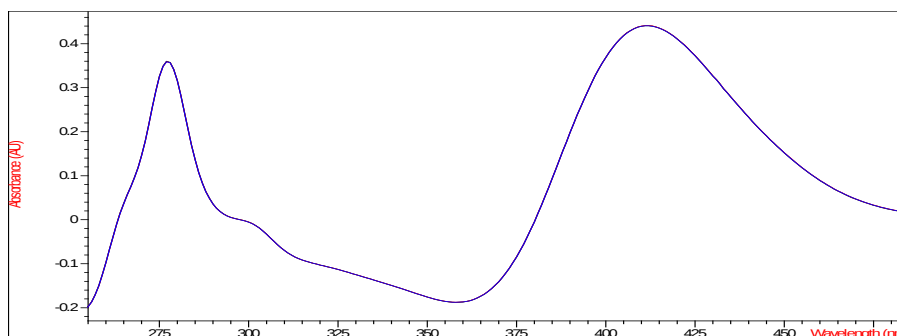
1-rasm. Rutin ishchi standart namunasi UB – spektri
