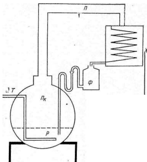
1-rasm. Suv bug'i bilan haydab olish moslamasi.:
