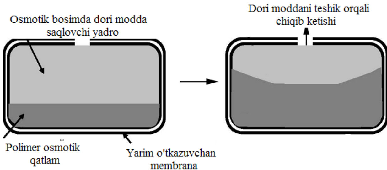
7-rasm. Osmotik nasos sistemalarning tuzilishi (Deen A. va boshq., 2003 )
