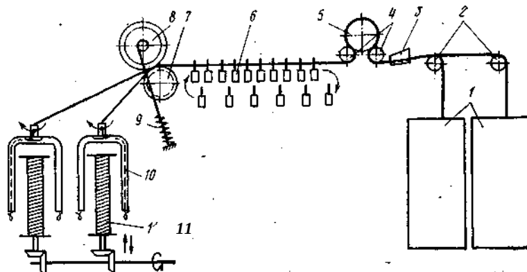
RN-216-L osma rogulkali piliklash mashinasining texnologik sxemasi
