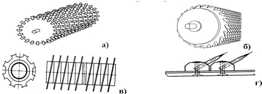
a) pichoqli, b) arrali, v) shakldor tishli diskli, g) ignali panjara
