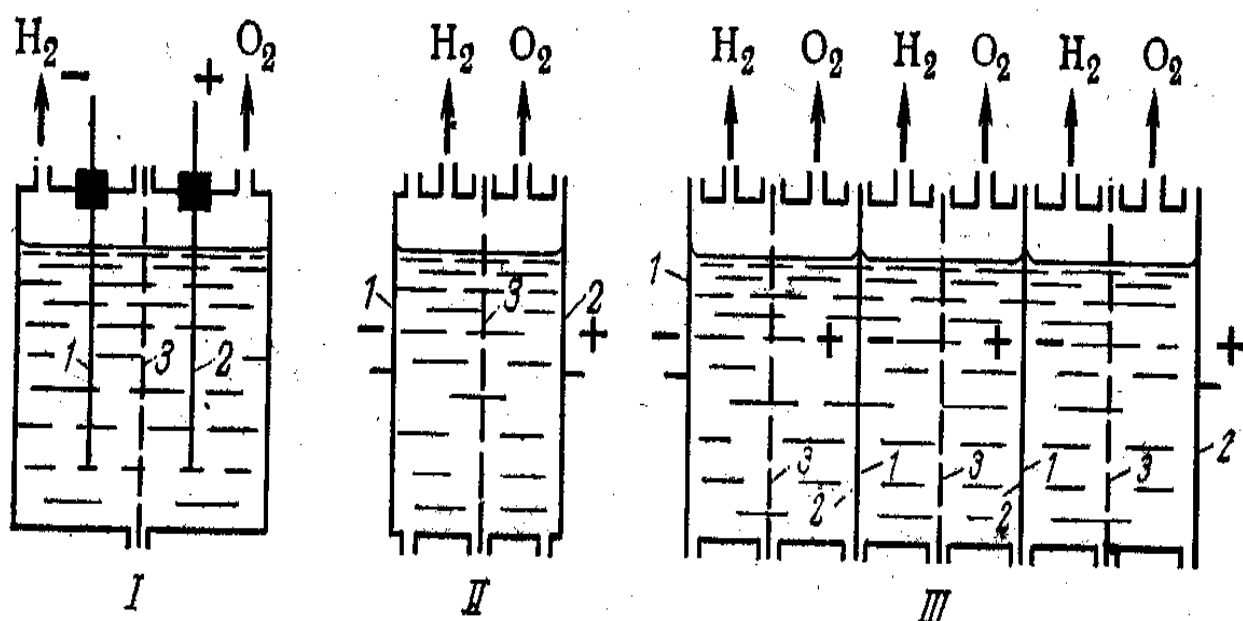
24 – rasm. Monopolyarvabipolyarelektrolizyorqurilmalarningsxemasi.
