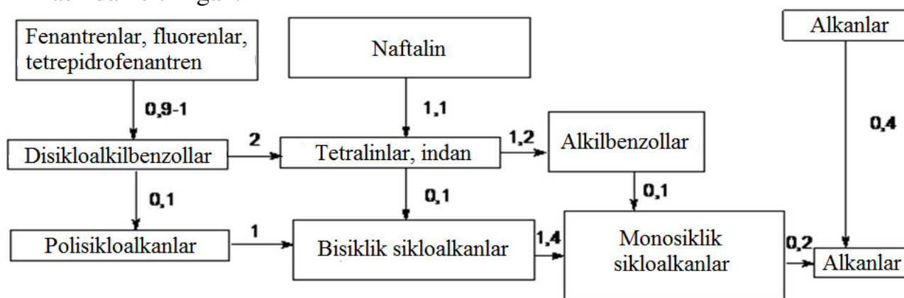
24–rasm. Uglevodorodlarning gidrokreking jarayonidagi o'zgarish sxemasi.
