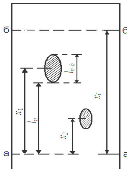
11–rasm. Yupqa qatlamda xromatografiyalash kattaliklarini o'lchash sxemasi.
