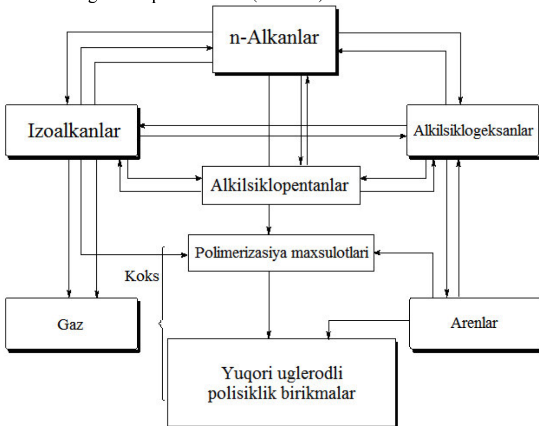
22-rasm. Riforming sharoitida uglevodorodlar o'zgarishlarining sxemasi.
