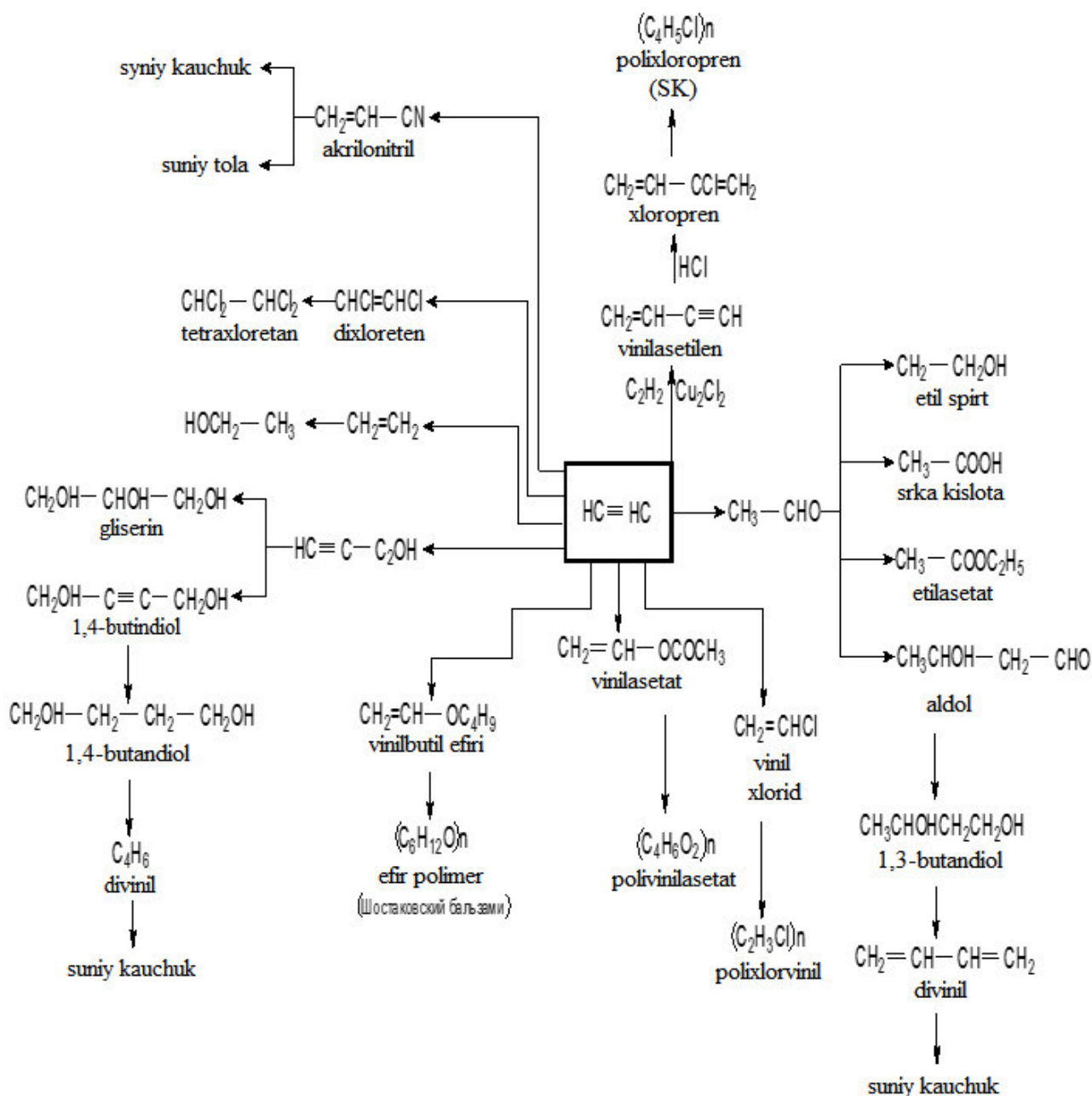
18-rasm. Asetilenni neft kimyosi sanoatida ishlatilishi.
