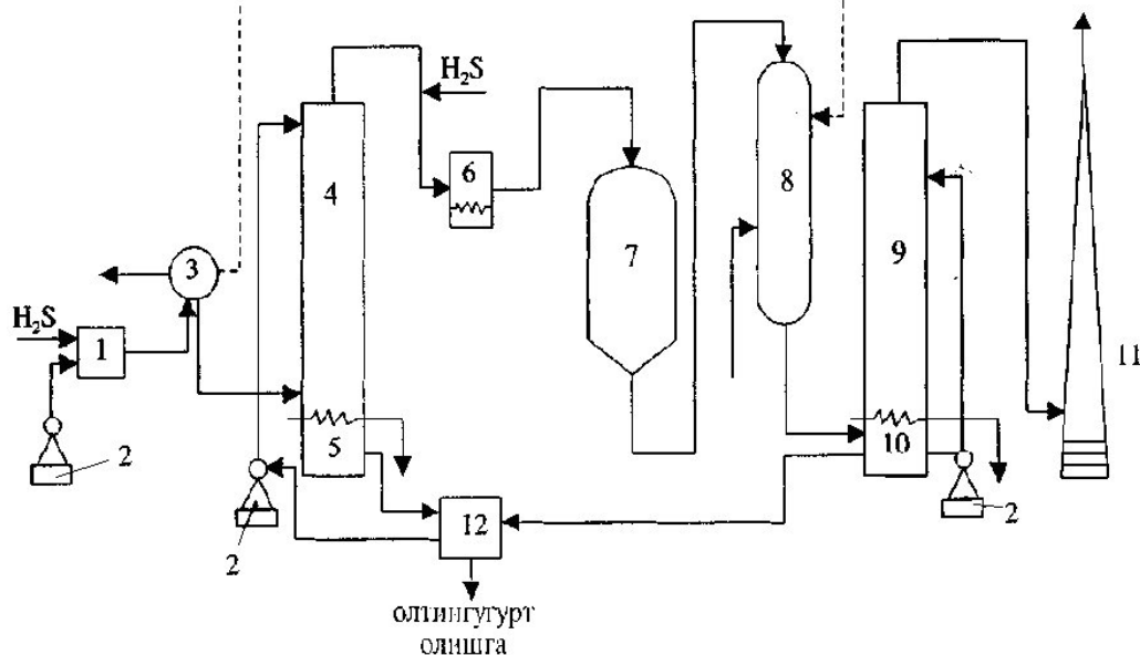
27-rasm. Oltinugurt olish texnologiyasining sxemasi.
