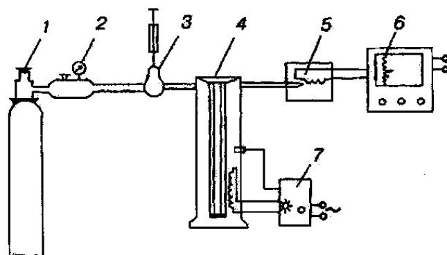
12-rasm. Gaz xromatograf sxemasi.
