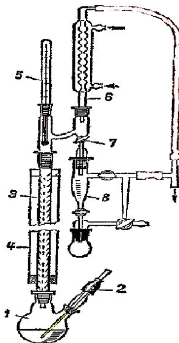
5-rasm. Rektifikatsiyalash qurilmasi:
