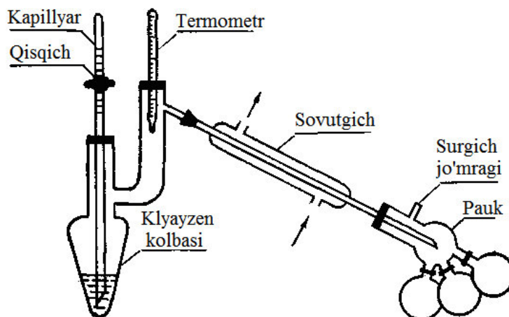
3-rasm. Laboratoriyada vakuumda haydash asbobi
