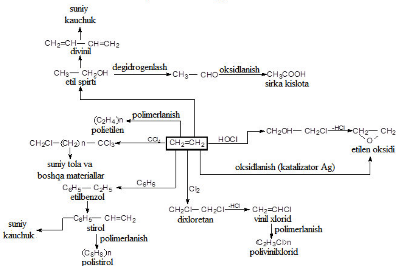
19-rasm. Etilenni neft kimyosi sintezida ishlatilishi.
