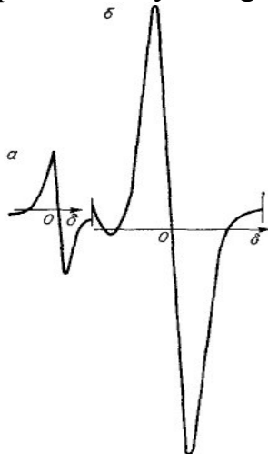
9-rasm. Etalon va neftning EPR spektri
