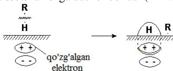
21-rasm. Uglevodorod molekulalarining yuzasidagi erkin elektronlar.
