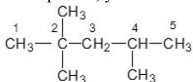
2,2,4-trimetilpentan (izooktan)
