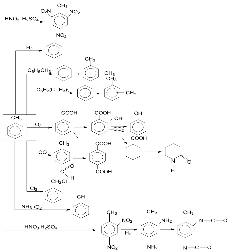
17-rasm. Neftikimyo sanoatida toluolni ishlatilish sohalari
