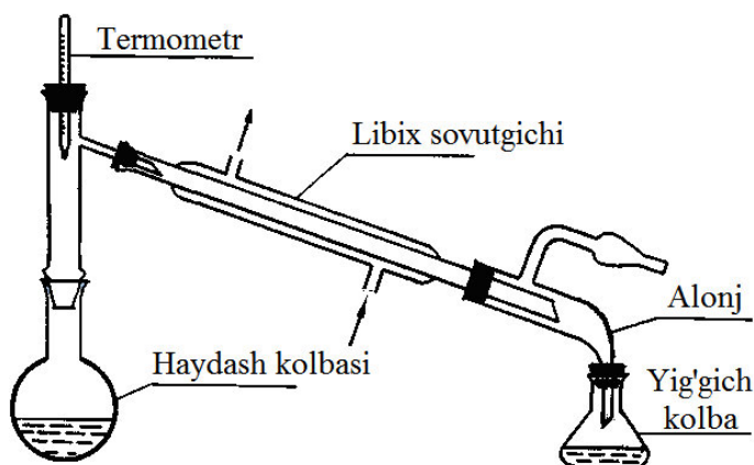
1-rasm. Oddiy haydash qurilmasi
