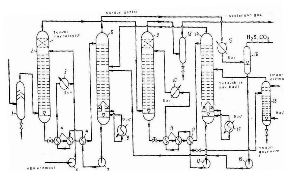
26-rasm. Gazlarni tozalash texnologiyasining sxemasi.
