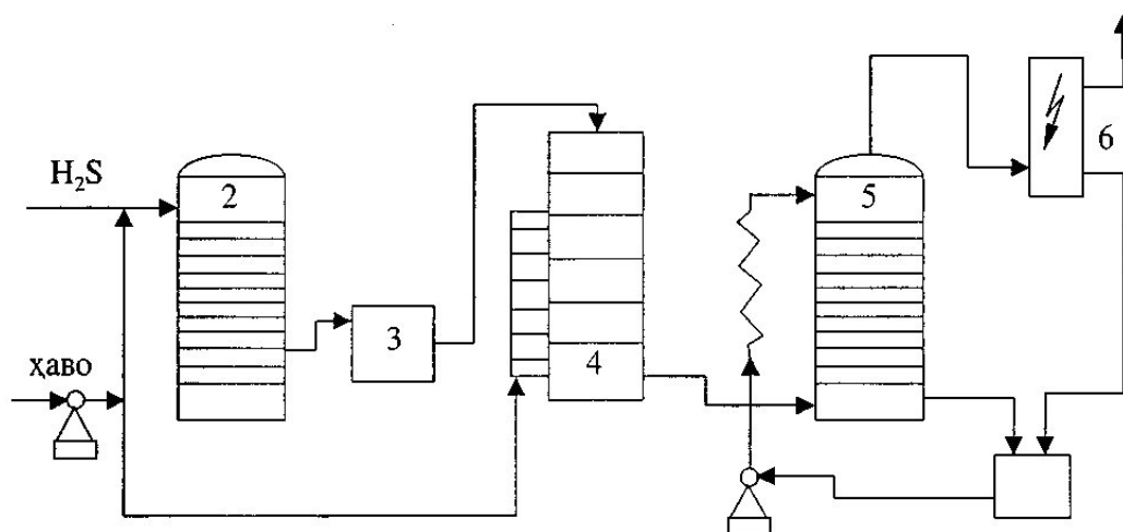
28-rasm. H_2SO_4 ni olish sxemasi.
