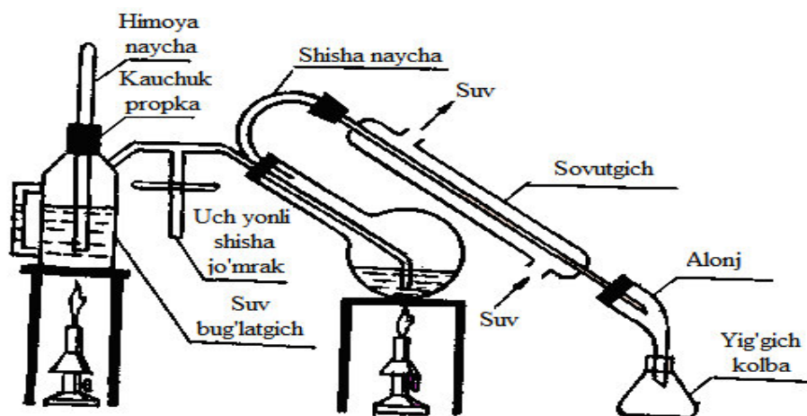
4-rasm. Suv bug'i yordamida haydash laboratoriya asbobi
