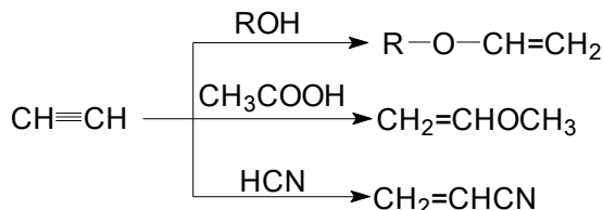
18-rasm. Asetilenni neft kimyosi sanoatida ishlatilishi.
