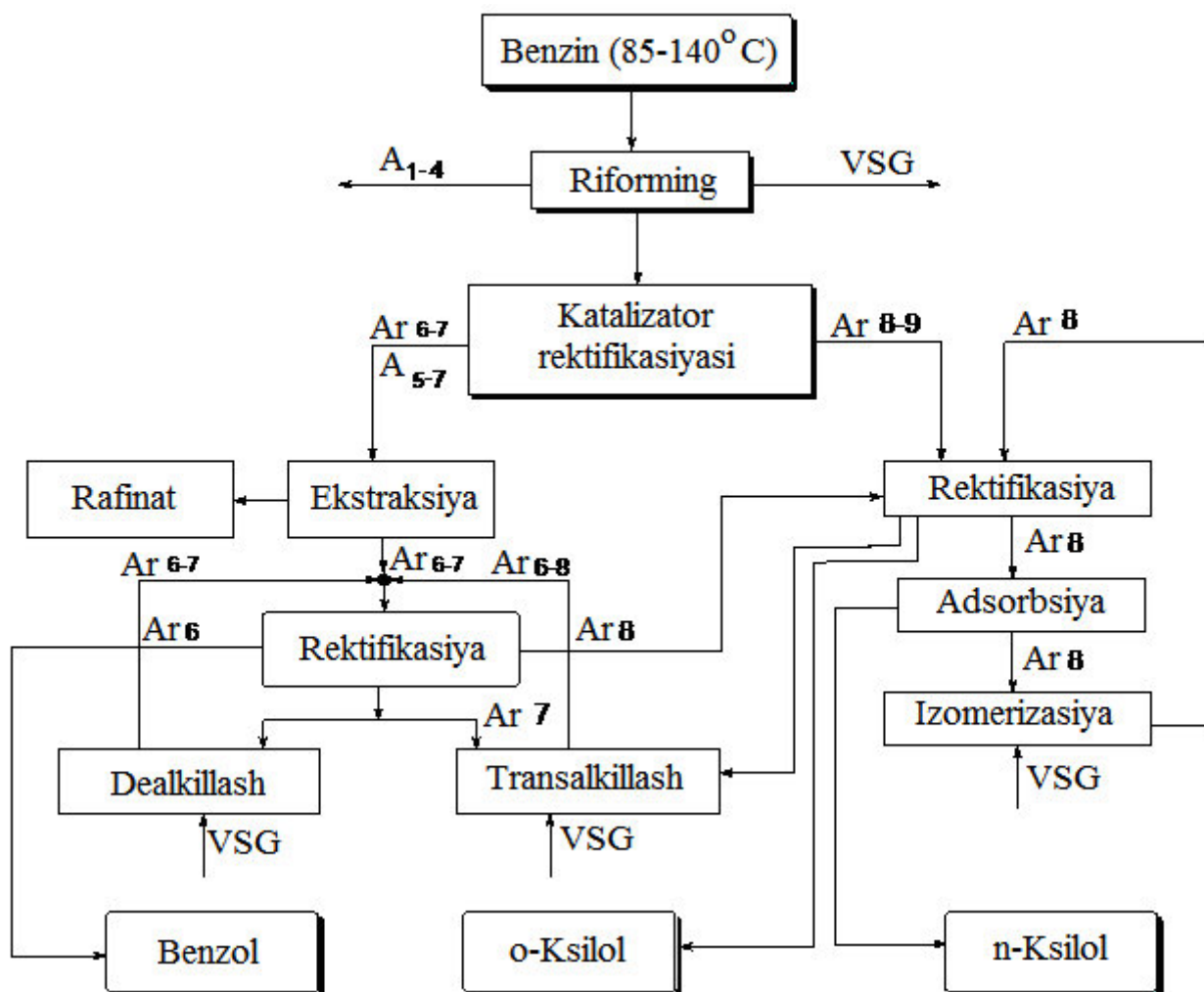
23-rasm. Arenlarni kompleks ishlab chiqarish sxemasi.
