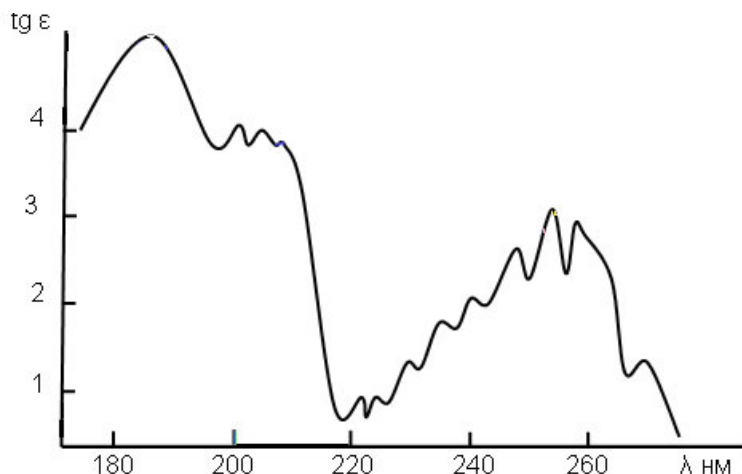
7-rasm. Neftdan olingan benzolning geptandagi UB spektri.
