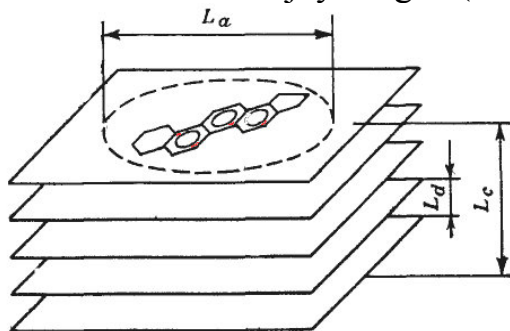
25-rasm. Asfaltenli moddalar bir bo'lagining tuzilishi
