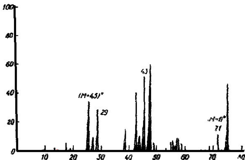
10-rasm. Moy aldegidning mass-spektri.
