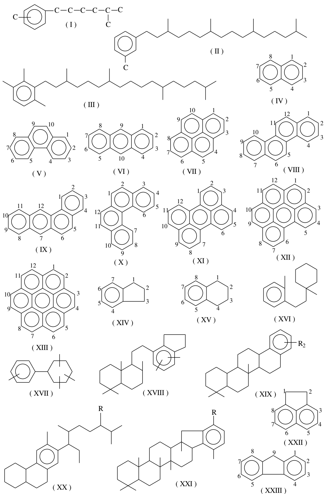
14-rasm. Neft tarkibidagi naften va aromatic uglevodorodlar.
