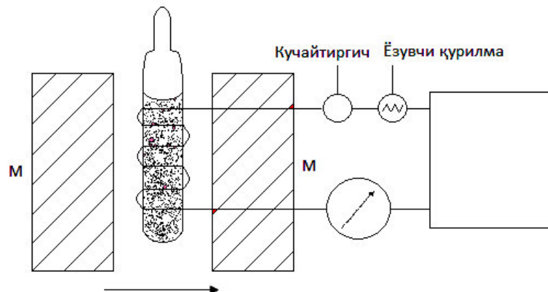
9-rasm. YaMR– spektrometrining umumiy ko'rinishi
