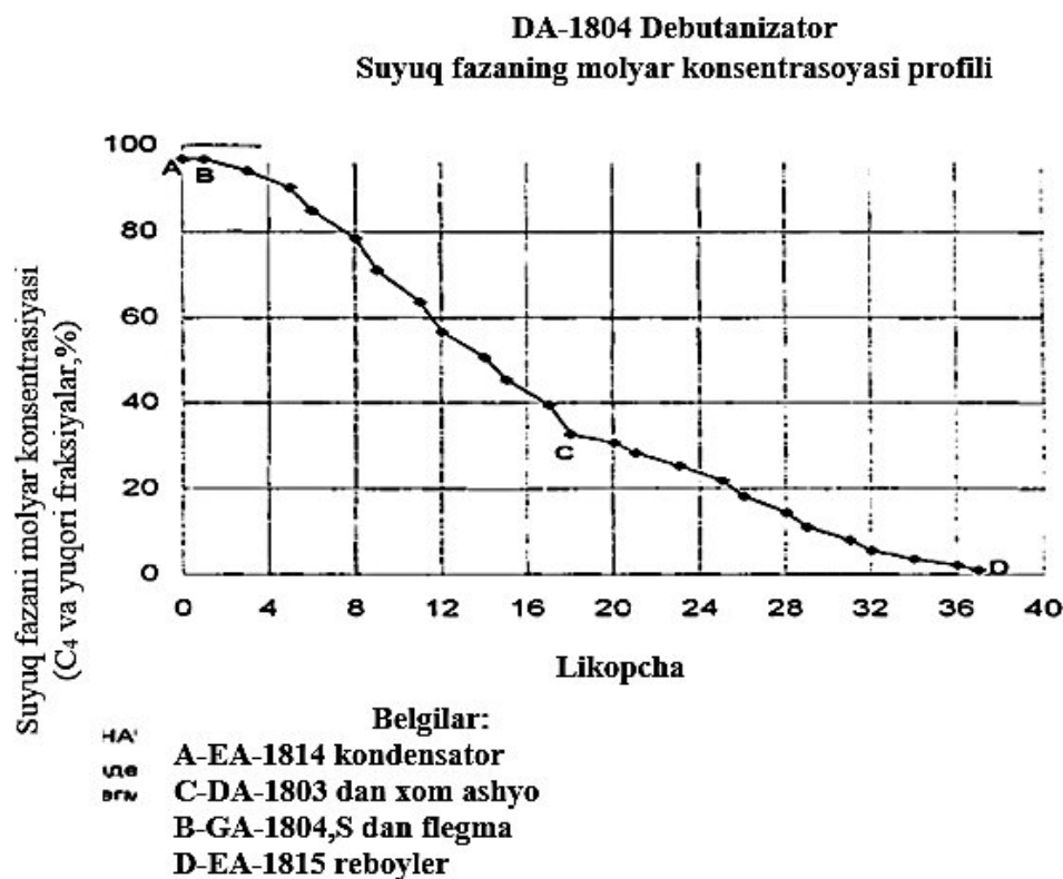
28-rasm. DA-1804 debutanizatorning suyuq fazasining molyar konsentratsiyasi profili.
