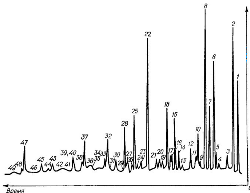
15-rasm. Neftning fraksiyasini 125 °C xromatogrammasi (skvalan–qo'zg'almas faza 50 °C)
