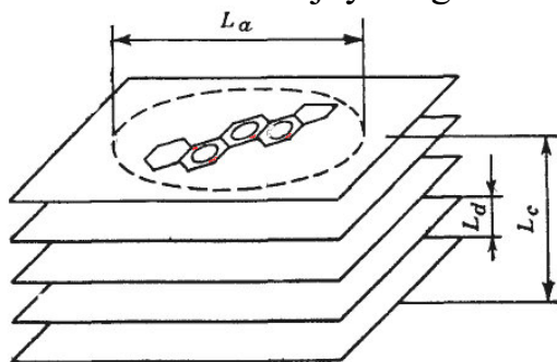
24-rasm. Asfaltenli moddalar bir bo'lagining tuzilishi
