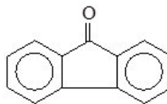
fluorennon
