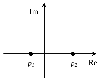
Рис.4.4. Корневой портрет объекта.
