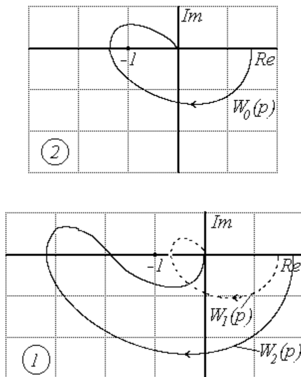
Рис. 8. Частотные характеристики, иллюстрирующие критерий Найквиста 1 - устойчивая система; 2 - неустойчивая система
