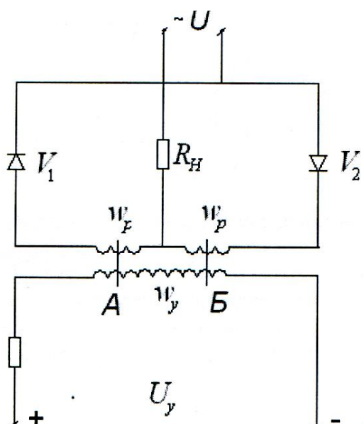
Рис.5.5. Магнитный усилитель.
