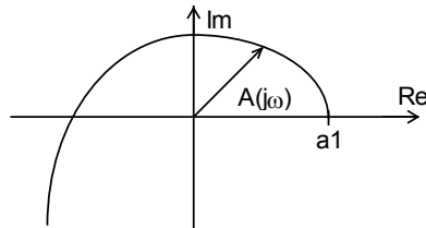
Рис. 1. Вид годографа Михайлова.
