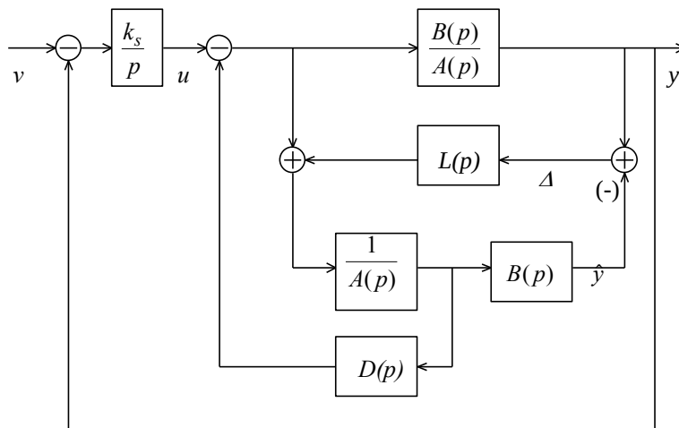
Рис. 5. Полная структурная схема системы, рассчитанной модальным методом
