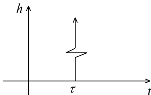
Рис. 1. Переходная характеристика звена
