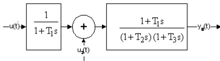
Рис. 8. Структура исходной системы.
