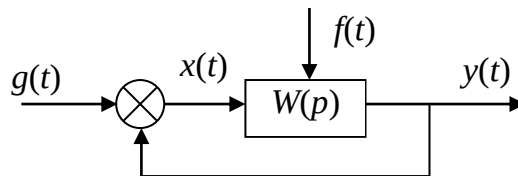
Рис. 4. Случайный задающий сигнал и случайная помеха в САУ
