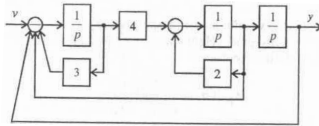
Рис.8.13. Структурная схема системы к задаче 10
