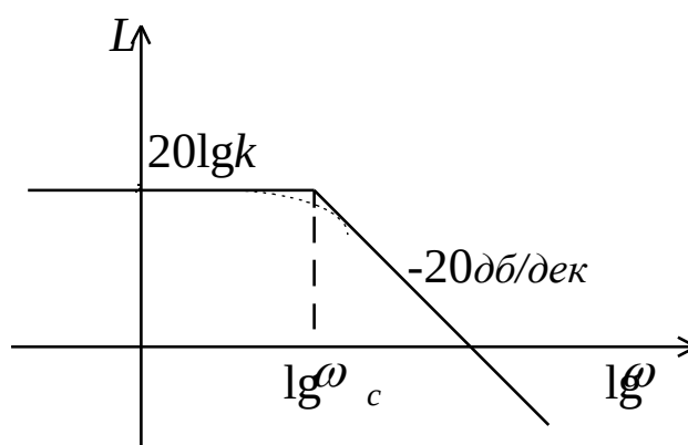
Рис. 10. ЛАЧХ апериодического звена
