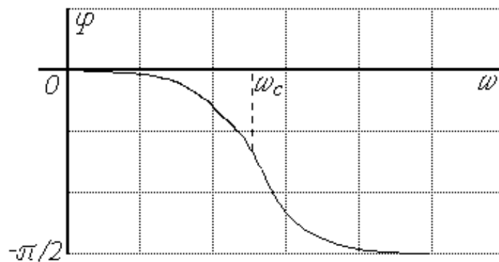
Рис. 8. ФЧХ аperiodического звена
