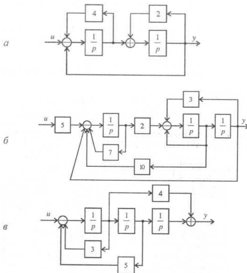
Рис.6.10. Структурная схема к задаче 5
