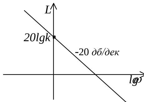
Рис. 9. ЛАЧХ интегрирующего звена
