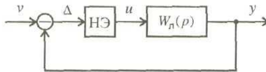
Рис. 1. Структурная схема комбинированной системы
