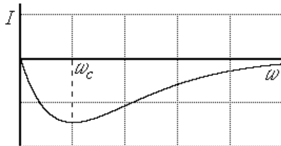
Рис. 6. МЧХ звена
