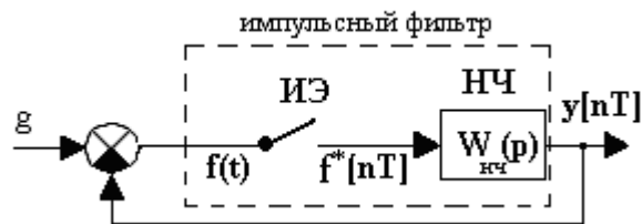
Рис. 1. Функциональная схема импульсной системы
