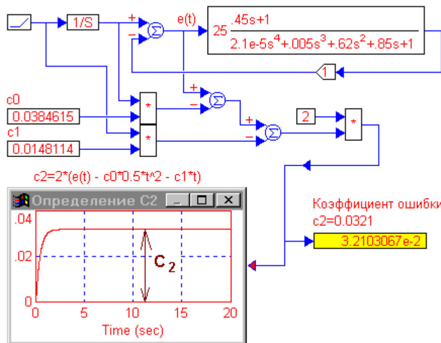
Рис.3. Схема для определения коэффициента ошибки c_2 САР по ускорению и осциллограмма с указанным значением коэффициента. Параболическое воздействие формирует интегратор, интегрирующий линейно растущий сигнал
