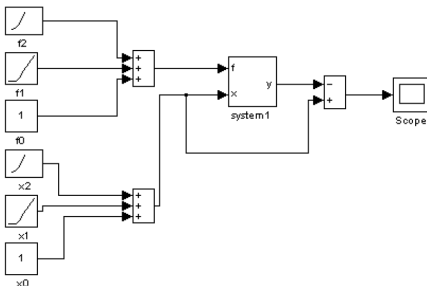
Рис.8.2. Схема эксперимента.
