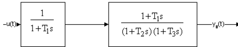
Рис. 9. Пример не полностью наблюдаемой системы
