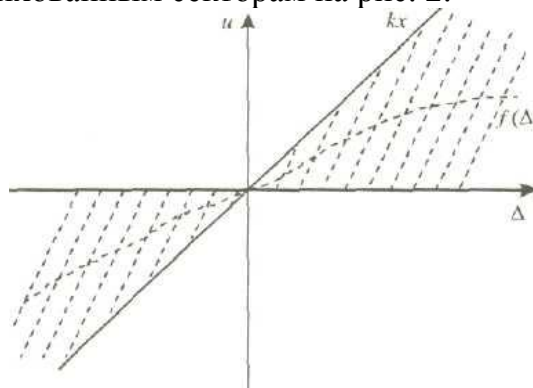
Рис. 2. Пример ограничений на нелинейность
