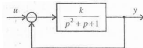
Рис.8.8. Структурная схема системы
