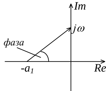
Рис. 2. Элементарный вектор, соответствующий устойчивому вещественному корню
