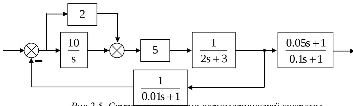
Рис.2.5. Структурная схема автоматической системы.
