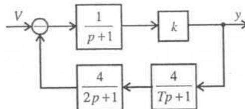
Рис.8.15. Структурная схема системы к задаче 14
