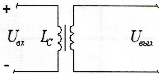
Рис.5.6. Стабилизирующий трансформатор.
