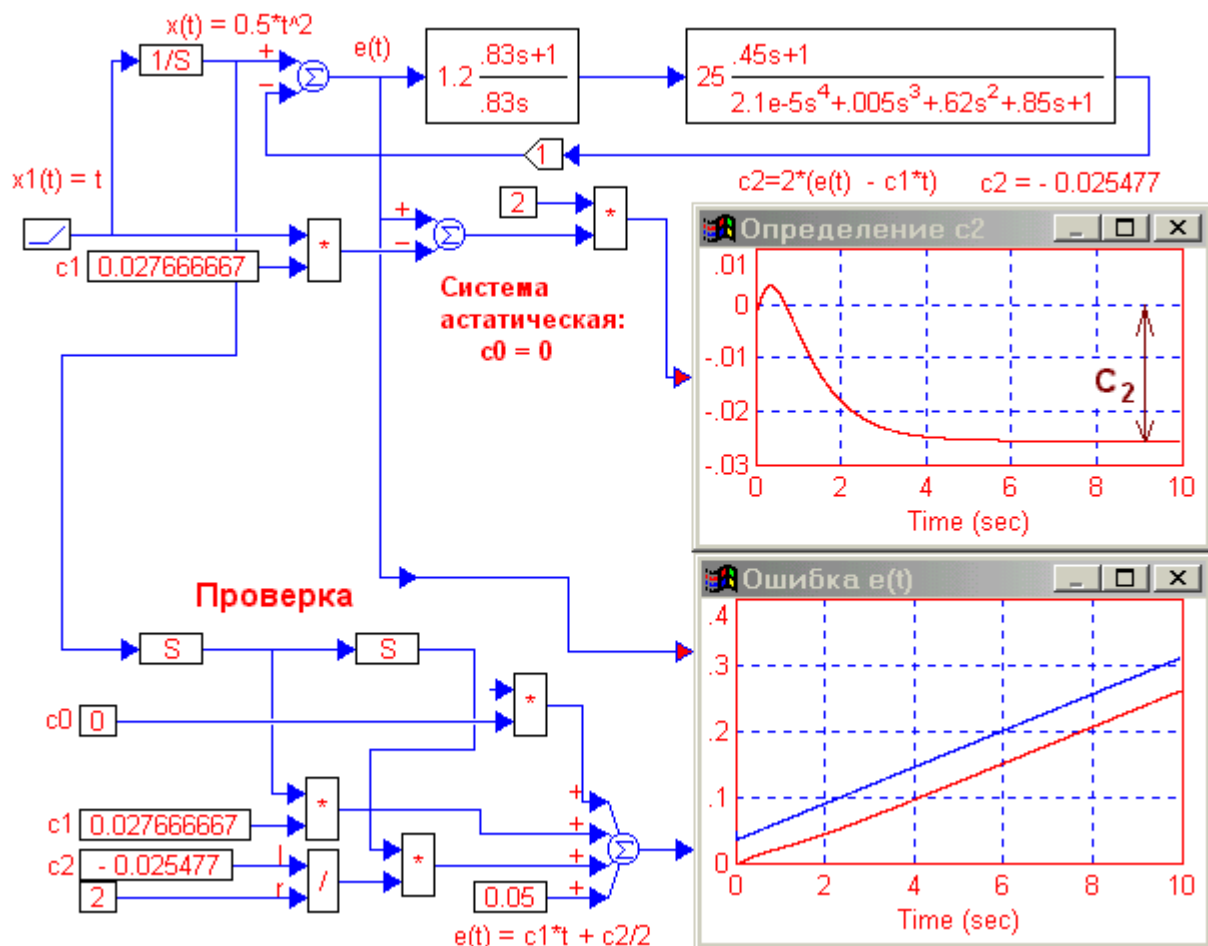
Рис.5. Схемы для определения коэффициента ошибки по ускорению c_2 астатической САР и проверки правильности определения коэффициентов ошибок. Синий график на нижней осциллограмме приподнят на величину 0,05 для удобства сравнения величин ошибок. Как видно, по окончании переходного процесса, примерно через 3 сек, значение ошибки e(t) , определенное с помощью коэффициентов ошибок растет линейно, как и положено при параболическом воздействии на систему первого порядка астатизма, и совпадает с ошибкой модели. Значение коэффициента c_2 для получения более высокой точности целесообразно определять в этом примере при длительности развертки осциллографа, равной 100сек
