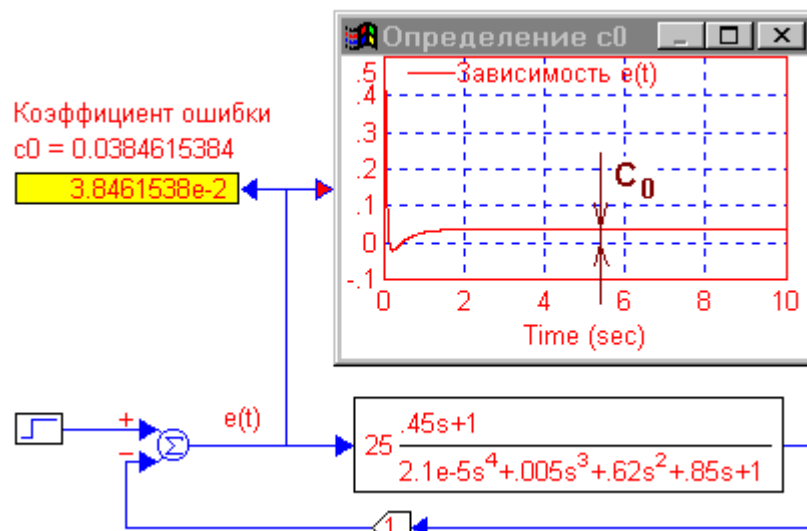
Рис.1. Определение коэффициента ошибки c_0 для статической системы. Значение коэффициента равно установившемуся значению ошибки регулирования
