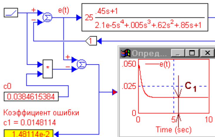
Рис.2. Определение коэффициента ошибки по скорости c_1 . Значение ошибки, численно равное коэффициенту c_1 , следует определять по окончании переходного процесса
