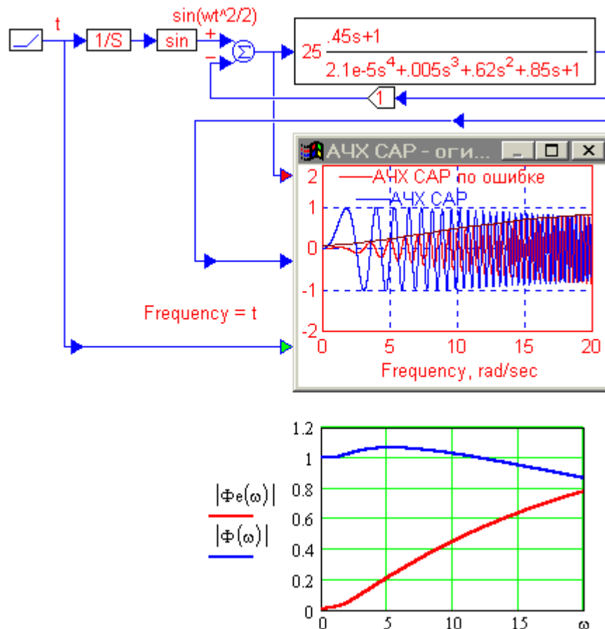
Рис.6. Использование ЛЧМ сигнала для построения АЧХ САР. Огибающие частотно-модулированного сигнала и представляют собой амплитудно-частотные характеристики (АЧХ). Внизу показаны для сравнения те же характеристики, построенные в программе Mathcad 2000
