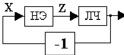
Рис. 10.1. Функциональная схема нелинейной системы:
