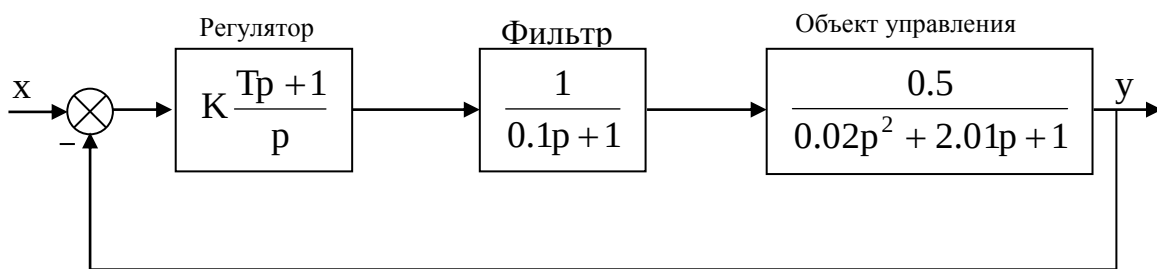
Рис.6.1. Структурная схема исследуемой системы.
