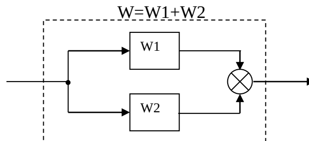
Рис.2.2. Параллельное соединение объектов.
