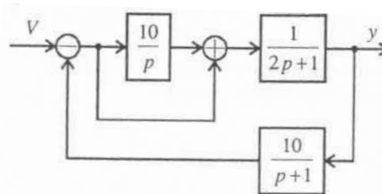
Рис.8.14. Структурная схема системы к задаче 13
