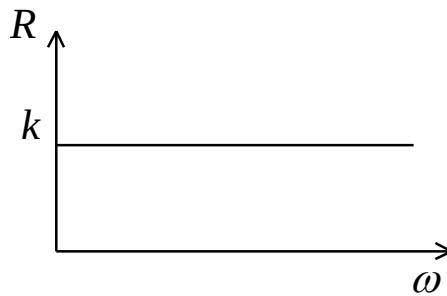
Рис. 2. ВЧХ пропорционального звена
