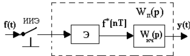
Рис.3. Расчетная функциональная схема разомкнутой импульсной системы
