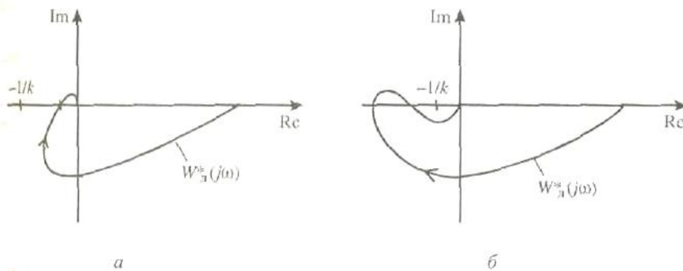
Рис. 3. Пример выполнения (а) и невыполнения (б) условий абсолютной устойчивости
