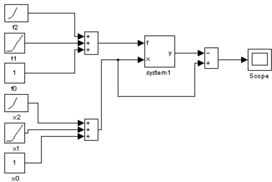
Рис.8.2. Схема эксперимента.
