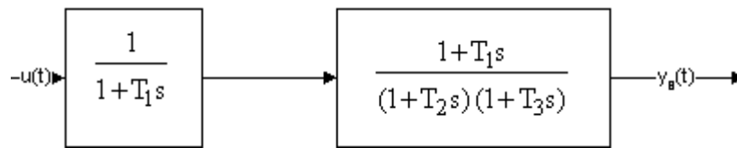
Рис. 9. Пример не полностью наблюдаемой системы
