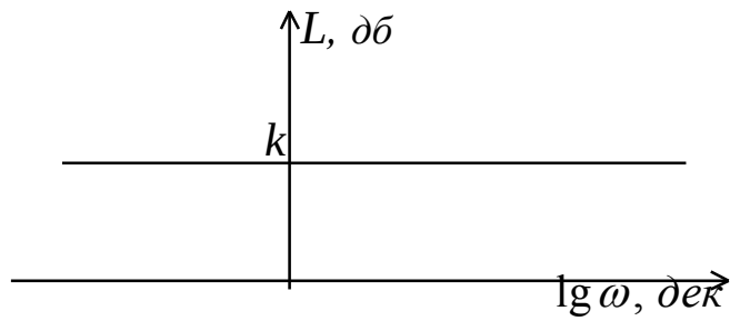
Рис. 4. ЛАЧХ пропорционального звена
