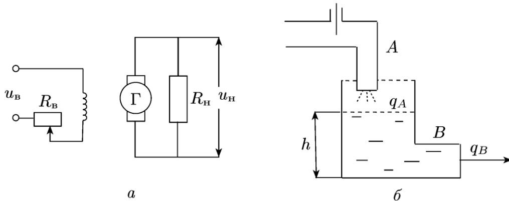
Рис. 5. Объекты управления: а — генератор напряжения; б - резервуар с жидкостью
