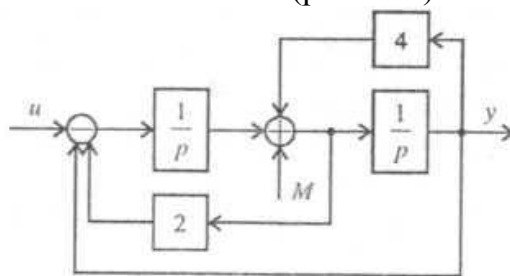
Рис.6.11. Структурные схемы к задаче 4
