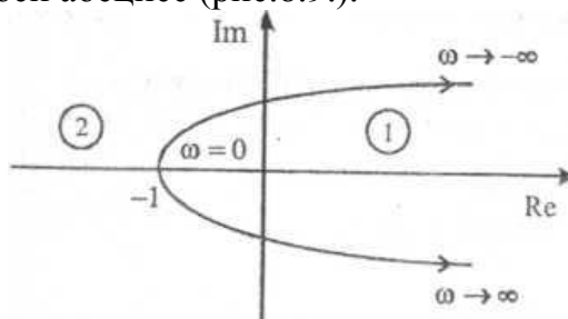
Рис.8.9. Кривая D -разбиения для исследуемой системы
