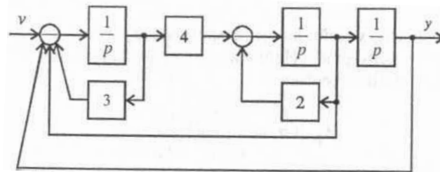
Рис.8.13. Структурная схема системы к задаче 10
