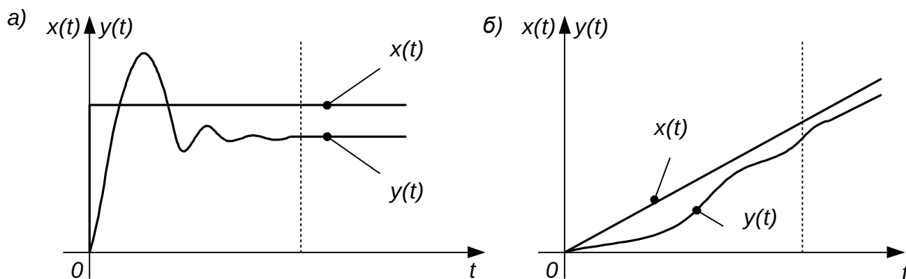
Рис. 3. Переходные и установившиеся режимы при типовых воздействиях
