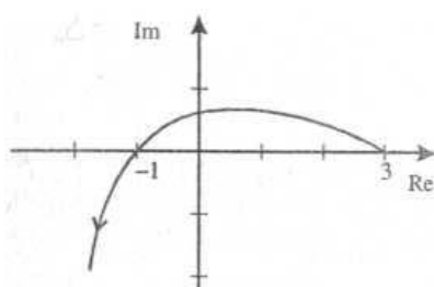
Рис. 8.2. Годограф Михайлова для примера 5
