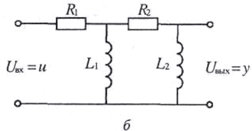
Рис. 4.7. Схемы к задаче 2.
