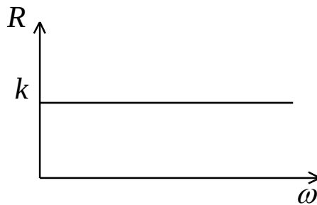
Рис. 2. ВЧХ пропорционального звена
