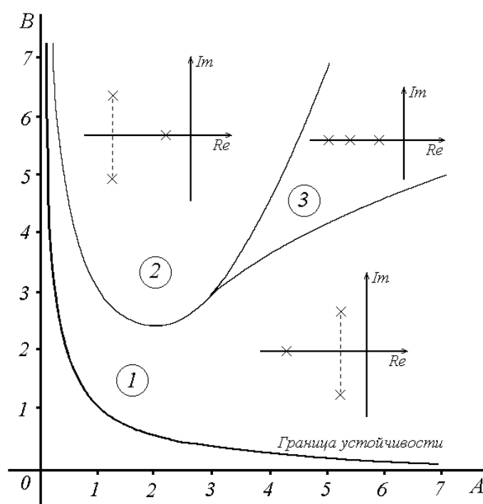
Рис. 4. Диаграмма Вышнеградского
