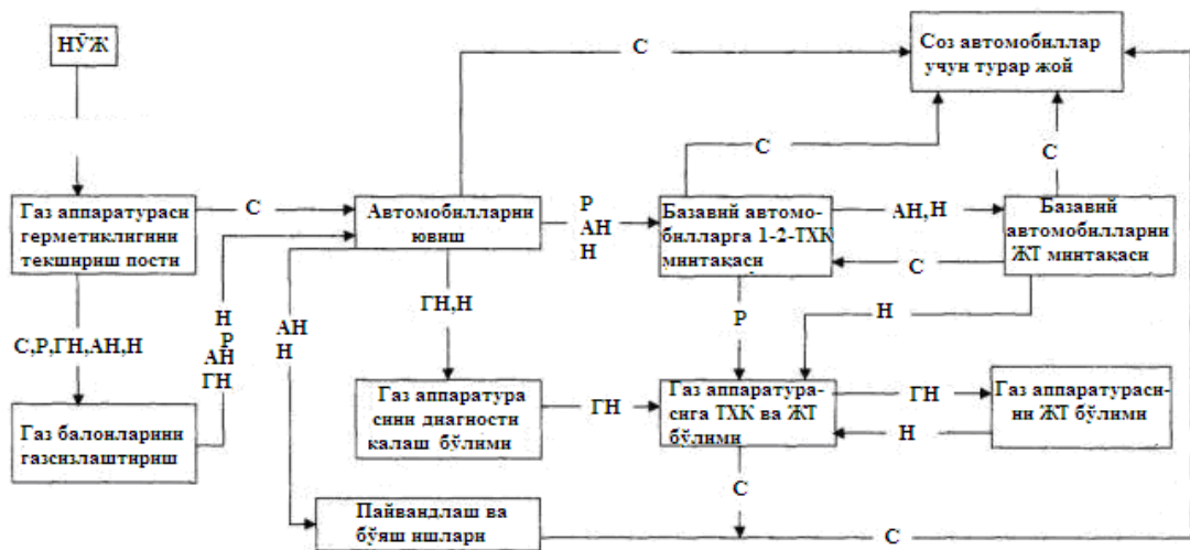
2.1-rasm. Gaz apparaturali avtomobillar TXK va JTni texnologik shakli:
