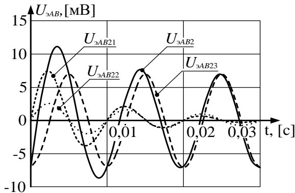
Рис. 6. Графики переходных напряжений в одной измерительной обмотке ИП с заданной разностью пульсирующих постоянных токов
