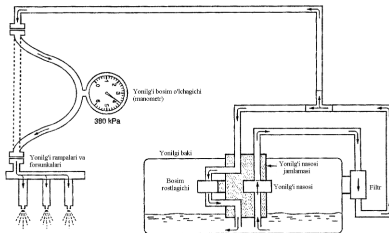
3.1-rasm. Yonilgi tizimidagi bosimni tekshirish sxemasi.
