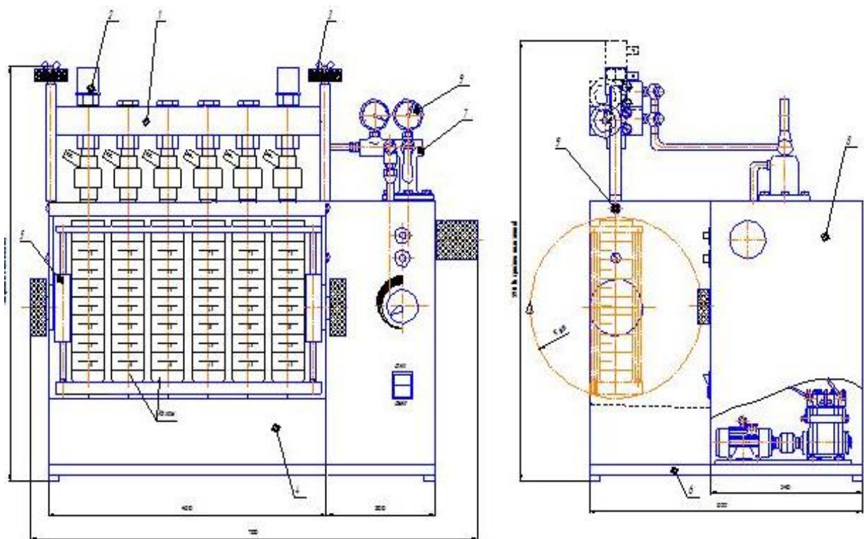
1-yuqori reyka; 2-trubka; 3-barashkali (quloqli) qotirgich; 4- menzurka; 5-pastki reyka; 6-fiksator; 7-reduktor; 8-manometr; 9-manometr.
