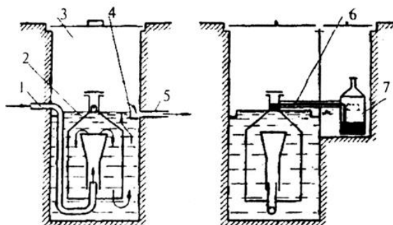
3.3-rasm. Moy-benzin to'plagich: a-qurilmani ishlash jarayoni shakli; b-moy va benzinni ajratish jarayoni shakli; 1-to'plagichga suv keladigan quvur; 2-ioy va benzin aralashmasini ajratish qalpog'i; 3-moy-benzin tutgich qudug'i; 4-suv sathini cheklovchi nov; 5-tozalangan suv chiqib ketadigan quvur; 6-moy-benzin aralashmasini o'tkazuvchi naycha; moy-benzin aralashmasini yig'adigan idish.
