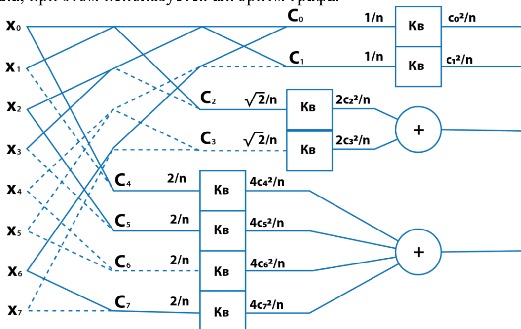
Рис. 2. Граф октавного алгоритма расчета спектральной энергии
