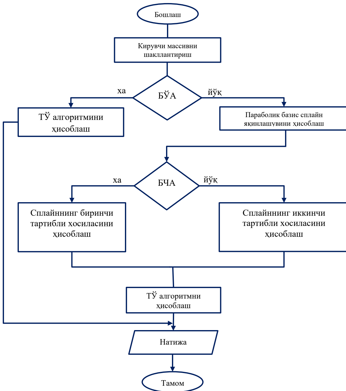
1-расм. Бўлак-ўзгармас(БЎ), бўлак-чизиқли(БЧ) ва бўлак-квадратик(БК) базисларда коэффицентларни ҳисоблаш алгоритми
