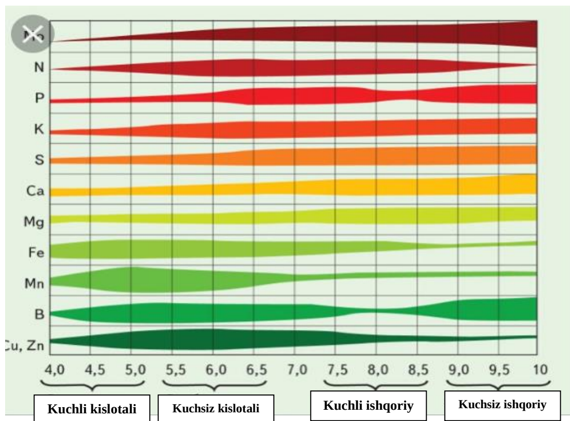
7.1-rasm. Tuproq muhitini aniqlash grafigi
