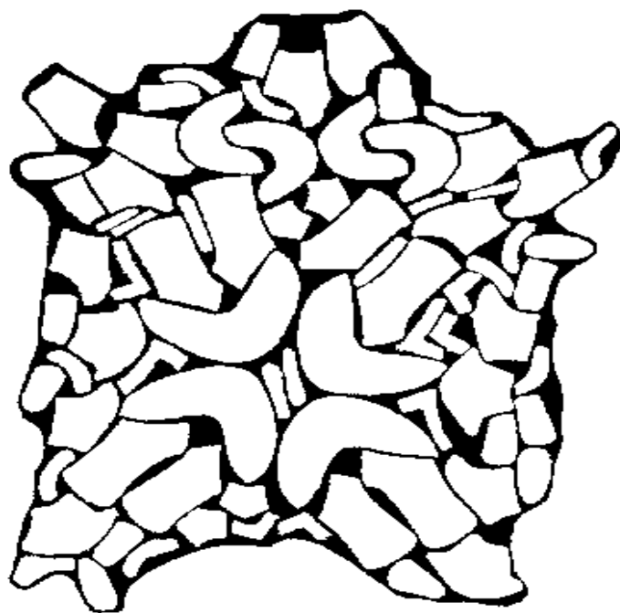
3.34-rasm. Poshnasi qoplangan modali ayallar tuflisi qismlarini, bolalar batinkasi qismlari bilan birgalikda shevro teridan bichilgan tasviri.
