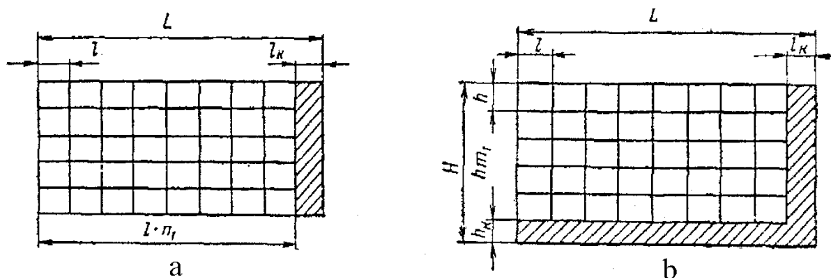
3.7-rasm. To'g'riuchakli andozalar va bichiladigan materiallarni qaytarilmaydigan razmerlari hisobiga paydo bo'ladigan chetki chiqindilar.
