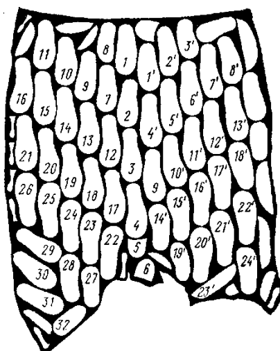
3.58-rasm. Cheprakni to'g'ri chiziqli olg'a siljish usulida qismlarni tutamlaridan birga qo'shib qirqish tasviri.
