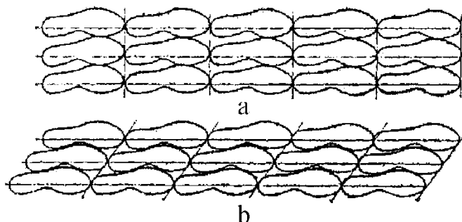
3.5-rasm. Tag charm andozalarini to'g'ri chiziqli olg'a siljib borish holatida joylashtirish
