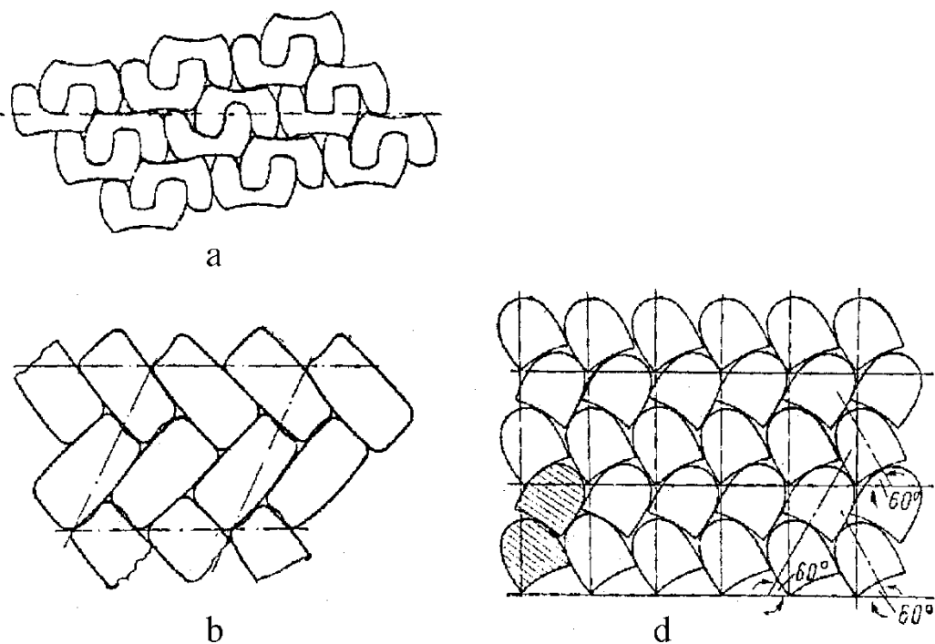
3.6-rasm. Boshliq (a), dastak (b), poshna (d) andozalarini belgilangan burchakka qayrib joylashtirish tasviri.
