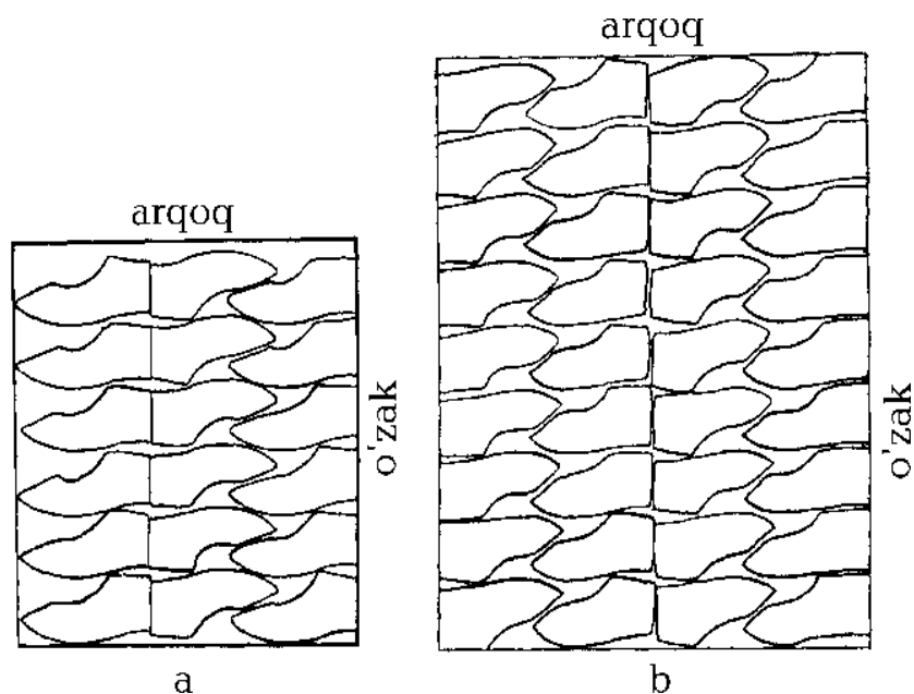
3.40-rasm. To'qima matolarning ko'pqavatli to'shamasida erkaklar yarim batinka qismlarini birgalikda qo'shib bichish tasviri.
