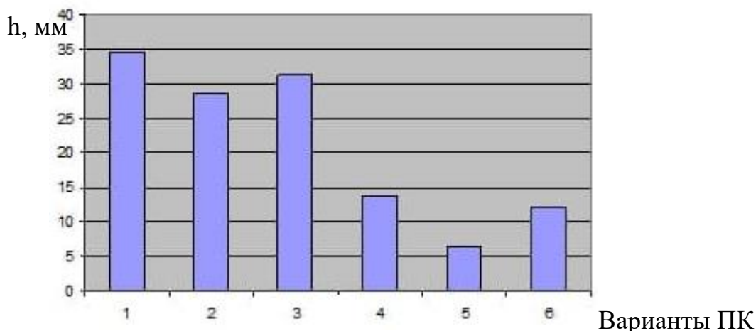
Рис. 2. Зависимость значения высоты прогиба ( h ) формозадающей поверхности от состава применяемой полимерной композиции
