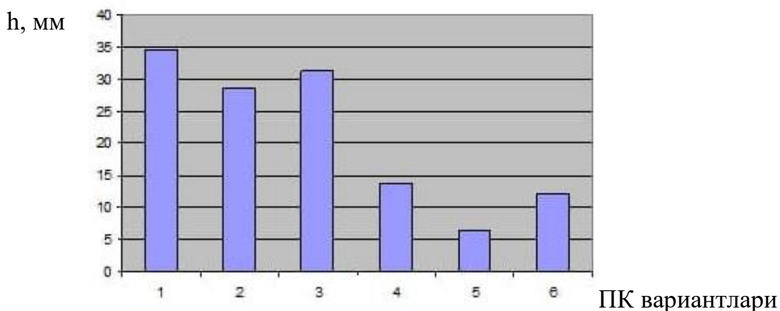
2-расм. Шакл барқарорлигини коллаген полимер композициясининг турли таркибига боғлиқлиги
