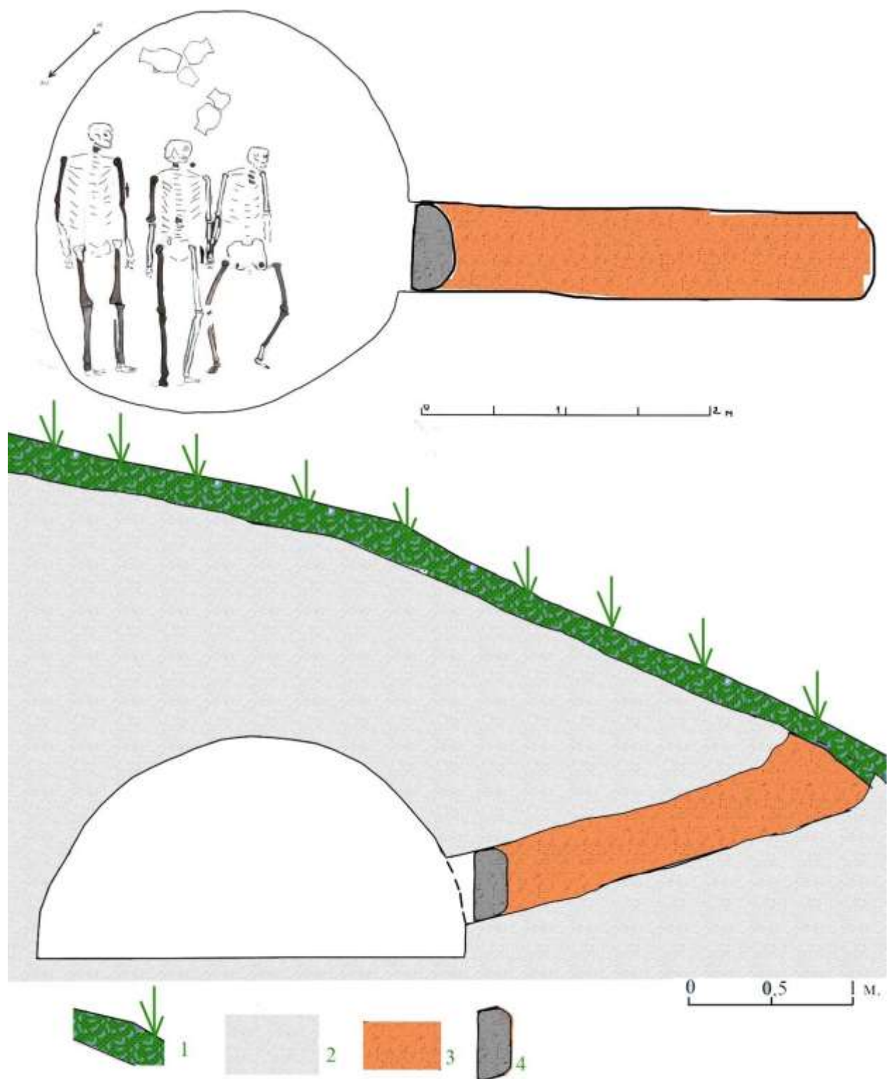
23 -расм. плани ва кесмаси
