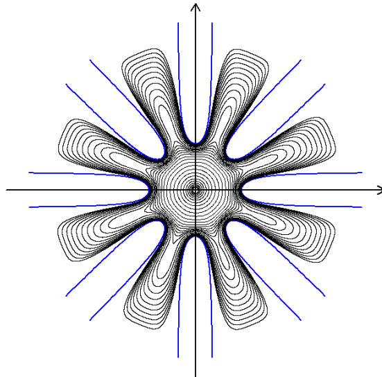
1-расм. n = 2 учун (3) системанинг траекторияларидан бири ва унинг \omega -лимит тўплами.
