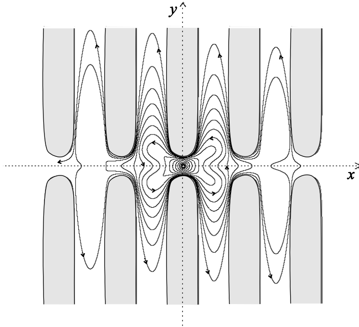
2-расм. Чексиз кўп боғлиқлик компоненталарига эга аналитик система.
