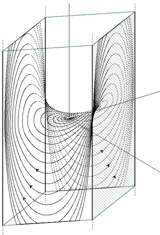
3-расм. (5) системанинг фазавий портрети
