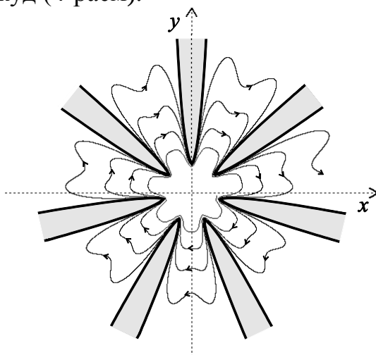
4-расм. 7 та боғлиқлик компонентасига эга бўлган полиномиал система
