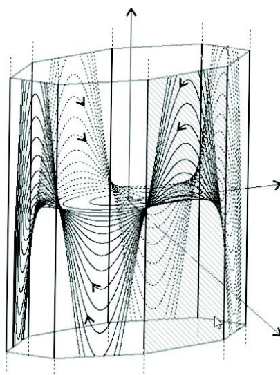
5-расм. Лимит тўплами саккизта тўғри чизикдан иборат бўлган уч ўлчовли полиномиал система
