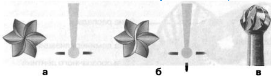
Рис. 104. Варианты шаровидных твердосплавных боров компании NTI: а – бор серии H1 с неактивной вершушкой рабочей части (все грани заканчиваются в «мертвой точке» на вершине бора, бор эффективно работает только в боковых направлениях); б – бор серии H1S с активной вершушкой рабочей части (имеет S-образную перекрывающую грань на вершине, эффективно работает по всем направлениям); в – бор H1SX с активной вершушкой рабочей части и дополнительной перекрестной насечкой на режущих гранях (имеет повышенную агрессивность).
