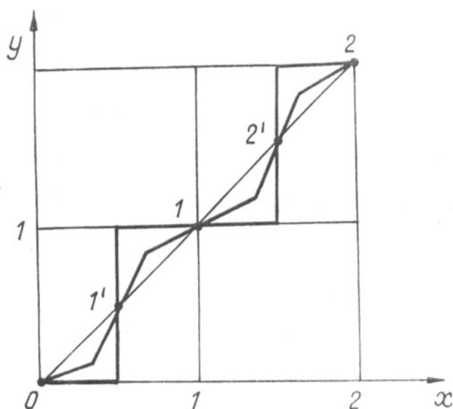
Расм. Кўпҳолатли элементларни ўтиш характиристикаси.
