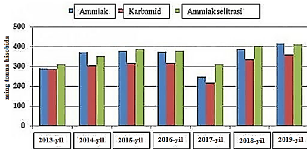
7-rasm. 2013-2018-yillarda Respublika kimyo zavodlarida ammiak, karbamid va ammiakli selitra ishlab chiqarish dinamikasi
