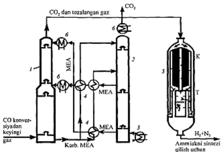
4-rasm. CO 2 dan (MEA-tozalash) va CO dan (metanlash) tozalashning texnologik sxemasi
