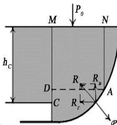
Расм 12. – Эгри чизиqli юзага таъсир
