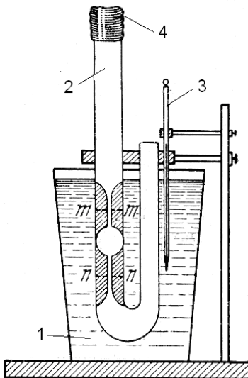
1.2-rasm. Kapillyar viskozimetrning ish jarayoni
