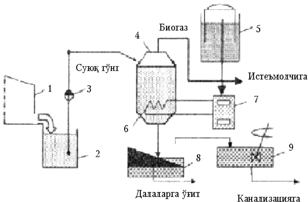
1-расм. Гўнг шарбатини биогаз ускурмасида қайта ишлашни технологик чизмаси
