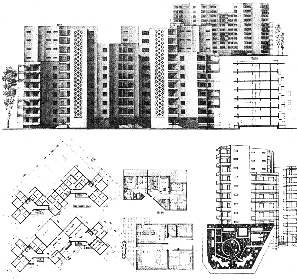
42-расм. Кўп қаватли икки секцияла турар жой биноси.
