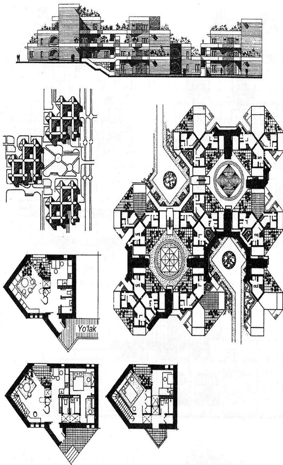
38-расм. 2-4 қаватли галереяли уйлар комплекси
