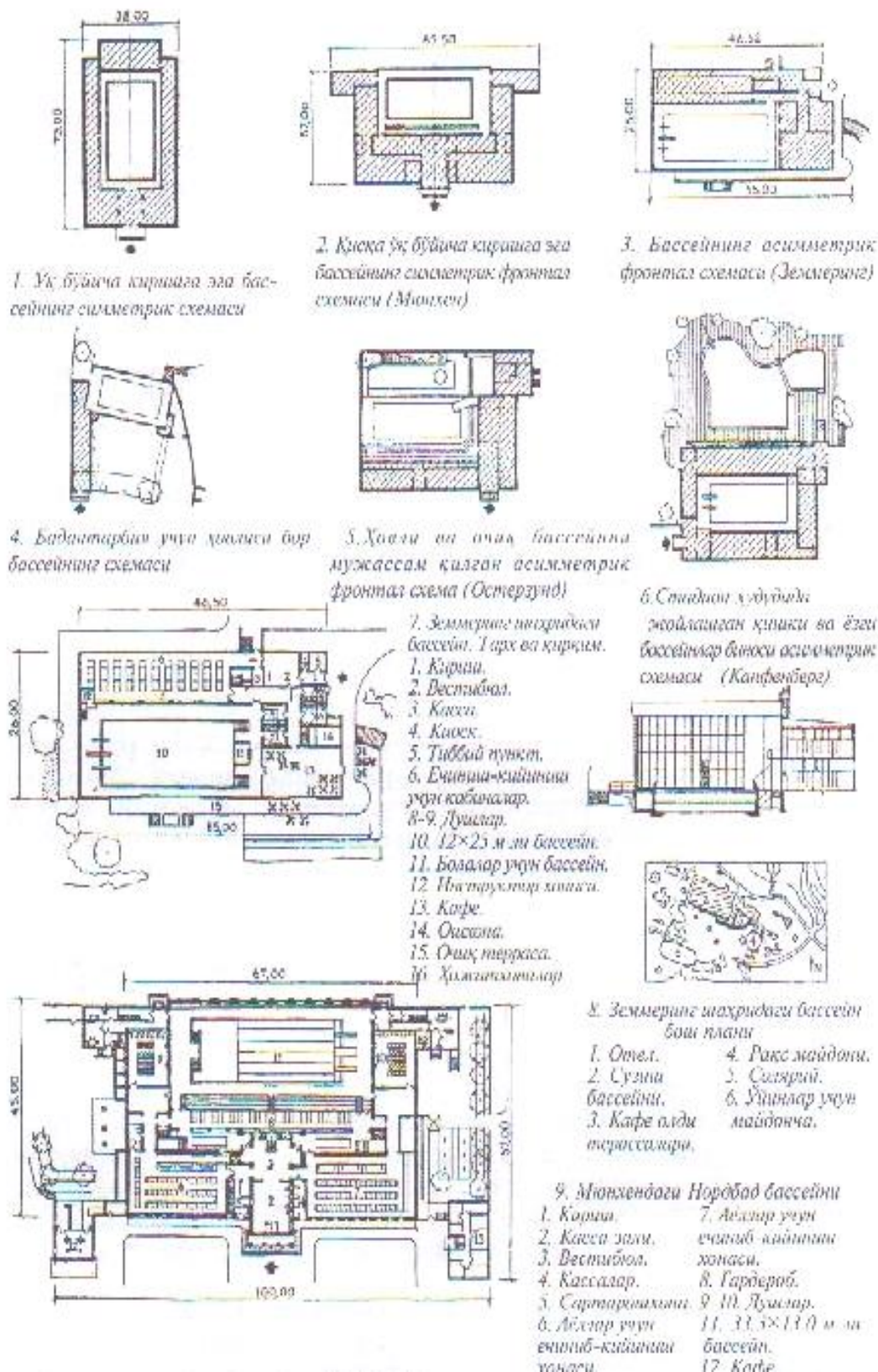
93-расм. Спорт бассейнларининг тархлари.
