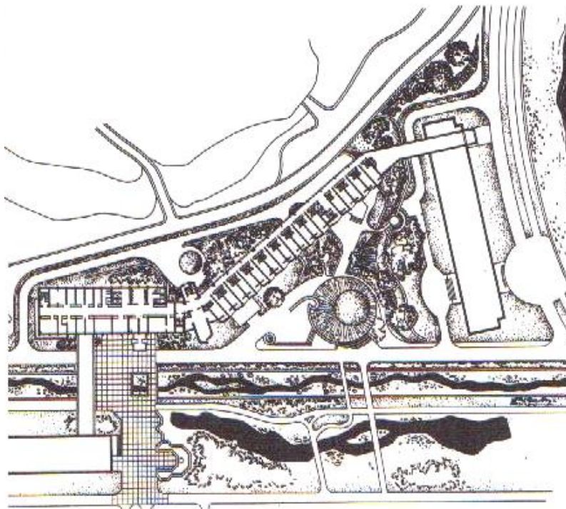
111-расм. Қримда қурилган санатория комплексининг макети ва бош режаси
