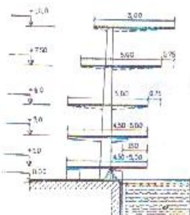
3. Сувага 1 ва 3 м ли трамздан ва 5, 7, 5 м ли баландликдан сакрани мосламаси
