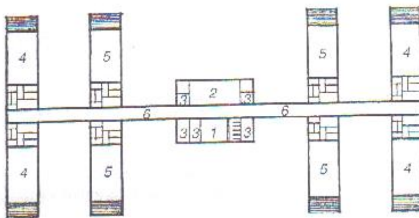
51-расм. 280 ўринли болалар муассасаси асосий хоналар гуруҳининг ўзаро боғланиш схемаси: 1 — вестибюль ; 2 - ошхона ; 3 - маъмурий-хўжалик хоналари ; 4 — боғчанинг ячейкалари ; 5 - яслининг ячейкалари ; 6 - коридор-галерея .
