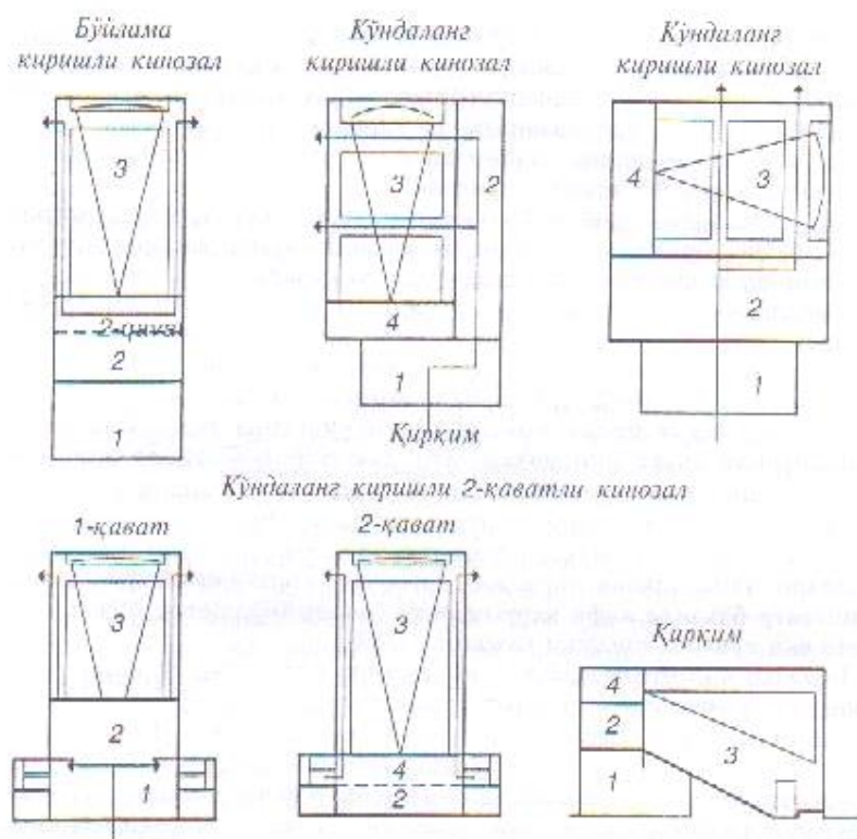
66-расм. Бир залли кинотеатрларнинг композициявий схемалари: 1-вестибюль; 2-фойе; 3-томоша зали; 4-кинопроекция хонаси
