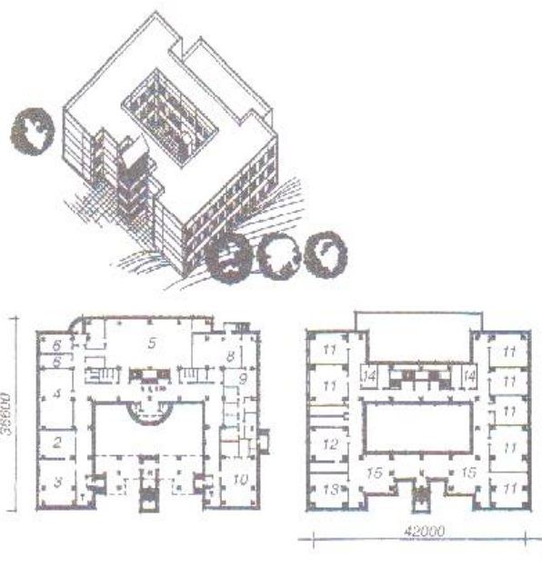
54-расм. 264 ўқувчига мўлжалланган умумтаълим мактаби. Умумий кўриниши ва тарҳи
