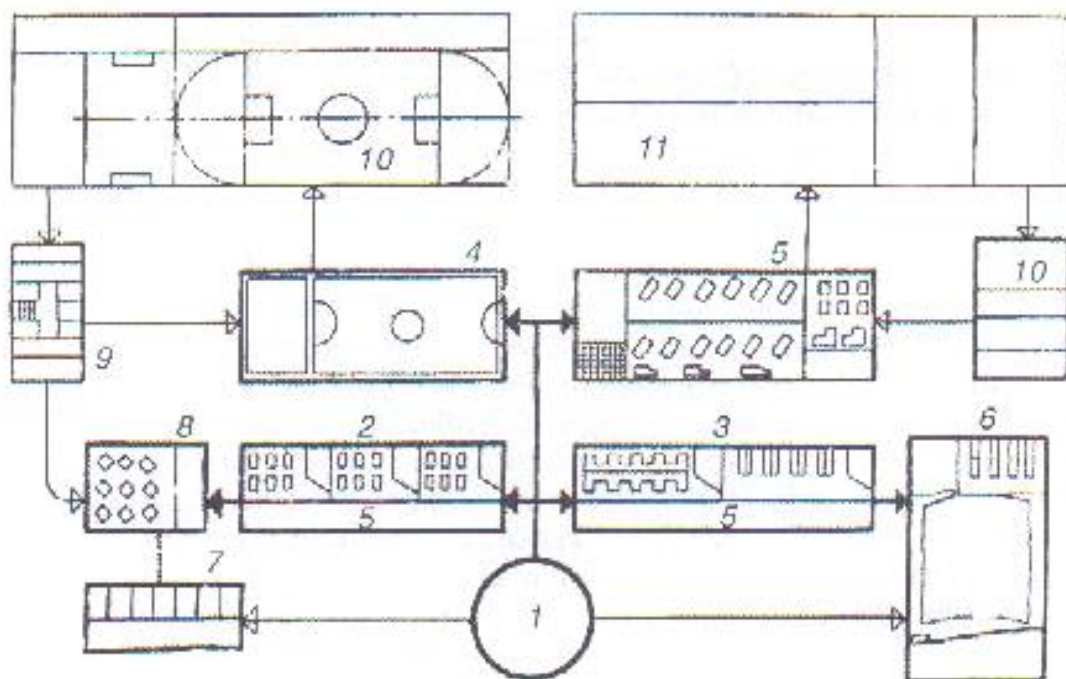
63-расм. Коллежлардаги хоналар гуруҳларининг ўзаро боғланиши: 1-бош кириш жойи ва вестибюль; 2-ўқув хоналари; 3-аудитория ва лабораториялар; 4-ўқув спорт хоналари; 5-рекреациялар; 6-кутубхона ва мажлислар зали; 7-маъмурий хоналари; 8-ошхона; 9-хўжалик хоналари; 10-ҳовлидаги спорт майдончалари; 11-ҳовли майдонидаги ўқув полигони
