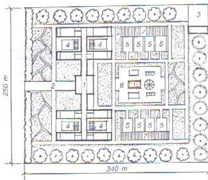
52-расм. 280 ўринли болалар муассасаси майдонини ташкил қилиш схемаси: - боғча-ясли биноси ; 2 - кириш хиёбони ; 3 - хўжалик ҳовлиси ; 4 — ясли гуруҳи болалари учун майдон ; 5 — катта болалар учун майдон ; 6 — ўйин учун майдон ; 7 - айвонлар .
