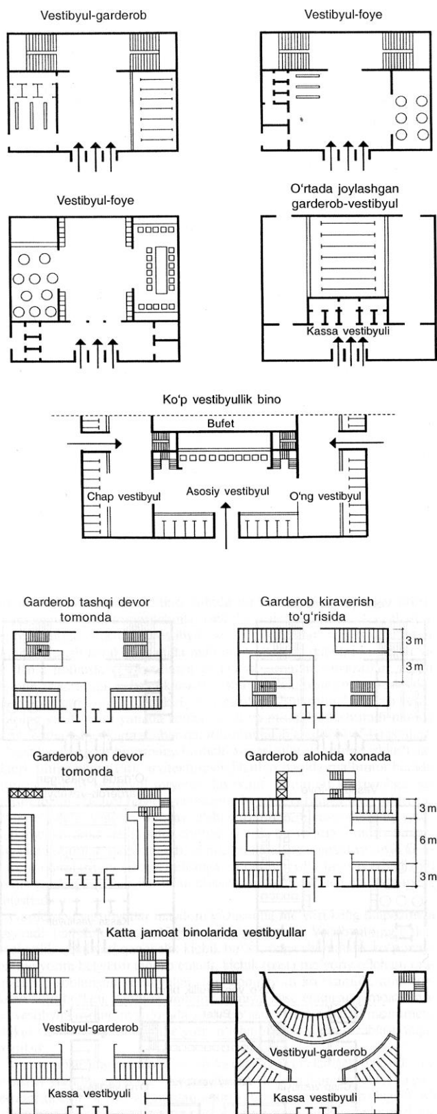
47-расм. Вестибюлларнинг турлари.
