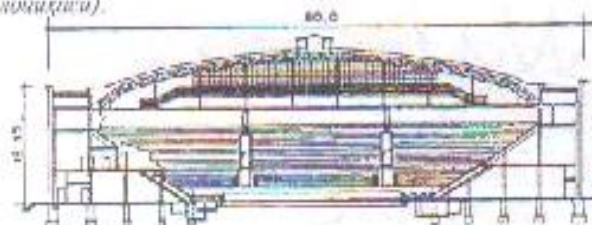
7. Москвадаги спорт саройи биносининг қирқими. ом ёнмаси металл фермалардан иборат. Трибуналар — бир ярусли
