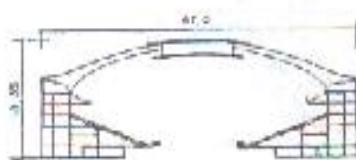
9. Дортмундаги спортзал биносининг қирқими. Том ёнмаси металл фермалардан иборат. Трибуналар — икки ярусли
