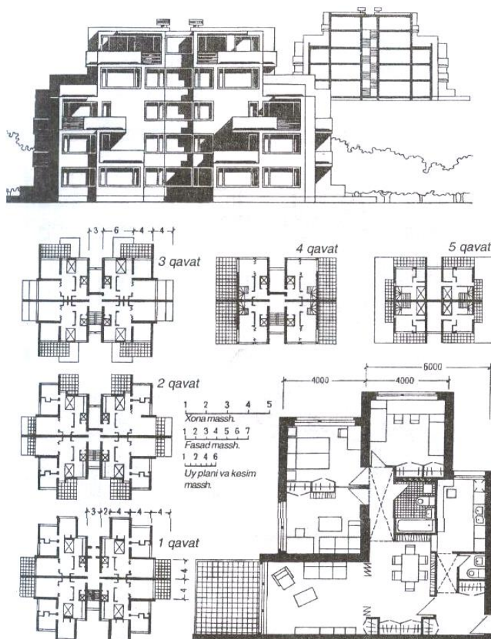
37-расм. 16 хонадонли ҳар тўрт томонига қисқариб борадиган ва ҳар бир хонадон террасага эга бўлган 5 қаватли бир секцияли турар жой биноси.
