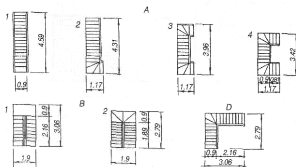
31-расм. Хона ичидаги зинапоя лойиҳасининг схемаси: А - бир тарафлама; 1 –тўғри; 2, 3, 4 - икки ва уч тарафлама; Б -икки тарафлама зинапоя; 1,2- зинапоя майдони билан; Д – бурчакли зинапоя.
