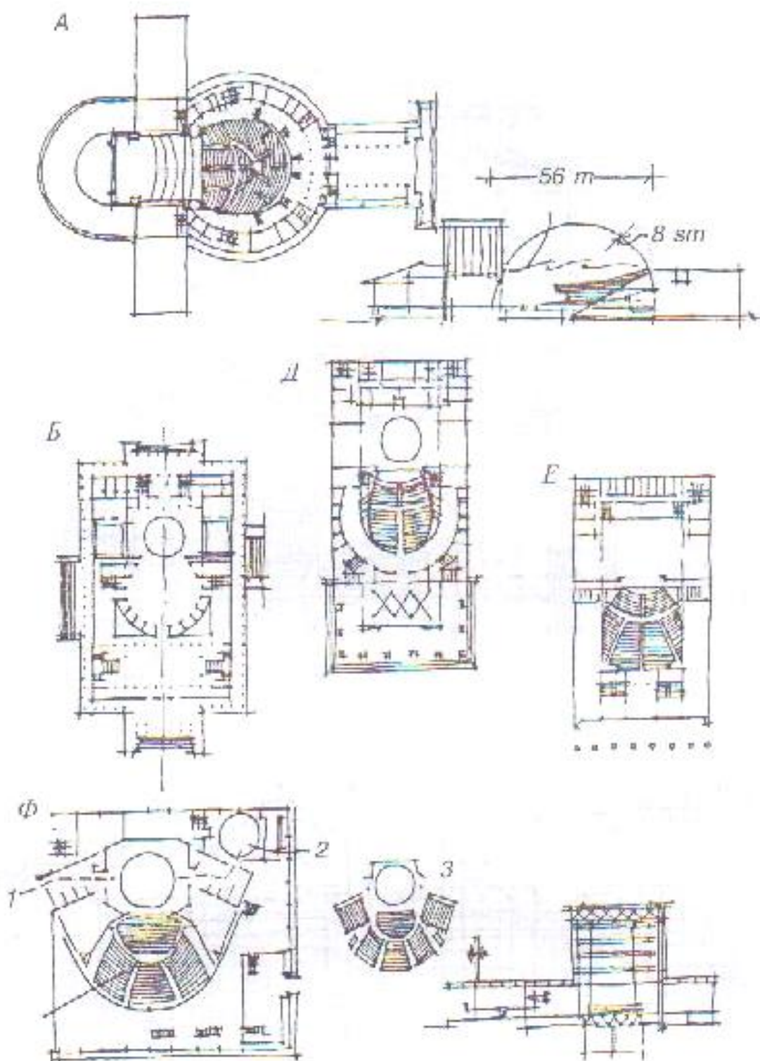
70-расм. Театрларнинг меъморий-режавий ечимларига доир намуналар:
