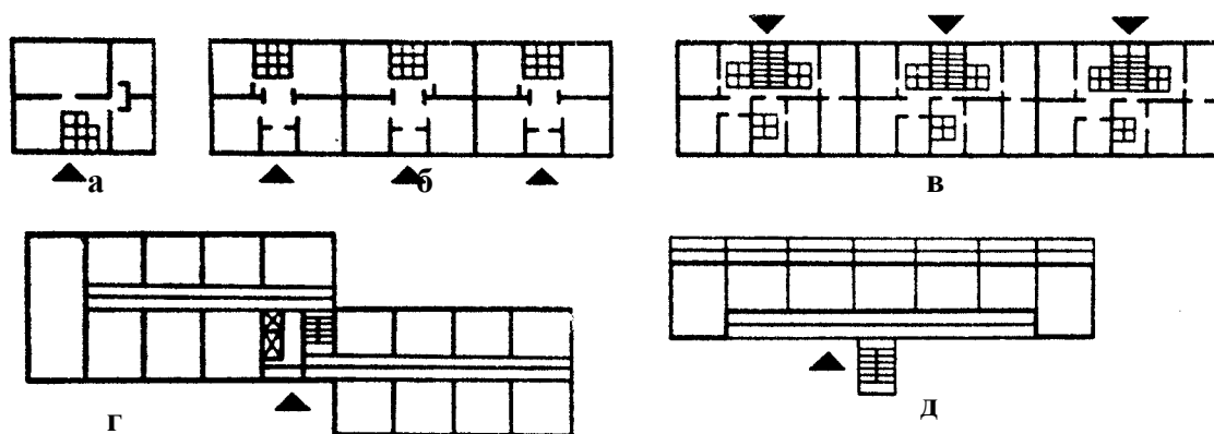
10-расм. Тураржой биоларига хос режавий композициялар: а - бир хонадонли; б - блокировкали; в-секцияли; г-коридорли; д-галереяли.
