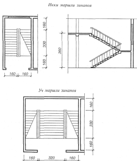
49-расм. Энг кўп қўлланиладиган зиналарнинг турлари.
