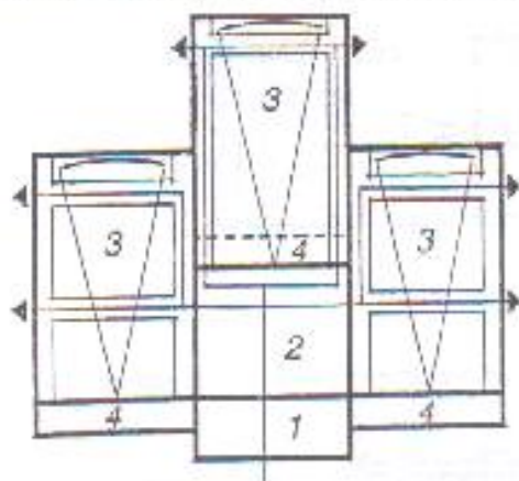
68-расм. Уч залли кинотеатрларнинг композициявий схемалари: 1-вестибюль; 2-фойе; 3-томоша зали; 4-кинопроекция хонаси
