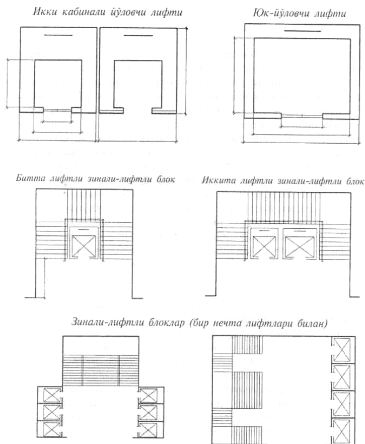
50-расм. Жамоат биноларидаги лифтлар.
