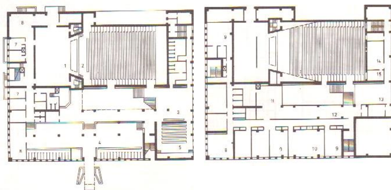
76-расм. 500 ўринлик залли шаҳар клуби: 1-эстрада; 2-томоша зали; 3-фойе; 4-вестибюл; 5-аудитория; 6-болалар билан шугулланиш хонаси; 7-артистлар хоналари; 8-омборхоналар; 9-клубоклар хоналари; 10-ўқув зали; 11-буфет; 12-кўрғазма зал; 13-меҳмонхона; 14-кинопроекцион хонаси; 15-товуш аппаратлари хонаси
