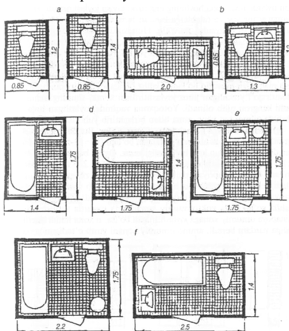
30-расм. Ҳожатхона ва ванна (обзан) хоналар лойиҳаси:
