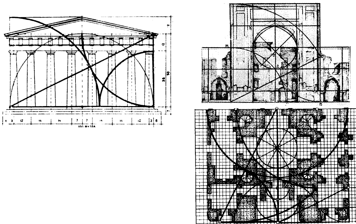
18-расм. Архитектурада пропорция (меъморий уйғунлик) асосида бино этилган обидалар: А- Афинадаги Парфенон биносининг тарзи; Б- Самарқанддаги Ишратхона мақбарасининг тарзи ва тарҳи.
