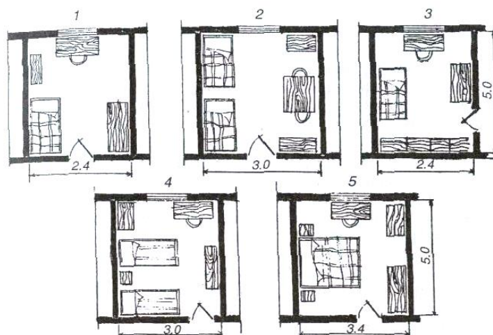
26-расм. Ётоқхоналарнинг тахминий лойиҳаси ва мебелларни жойлаштириш:
