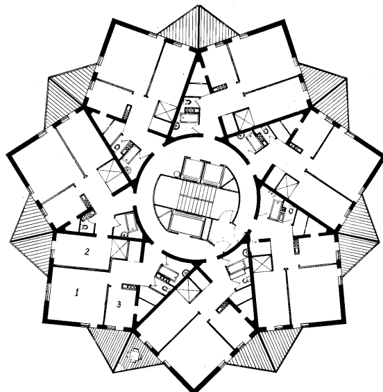
15-расм. Ўққа нисбатан симметрия. Кўп қаватли тураржой биноси (макети ва тарҳи).
