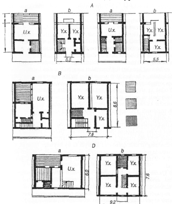
32-расм. Зинапояларнинг хонадон ичида жойлашиши: А - уч хонали хонадон; Б - тўрт хонали хонадон; Д - беш хонали хонадон; а - биринчи қават; б - иккинчи қават.
