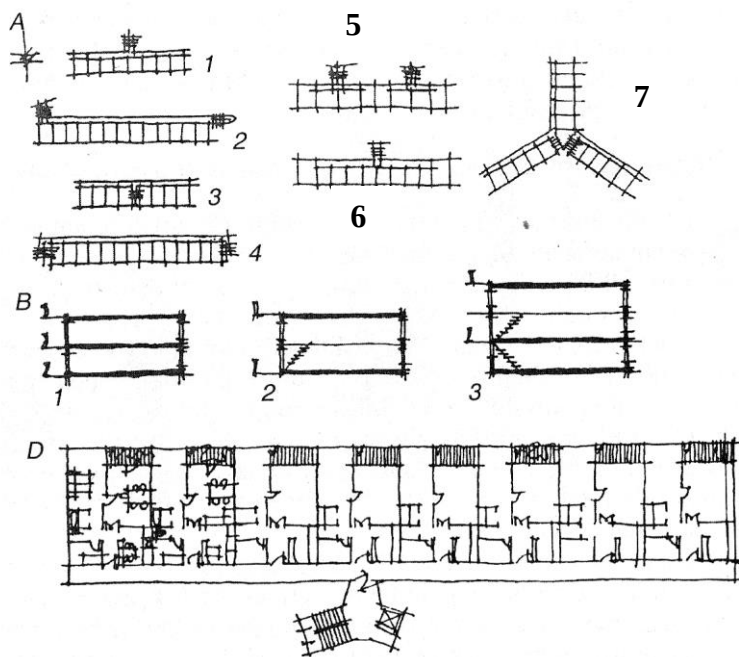
40-расм. Галереяли уйлар: а) галереяли уйлар схемалари: 1-2 – зинапоя уй габаритидан ташқарида; 3-4- зинапоя уй габаритида жойлашган; 5-6 – галереяли секцияли уйлар; уч нузли уй; Б-уйларнинг қирқимлари: 1- қаватдаги йўлак; 2- икки қаватга бир йўлак (икки қаватга жойлашган хонадонлар учун); 3- уч қават учун йўлак; Д-зинапоя уй габаритидан жойлашган 5 қаватли галереяли уй.
