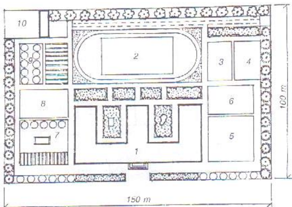
57-расм. Мактаб ҳудудининг режа:
