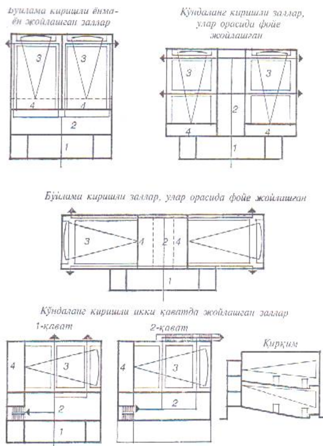
67 -расм. Икки залли кинотеатрларнинг композициявий схемалари: 1-вестибюль; 2-фойе; 3-томоша зали; 4-кинопроекция хонаси
