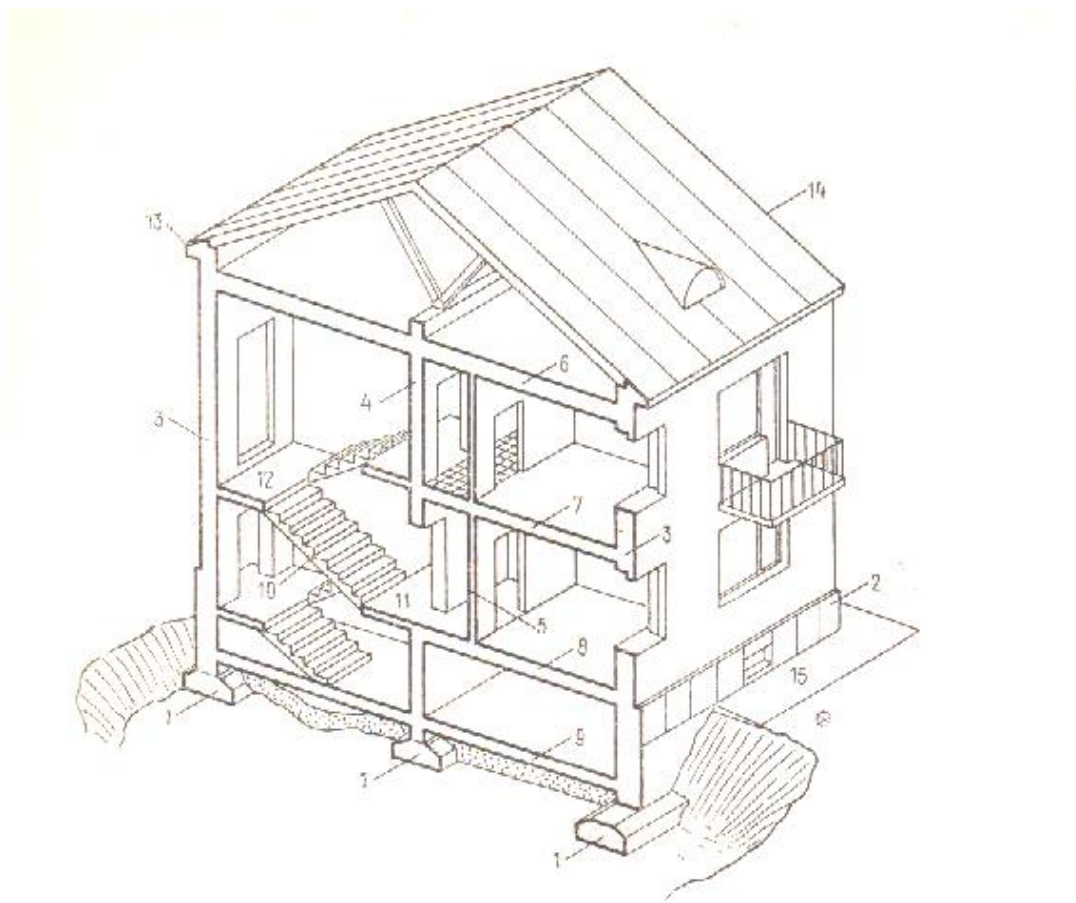
6-расм. Икки қаватли бионинг конструктив таркибий қисмлари:
