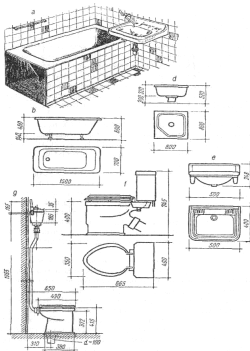
29-расм. Сантехник жиҳозлар:
