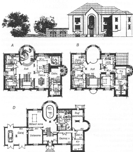
35-расм. Кам қаватли юқори комфортли турар жой биноси: А — биринчи қават тарҳи; Б — иккинчи қават тарҳи; Д — цокол қавати тарҳи.
