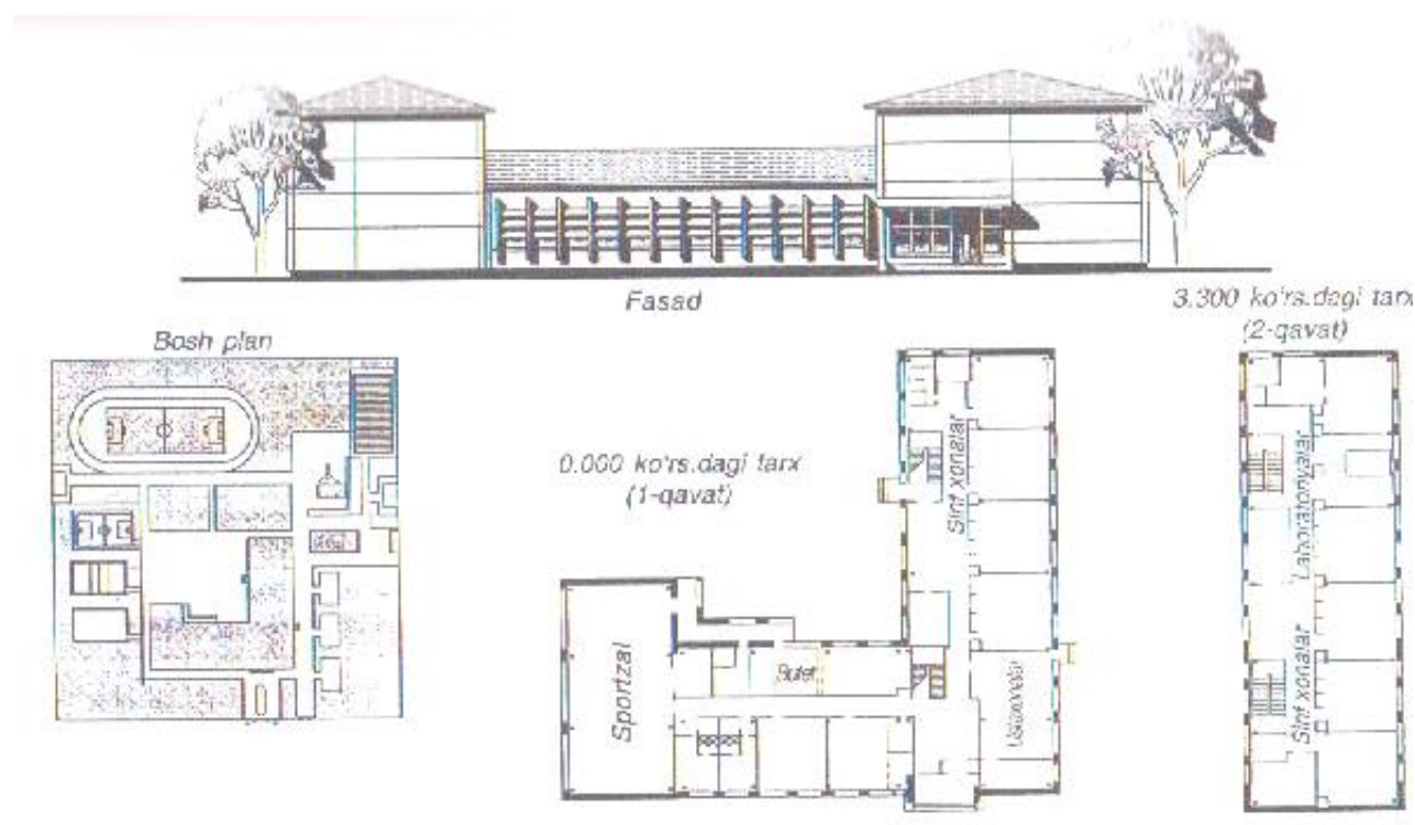
59-расм. 192 ўқувчига мўлжалланган намунавий мактаб лойиҳаси.
