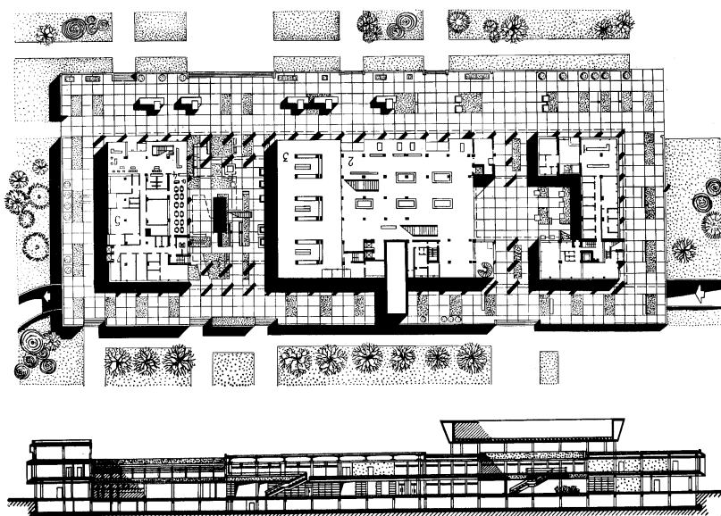
3-расм. Жамоат бинолари. Навоий шаҳрининг савдо маркази. Умумий кўриниши, тарҳи ва қирқими.
