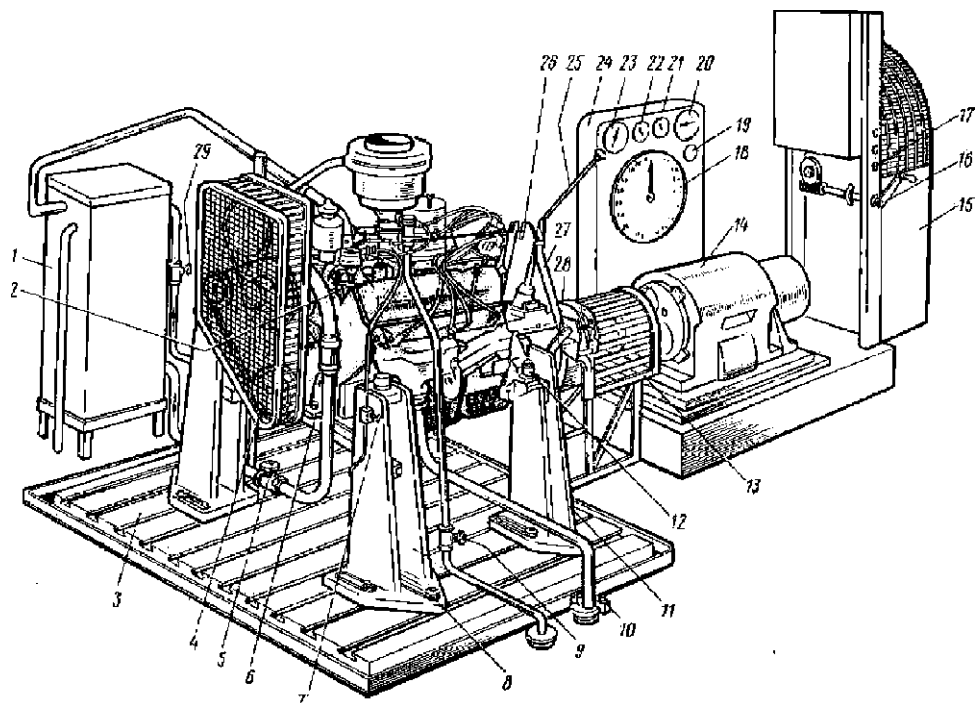
27-rasm. Dvigatelni sinash jihozi: 1-sovitish suyuqligi baki; 2-dvigatel; 3-plita; 4-shkiylarning himoya g'iloqi; 5-sovitish tizimiga keluvchi suvni berkitish krani; 6-dvigatelning oldingi tayanchini mahkamlash gaykasi; 7-suyuq yonilg'i bilan ta'minlash krani; 8-ustunni qotirish gaykasi; 9-yonilg'i berkitish krani; 10-chiqarish quvurini mahkamlash gaykasi; 11-ustun; 12-dvigatelning orqa tayanchini mahkamlash bolti; 13-kardan valini himoya g'iloqi; 14-elektrodvigatel; 15-suyuqlikli reostat; 16-reostatni boshqarish ushlagichi; 17-elektrodvigatelni boshqarish tugmasi; 18-yuklanishni ko'rsatuvchi raqamli ko'rsatkich; 19-ogohlantirish lampasi; 20-taxometr; 21-moy harorati ko'rsatkichi; 22-suv harorati ko'rsatkichi; 23-manometr; 24-124 boshqarish pulti korpusi; 25-uzatmalar qutisi ushlagichi; 26-karbyurator drosselini boshqarish tortqisi; 27-qo'l tormozi richagi; 28-ilshish muftasi tepkisi; 29-vodoprovod suvini berkitish krani.
