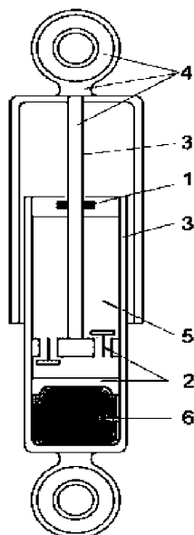
51-rasm. Ishlash jarayonida amortizator-ning shikaslanish va ishdan chiqish joylari.
