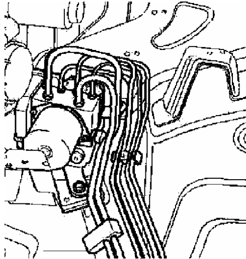
66-rasm XUNDAY avtomobilining avtoblokirovka tizimining(ABS) joylashuv shakli
