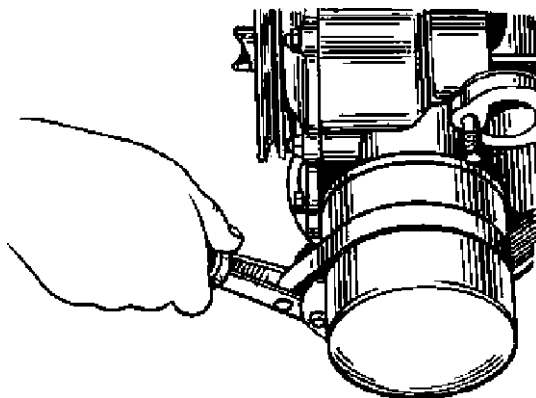
31-rasm. Neksiya va VAZ avtomobil dvigatellarining moy fil'trini yechib olish shakli.
