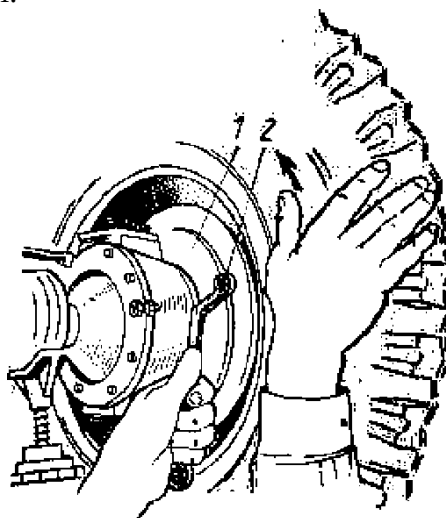
62-rasm. Kolodka va tormoz barabani orasidagi tirqishni sozlash: 1-tayanch disk; 2-barmoq ekstsentrigi
