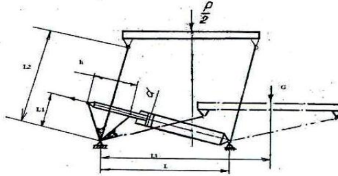
13-rasm. Richagli gidravlik ko'targichning xisobiy sxemasi.
