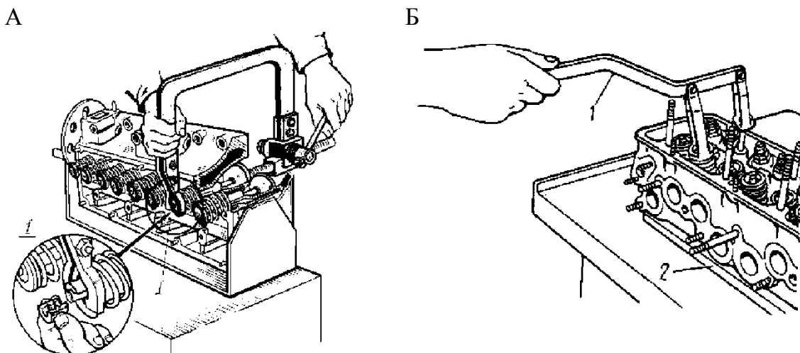
7.24-rasm. Silindr kallaklarini bo'laklarga ajratish shakli: 1-klapan birikmasini yechish moslamasi; 2-klapanlarni harakatini chegaralovchi taglik
