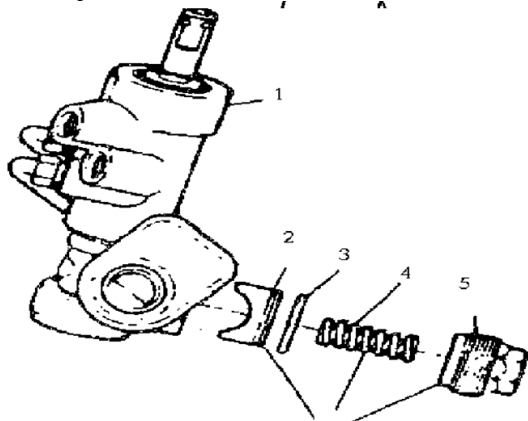
60-rasm. Reyka va vint orasidagi tirqishni sozlash: 1-rul karteri; 2- plunjer; 3-zichlashtirish halqasi; 4-prujina; 5- sozlovchi tiqin; 6-chegaralovchi gayka.
