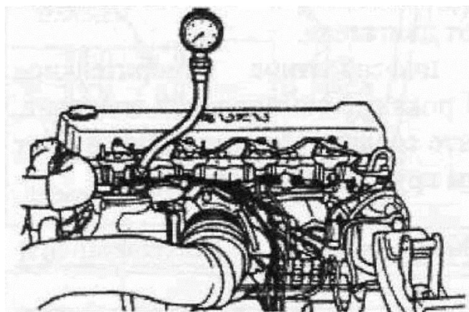
14-Rasm. Manometrli (a) va o'zi yozuvchi (b) kompressometrlar hamda Isuzu avtomobili dvigatelining kompressiyasini o'lchash shakli (s).
