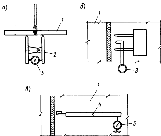
7.5-расм. Пайвандлаш пайтида деформация ва кўчишни аниқлаш схемаси:
