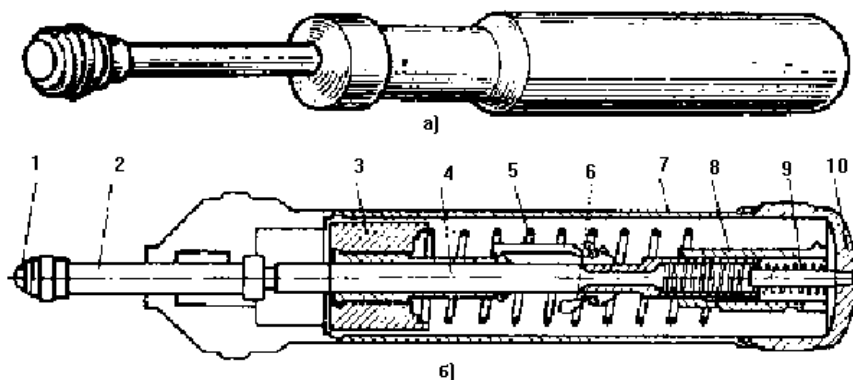
9.1-rasm a) umumiy ko'rinish; b) pribor sxemasi; 1-sharcha, 2-zarba beruvchi sterjen, 3-
