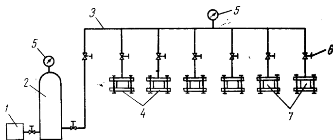
2.3-расм. Намуна плиткаларни сув ўтказувчанликка синов ускунаси.
