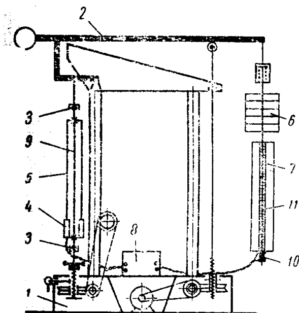
10.3-расм. Арматура пўлатини релаксацияга синаш қурилмаси схемаси: 1-станина (мустаҳкам пўлат асос); 2-ричаг
