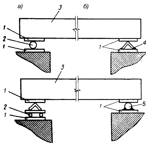
31-расм. Таяниш схемалари:
