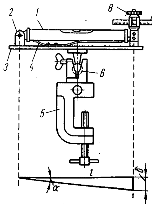
8.6-рaсм. Стопани клинометри:
