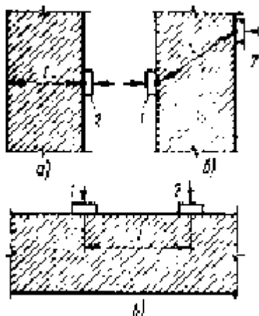
5.2-rasm. Betondan tovush o'tishi sxemasi.
