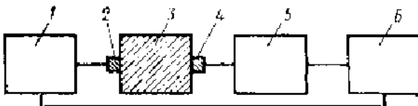
13.5-rasm. Betondagi ultratovush tezligini aniqlash sxemasi.
