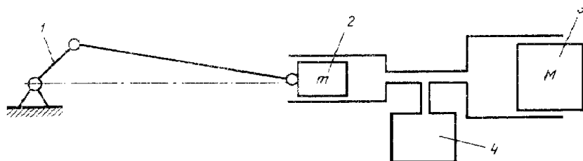
2.6 rasm. Pulunjerli gidropulg'sator sxemasi.
