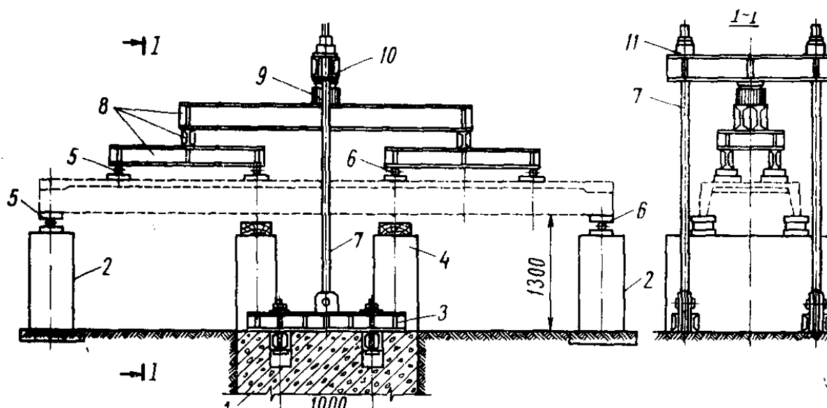
32-rasm. Plitani stendda sinash sxemasi:
