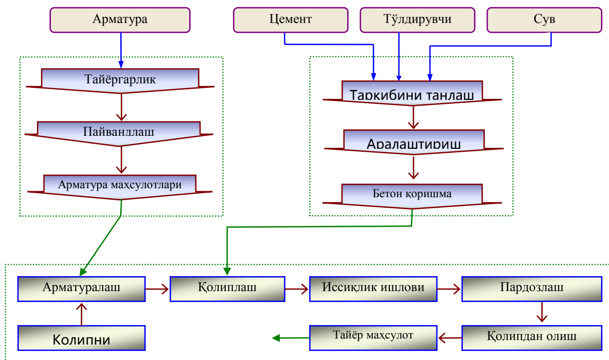
Yig'ma temirbeton ishlab chiqarish zavodida nazorat bosqichlari sxemasi
