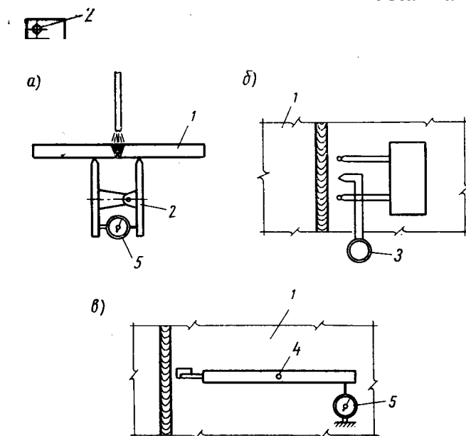
14.5-рasm. Пайвандлаш пайтида деформация ва кўчишни аниқлаш схемаси:
