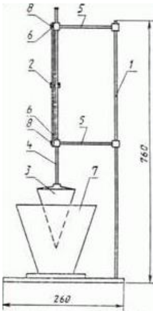
8.1-рasm. Қоришма аралашмасини ёйилувчанлигини аниқлаш прибори 1- штатив; 2- шкала; 3-эталон конус;
