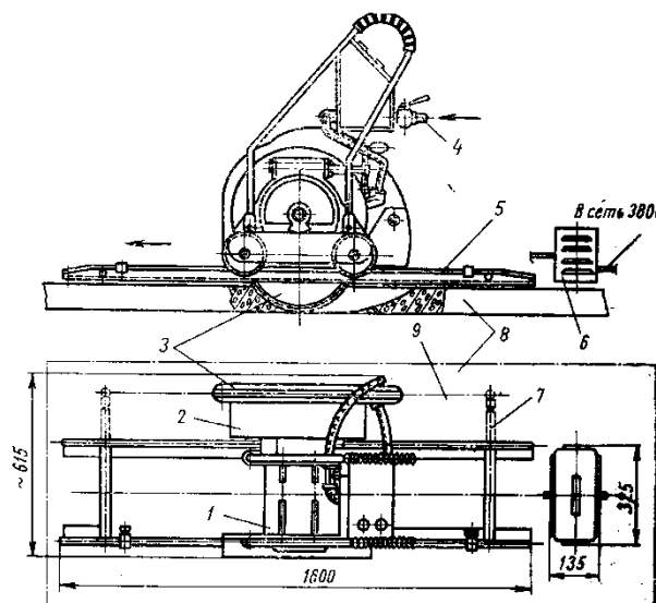
3.1.-rasm.URJ-2 stanogi:
