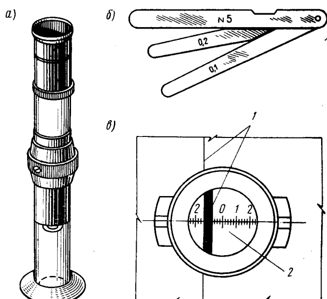
8.9-расм. Дарзларни ўлчаш приборлари:
