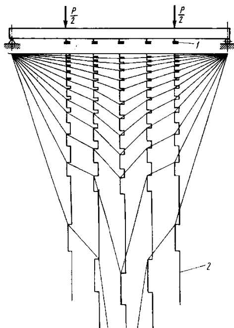
8.5-rasm. Tusinni IPD-1 pribori bilan sinalganda salqiliklar yozuvi sxemasi:
