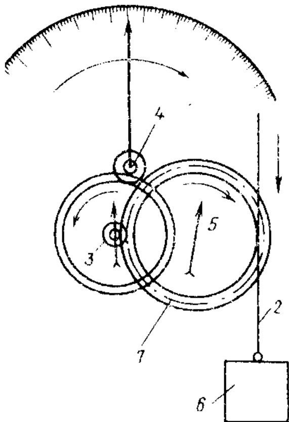
8.4-rasm. Progibomer knematik sxemasi
