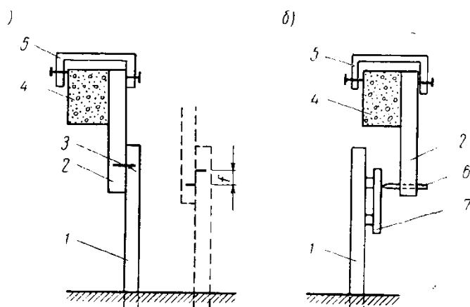
8.1-rasm. Sodda uskunalar yordamida salqilikni aniqlash sxemasi:
