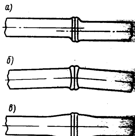
14.4-расм. Контактли пайвандлашдаги нуқсонлар.
