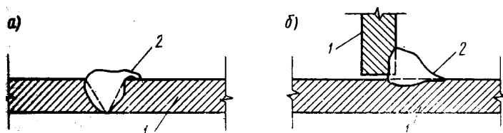
14.2-расм. Пайванд қуйқаси:
