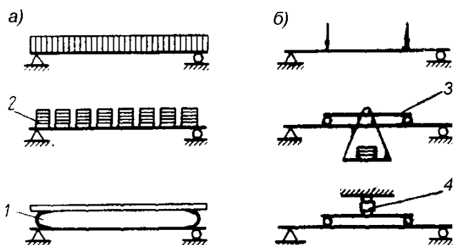
30-расм. Конструкцияларни юклаш схемалари:
