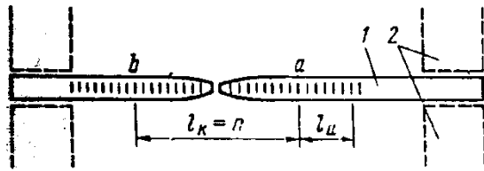
6.1-rasm. Armatura po'latidan olingan namunaga belgi qo'yish sxemasi:
