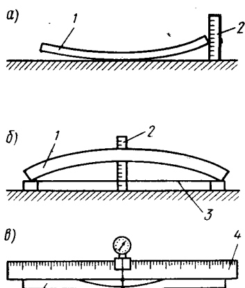
14.7-рasm. Металл маҳсулот ва қурилмаларни пайвандлашда ҳосил бўладиган қолдиқ кўчишларни ўлчаш схемаси.
