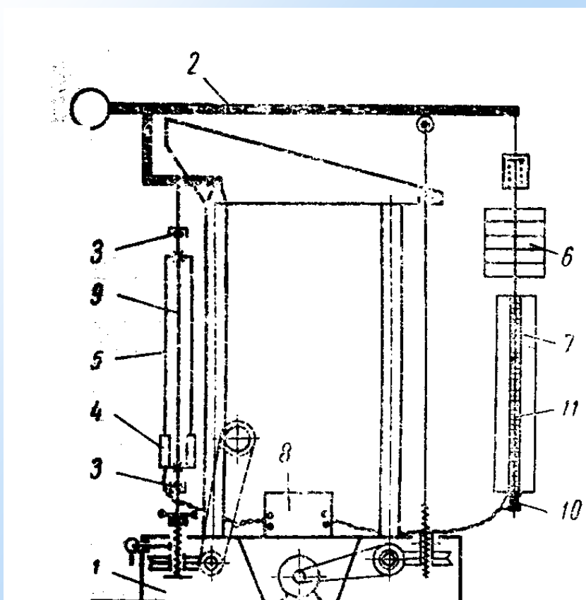
Armatura po'latini relaksatsiyaga sinash qurilmasi sxemasi
