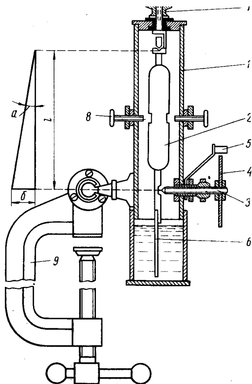
7-расм. Аистов клинометри КА-4:
