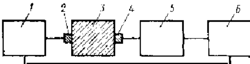
5.1-rasm. Betondagi ulg'ratovush tezligini aniqlash sxemasi.
