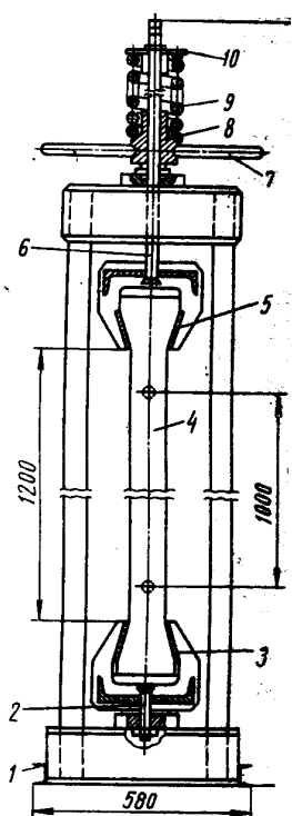
3.5-Расм.Давомий чўзиш учун қўлланиладиган қурилма схемаси:
