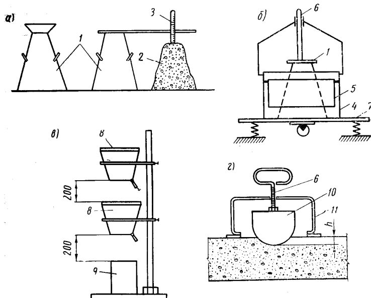
4.1-Расм.Бетон қоршмасини ёйилувчанлиги ва қаттиқлигини аниқлаш:
