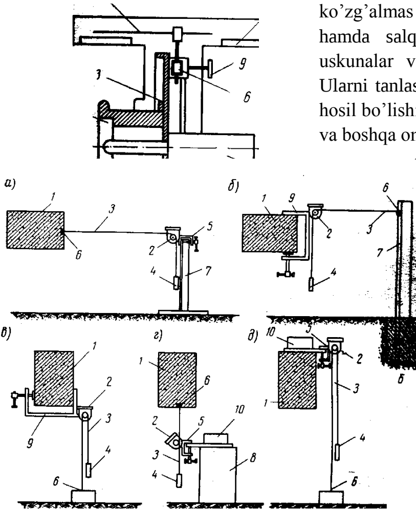
8.3-Rasm.Progibomerlarni o'rnatish sxemalari: a, b-konstruktsiyani gorizontal holda sinalganda; v, g, d-konstruktsiyani vertikal holda sinalganda;
