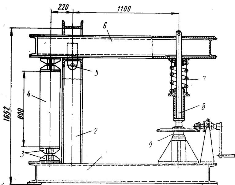
3.4-рasm. Давомий сиқиш учун мўлжалланган пичаг-пружинали кўпикма схемаси
