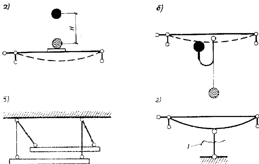
2.5.rasm. Gravitatsion kuchlar yordamida tebranish hosil qilish sxemasi.
