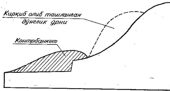
6.4 – расм. +ияликларни яссилаб ва контрбанкет +уриб уларнинг мустацкамлигини ошириш схемаси.
