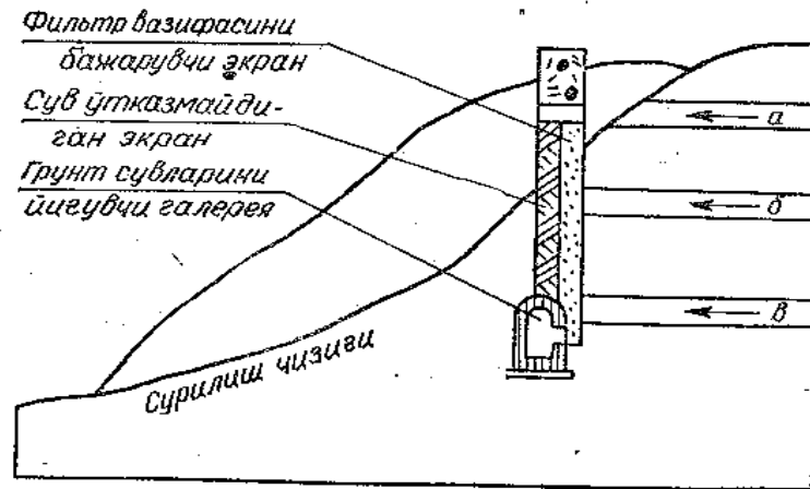
6.5 – расм. Дренажли галереянинг суриладиган +ияликда жойланиш схемаси:(М.З.Назаров расми). а, б, в – сувли =атмлар.
