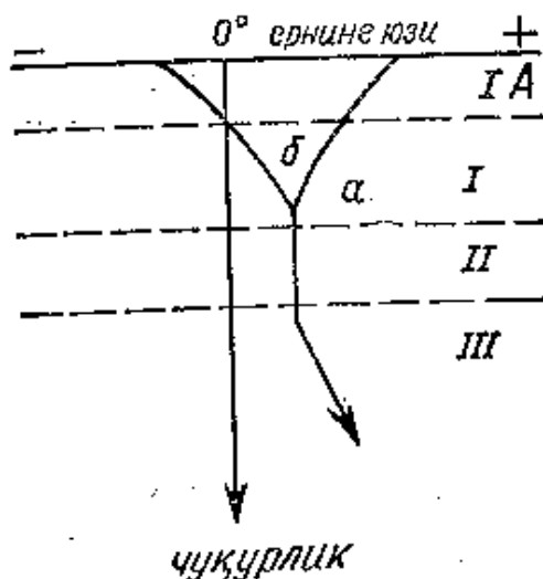
2-расм. Ер ичида температу- ранинг тақсимланиш схемаси
