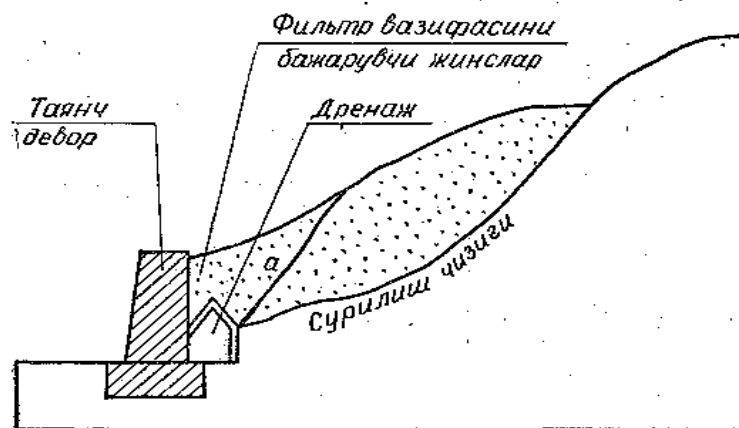
6.6 – расм. Суриладиган +ияликни таянч девор ёрдамида мустацкамлаш.
