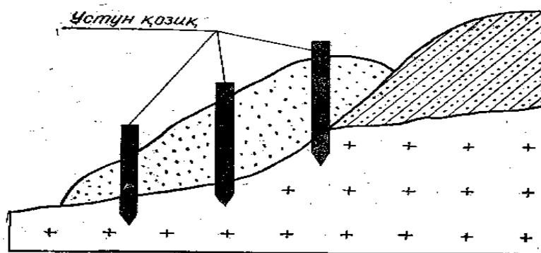
6.3 – расм. Суриладиган =ияликни устун =ози\лар ёрдамида мустацкамлаш (/О.Мавлонов, С.Зоцидов расми.).
