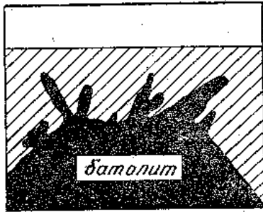
3.1-рasm. Магматик жинсларининг магмадан шосил боелиш схемаси: 1-чуқурликдаги 2-ер устига чикиб қолганлари
