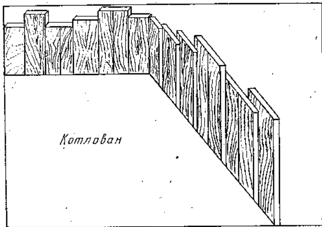
6.10 расм. Котлован атрофига оёрнатилган шипхатли деразалар.
