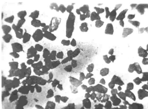
9.1 – rasm. Boyitilgan Qoratog' fosforiti flotokonsentrati zarrachalarining mikrosurati.
