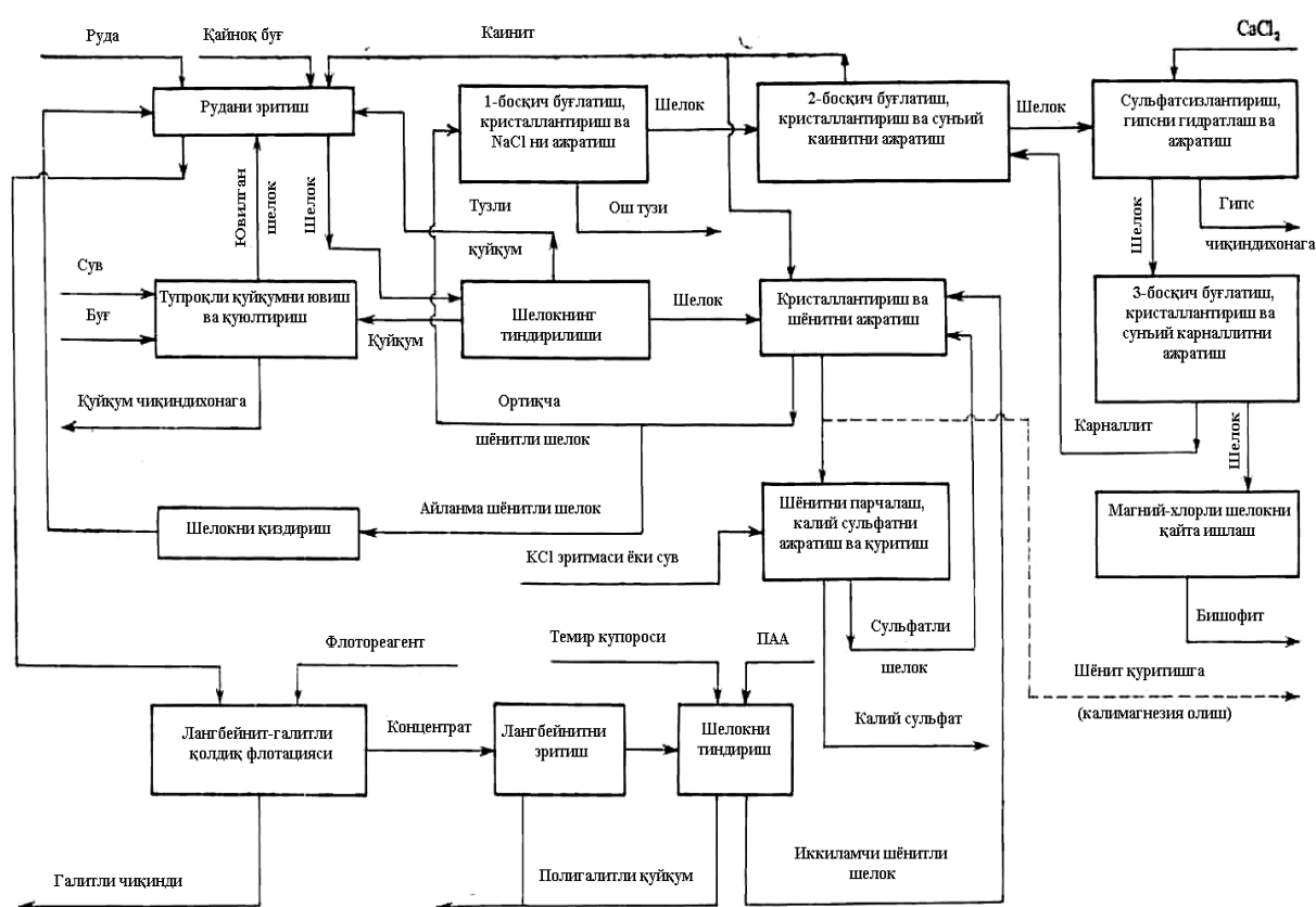
7.7 – rasm. Prikarpatiya polimineral rudasini qayta ishlash sxemasi.
