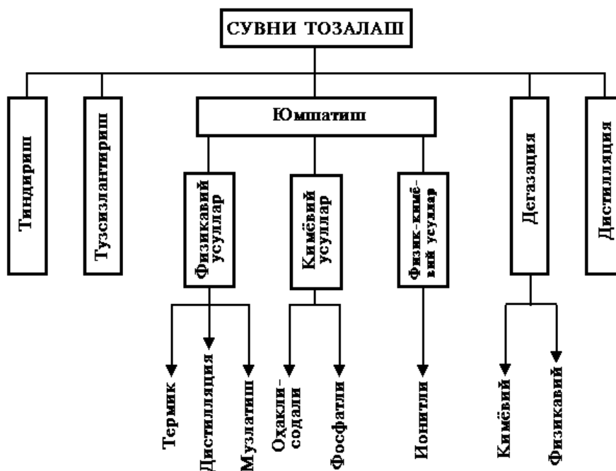
4.1 – rasm. Suvni tozalash sxemasi.
