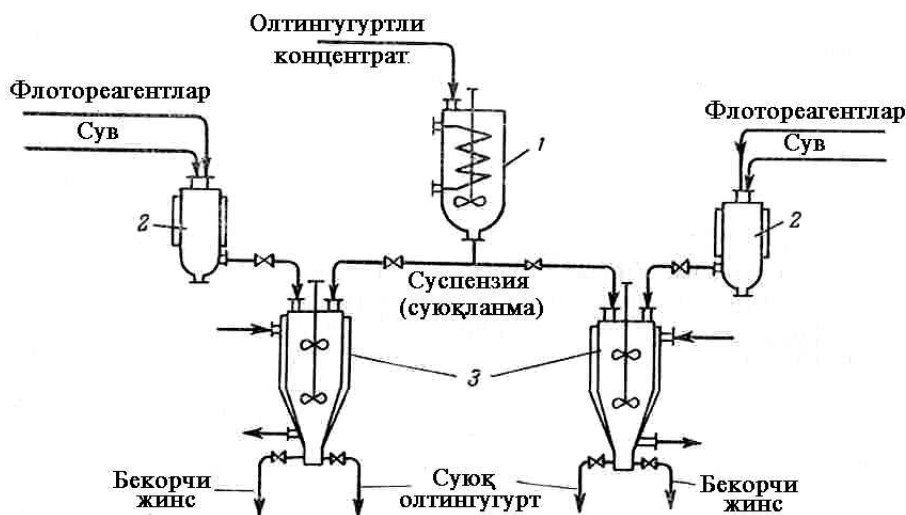
6.1 – rasm. Avtoklavlarda flotatsiyalash orqali oltingugurtli konsentratlardan oltingugurt olish sxemasi:
