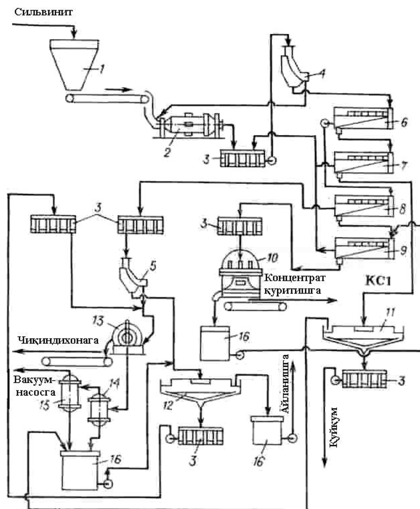
7.4 – rasm. Oldindan tuproqli quyqum flotatsiyalangan silvinitdan kaliy xlorid ishlab chiqarishning flotatsiyali usuli sxemasi.
