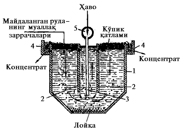
2.5 – rasm. Havo yordamida aralashtiriladigan flotatsiya mashinasi:
