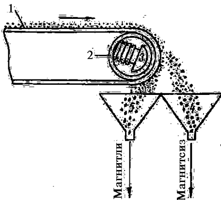
2.3 – rasm. Elektromagnit separator (ajratgich) sxemasi:
