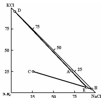
6.1-rasm. Kaliy xlorid taqsimlanishi hisobi uchun e.q. – NaCl – KCl sistema diagrammasi.
