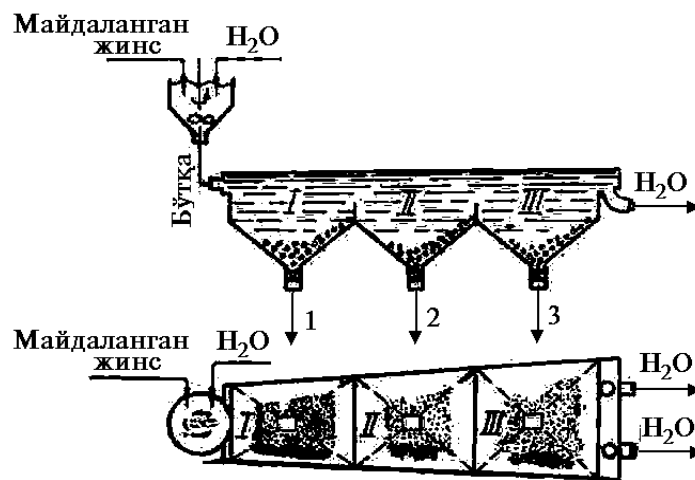
2.1 – rasm. Ho‘l gravitatsion boyitish sxemasi:
