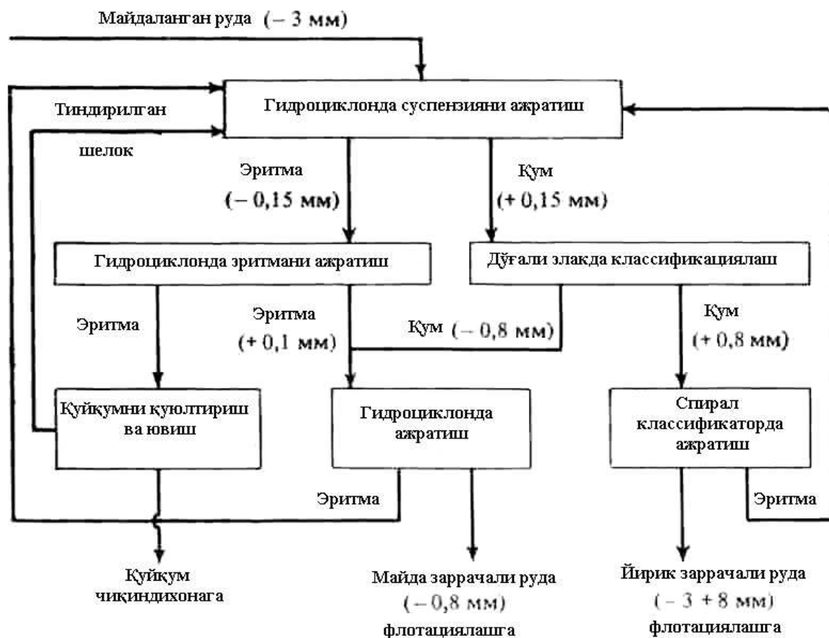
7.2 – rasm. Silvinit rudasini quyqumsizlantirish sxemasi.
