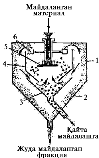
2.2 – rasm. Havo separatorining sxemasi:
