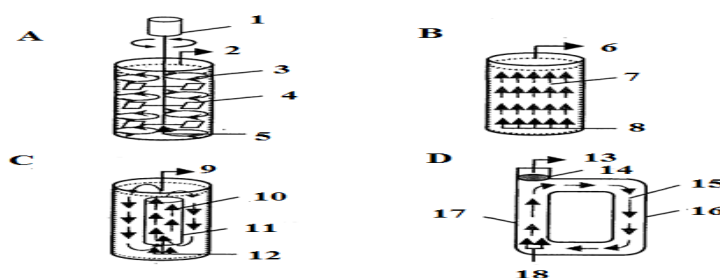
5-rasm. Turli tipdagi bioreaktorlarning soddalashtirilgan shemasi:
