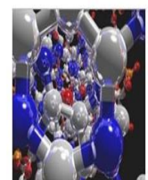
ХИМИЯ
