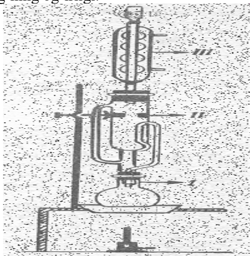
14.1.-rasm. Sokslet apparati.
