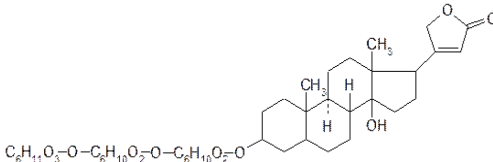
Digitoksin
