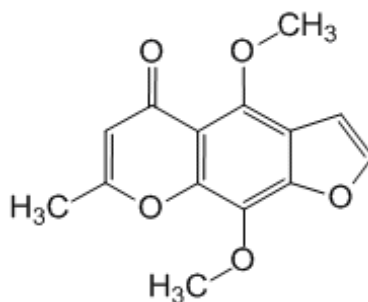
Kellin
