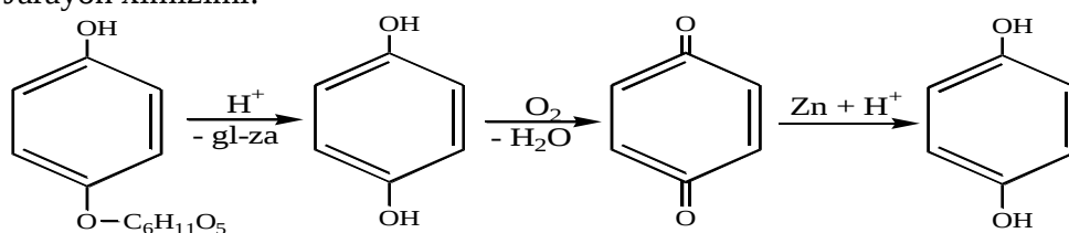
Arbutin
