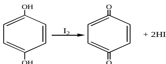
Arbutin
