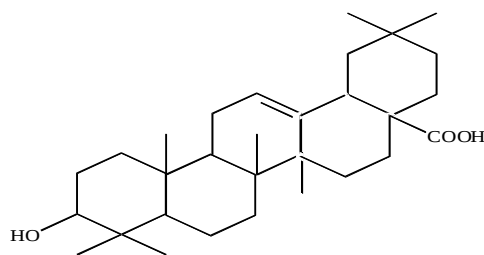
Oleanolkislota
