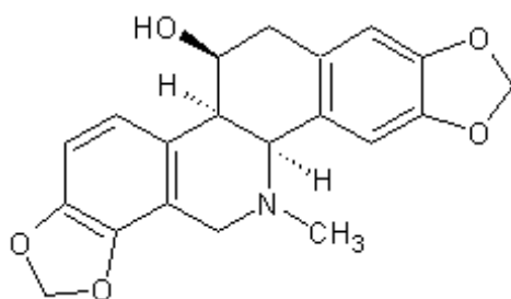
Xelidoiin
