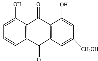
Aloe emodin
