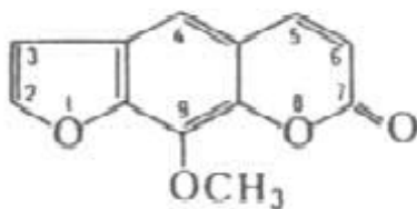
Kantatoksin
