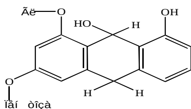
Jasterin
