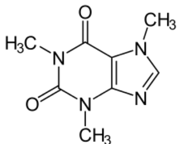
Kofein
