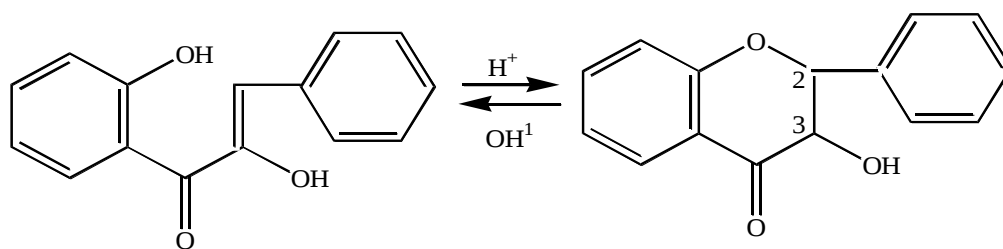
Flavonon
