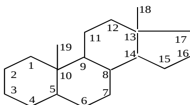
Siklopentan pergidrofenantren
