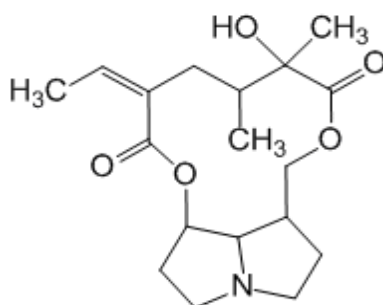
Platifillin
