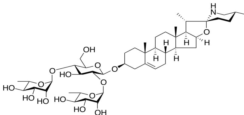
Solamargin
