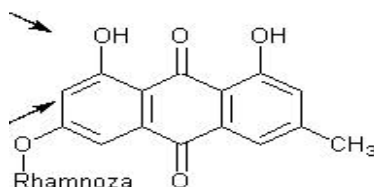
Frangulin A
