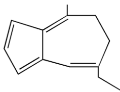
Xamazulen
