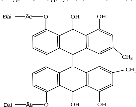
Frangularozid
