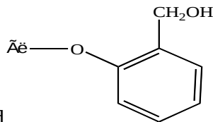
Salitsin
