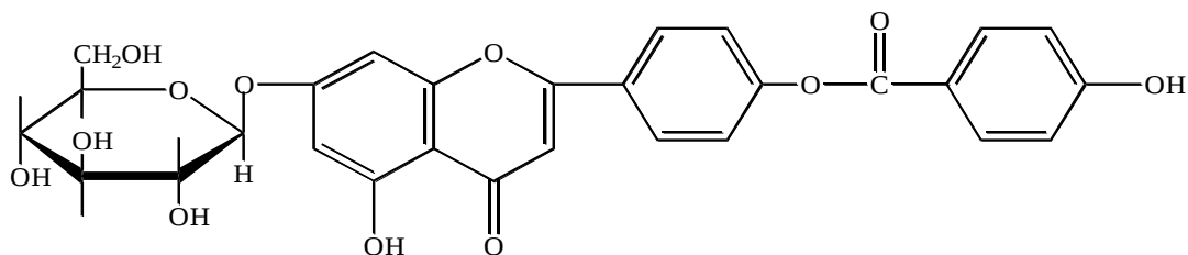
Kvinkvelozid
