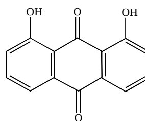
Xriaofanol
