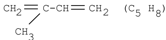
Izopren
