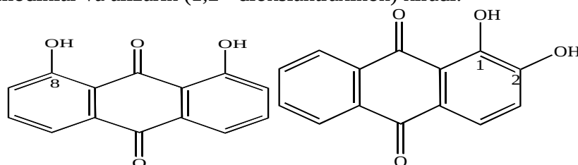
Xrizatsin
