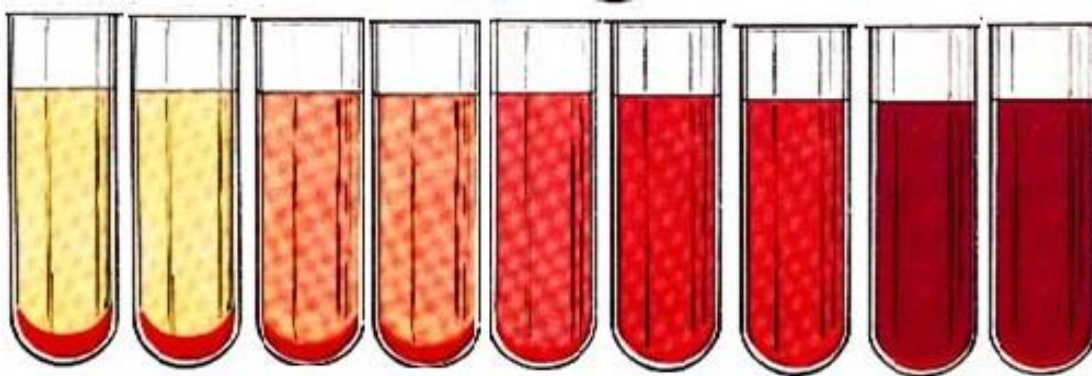
1.2.-rasm. Gemolitik ko'rsatkich (indeks) ni aniqlash.
