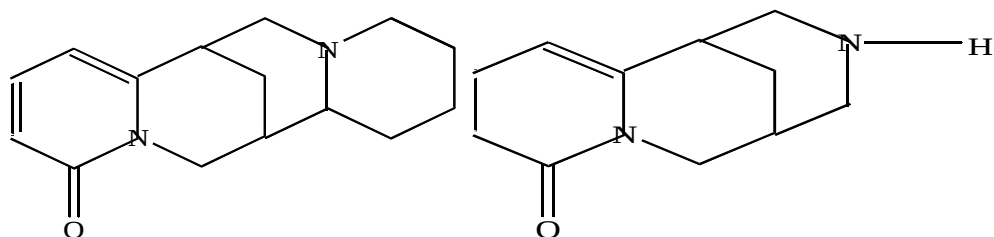
Termopsin
