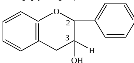
Katexin (3 - flavanol)
