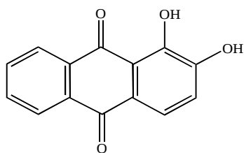
Alizarin
