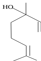
Linnaol
