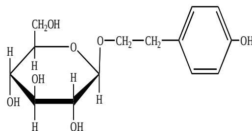
Salidrozd (rodiolozid)
