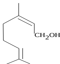
Geraniol
