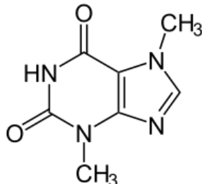
Teobramin
