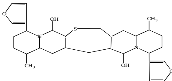
Nuflein
