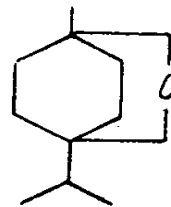
Sineol
