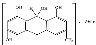
Jasterin
