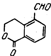
Eritrotsentaurin
