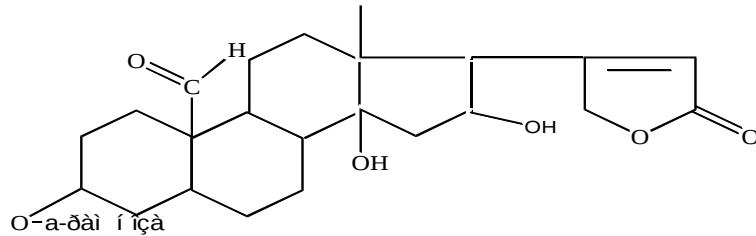
Adonitoksin
