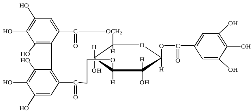
Korilagin
