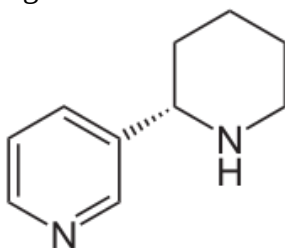
Anabazin
