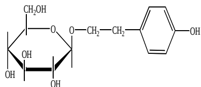
Salidrozd
