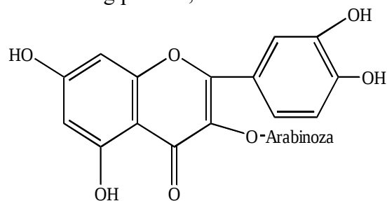
Avikulyarin
