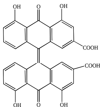
Direin
