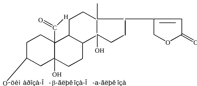
K- strofantozid
