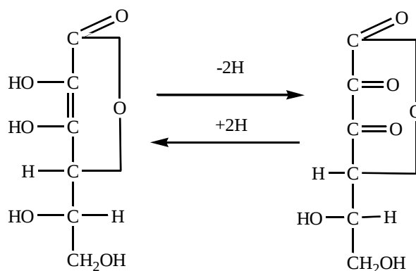
Degidroaskorbin kislota
