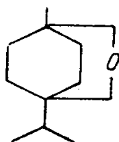
Sineol
