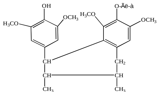
Feligozid
