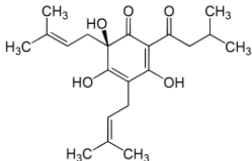
Xumulin alkaloidi
