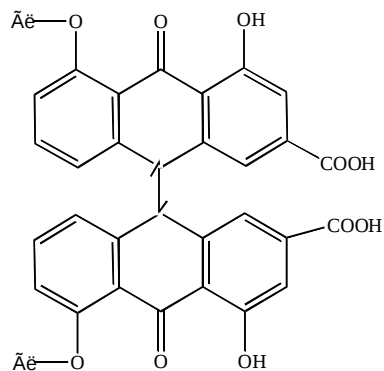
Sennozid A,B
