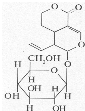
Sverozid
