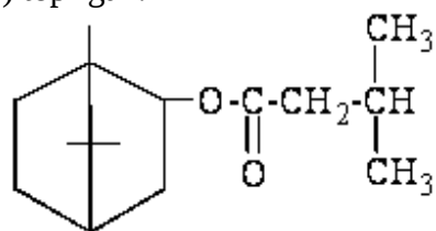
Bornilizovalerianat
