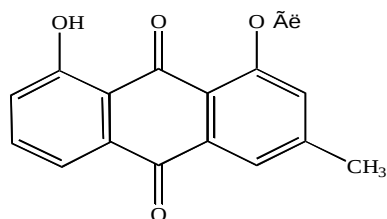
Xrizafanol
