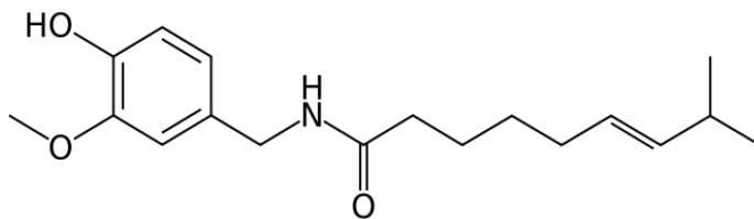
Kapsaitsin
