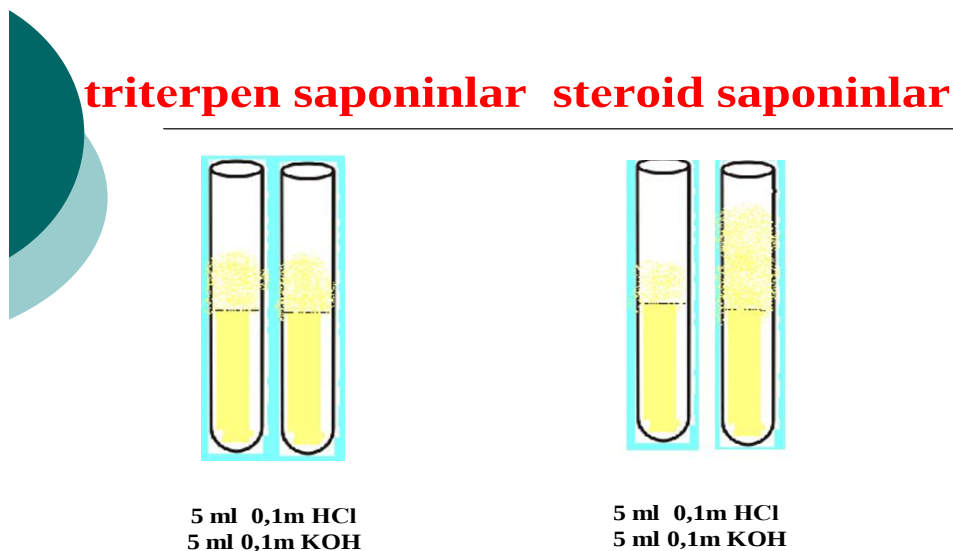
1.1.-rasm. Fontan Kandel reaksiyasi yoki tasnifi reaksiyasi.
