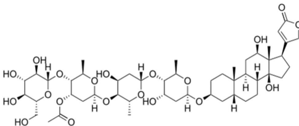
Lantozid C
