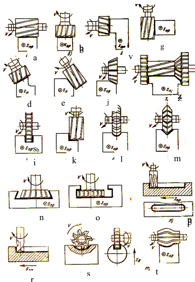
20.3- rasm. Frezerli ishlov berish sxemalari.
