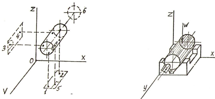
8.4-rasm Silindr detallarni asoslash
