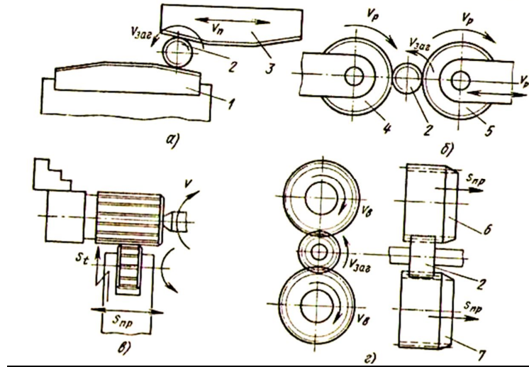
23.4-rasm. Juvalash sxemalari.
