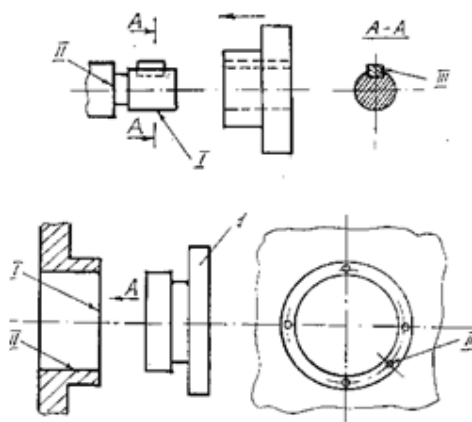
1.4-rasm. Yordamchi bazalar.
