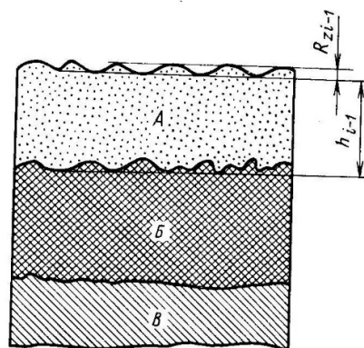
14.1-rasm. Quyimga tasir etuvchi omillar.
