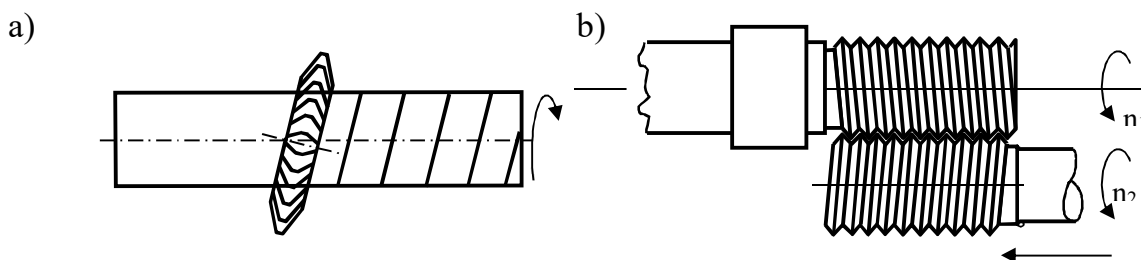
9.7- rasm. Rezbalarni a-diskli va b-guruxli frezalash.
