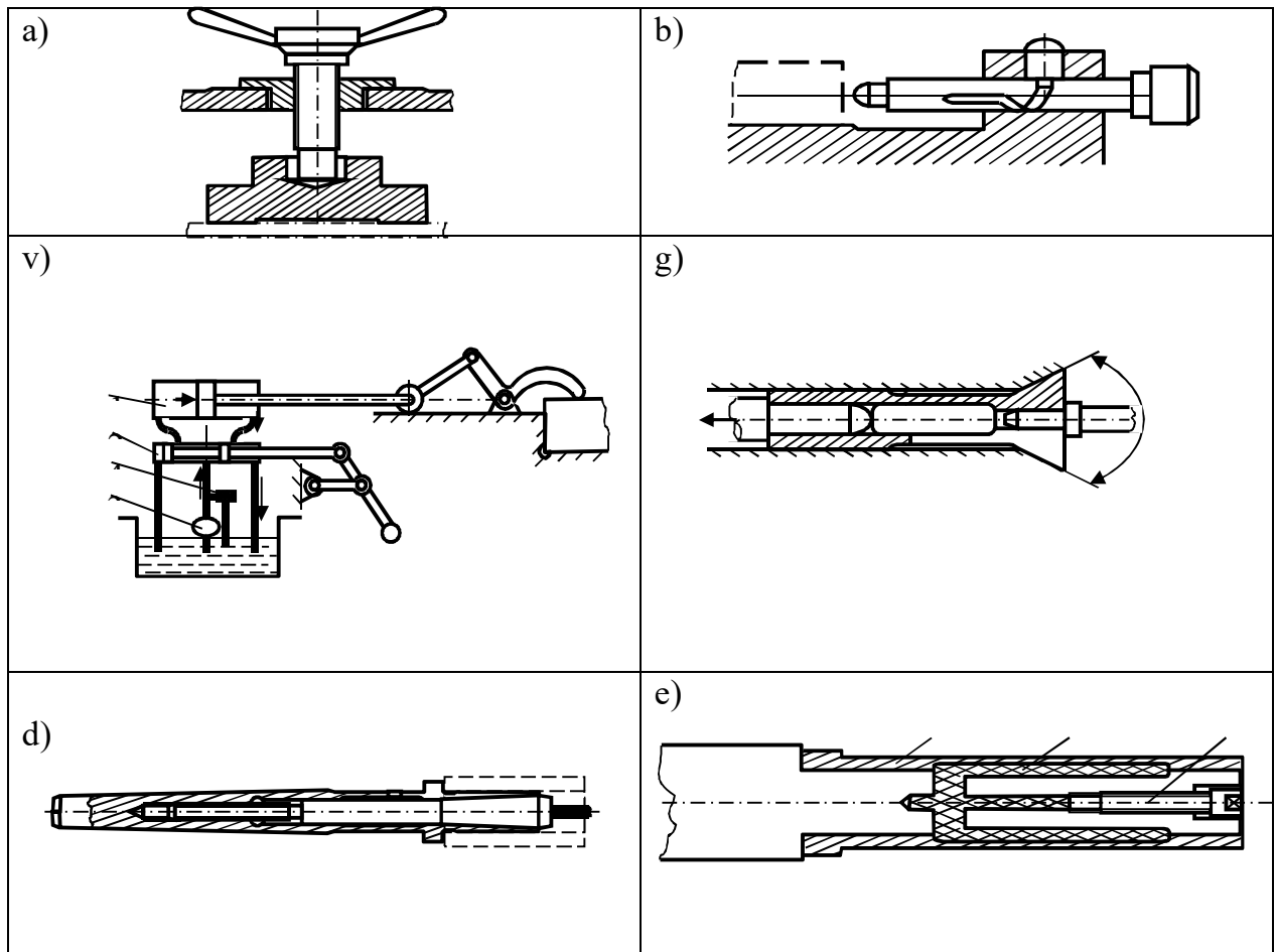
18.11-rasm. Moslamalarda qisuvchi qurilmalar.
