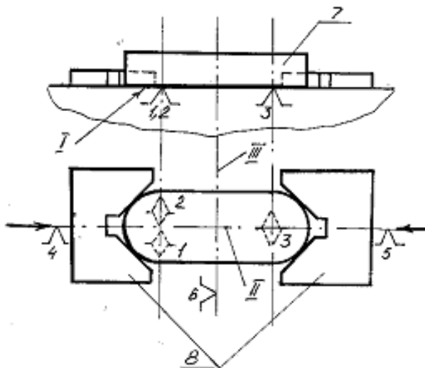
1.10-rasm. Tayyorlamani moslamaga bazalash sxemasi.
