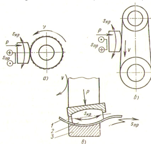
24.8-rasm. Yaltiroqlash sxemalari.
