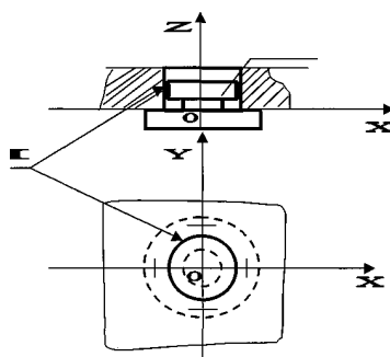
1.9-rasm. Disk shaklli detalni bazalash sxemasi. I-qo'shaloq tayanch bazasi (X va U o'qlari bo'yicha siljishni yo'qotadi)
