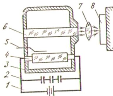
25.9-rasm. Optik kvantli generator sxemasi.
