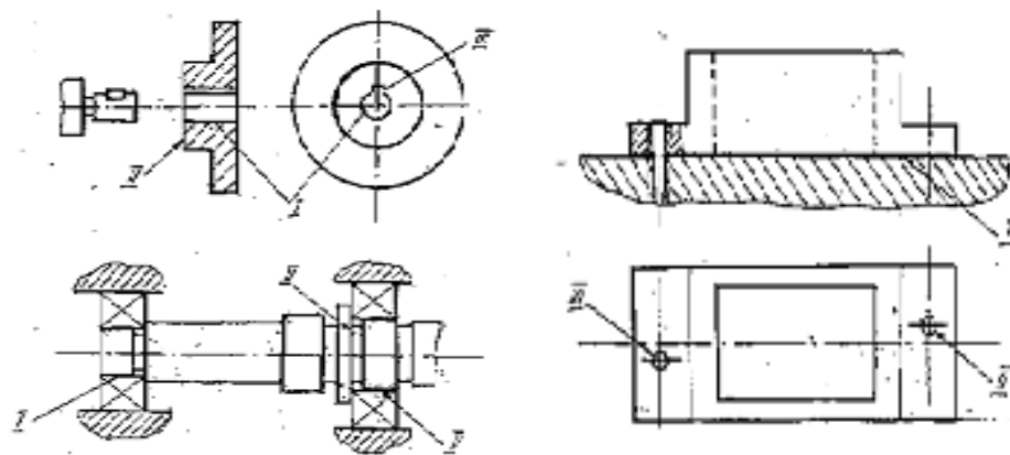
1.3-rasm Asosiy bazalar.
