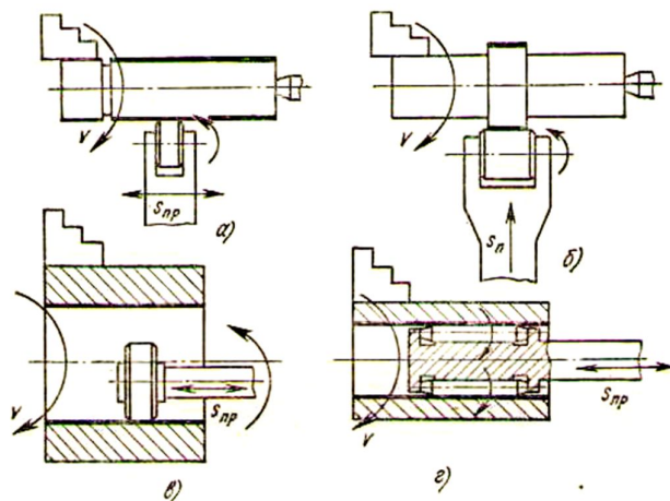
23.1-rasm. Tayyorlama yuzalarini juvalash sxemalari.
