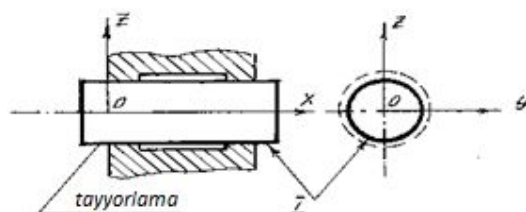
1.8-rasm. TSilindr shaklli detalni bazalash sxemasi.
