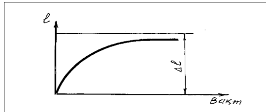
3.4-rasm. Keskichning issiqlik ta'sirida uzayishi grafigi.
