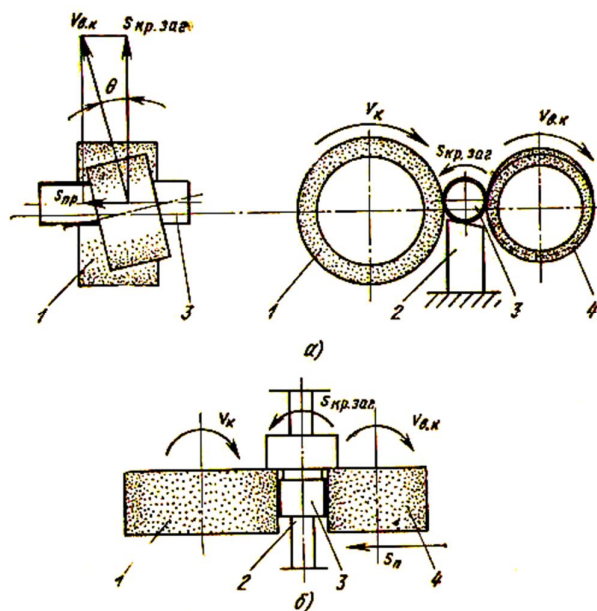
24.3-rasm. Markazsiz jirvilash sxemalari.
