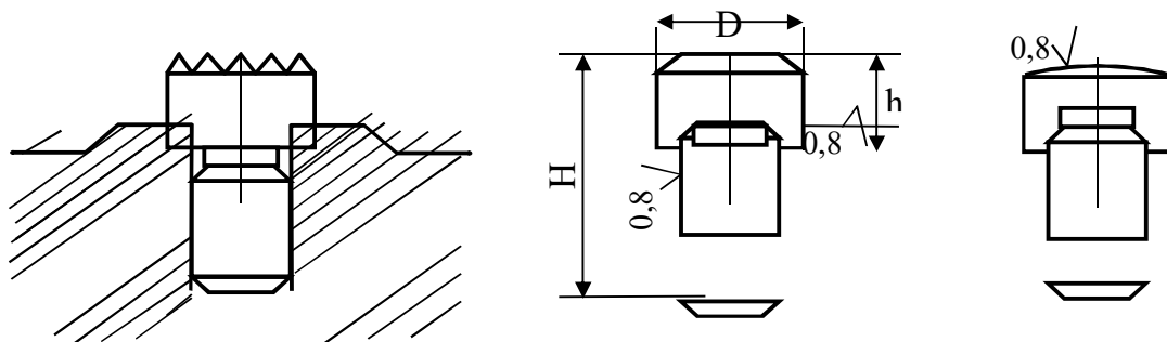
18.1-rasm. Moslamaning tayanch elementlari.
