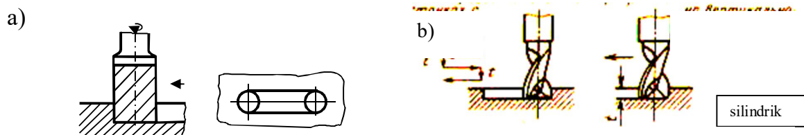
20.12- rasm. Oxirli frezalar bilan shponka uyalarini frezalash.
