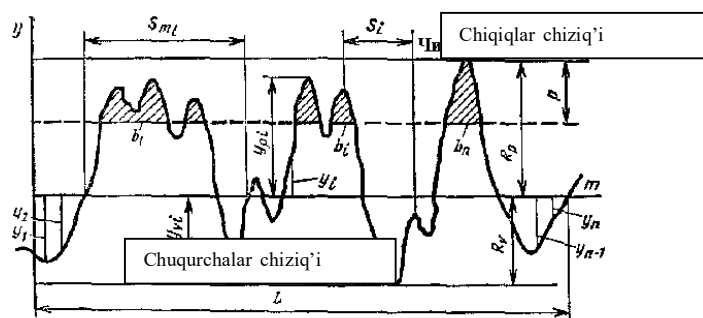
12.1-rasm. Yuzaning profilogrammasi va g'adir-budurlikning asosiy ko'rsatkichlari.
