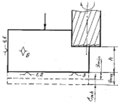
2.1-rasm. Mahkamlash xatoligini xisoblash sxemasi.
