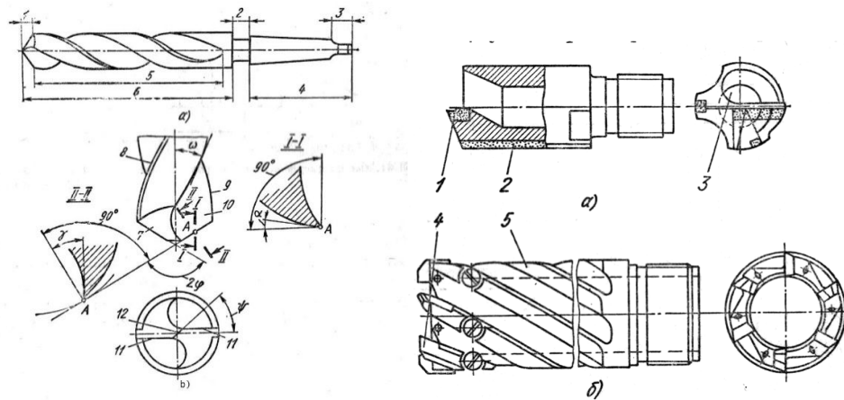
19.7-rasm. Teshiklarga ishlov beruvchi asboblarning sxemalari.
