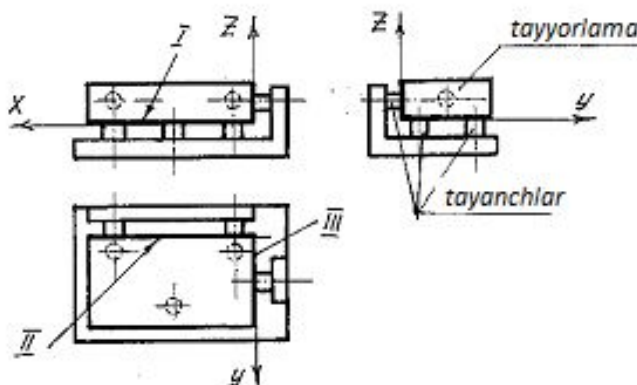
1.7-rasm. Prizma shaklli detalni bazalash sxemasi.
