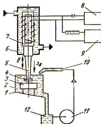
25.6-rasm. Ultratovushli ishlov berish sxemasi.
