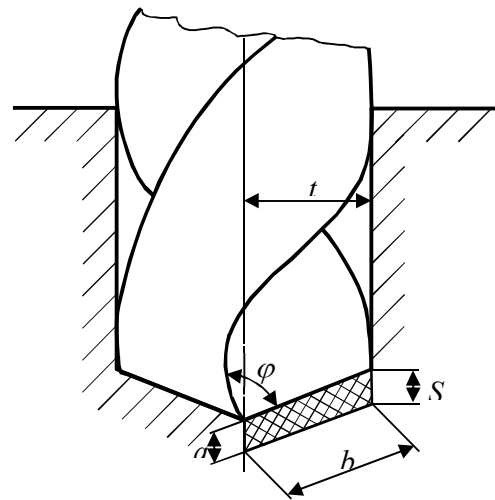
19.9-rasm. Qirindi qalinligi va enini aniqlash sxemasi.
