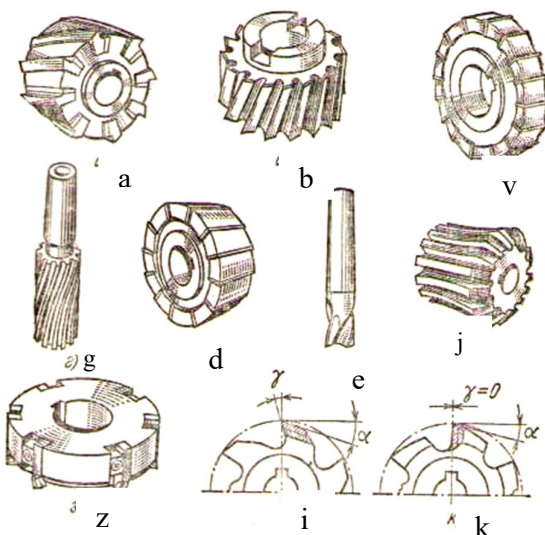
20.2-rasm. Frezalar turlari.
