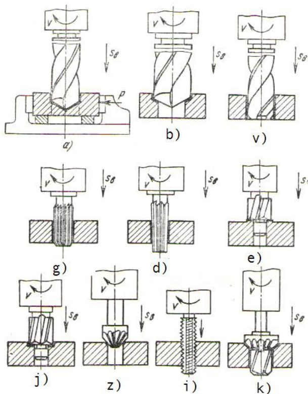
19.6-rasm. Teshiklarga ishlov berish sxemalari.
