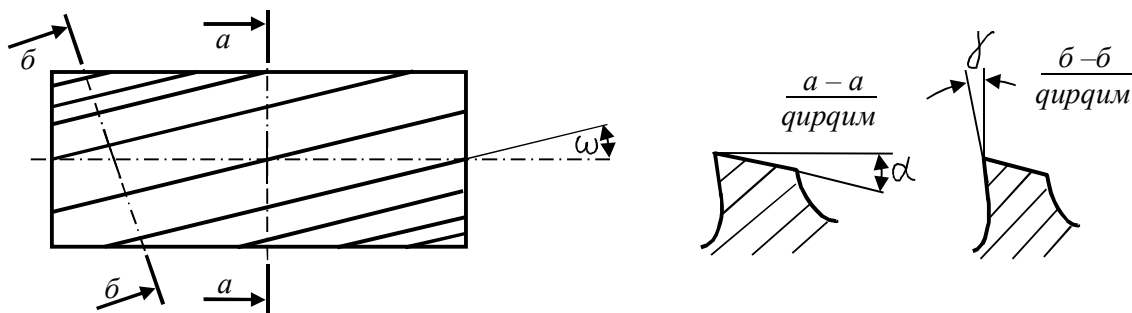
20.4 –rasm. Silindrik frezaning geometrik parametrlari.
