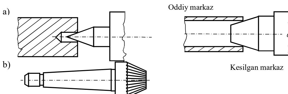
18.8- rasm. Markazlash elementlarining turlari.
