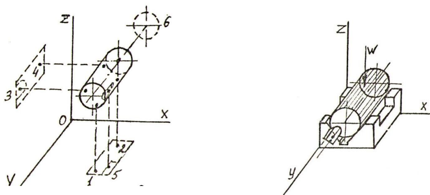
6.2-rasm. Silindr detallarni asoslash
