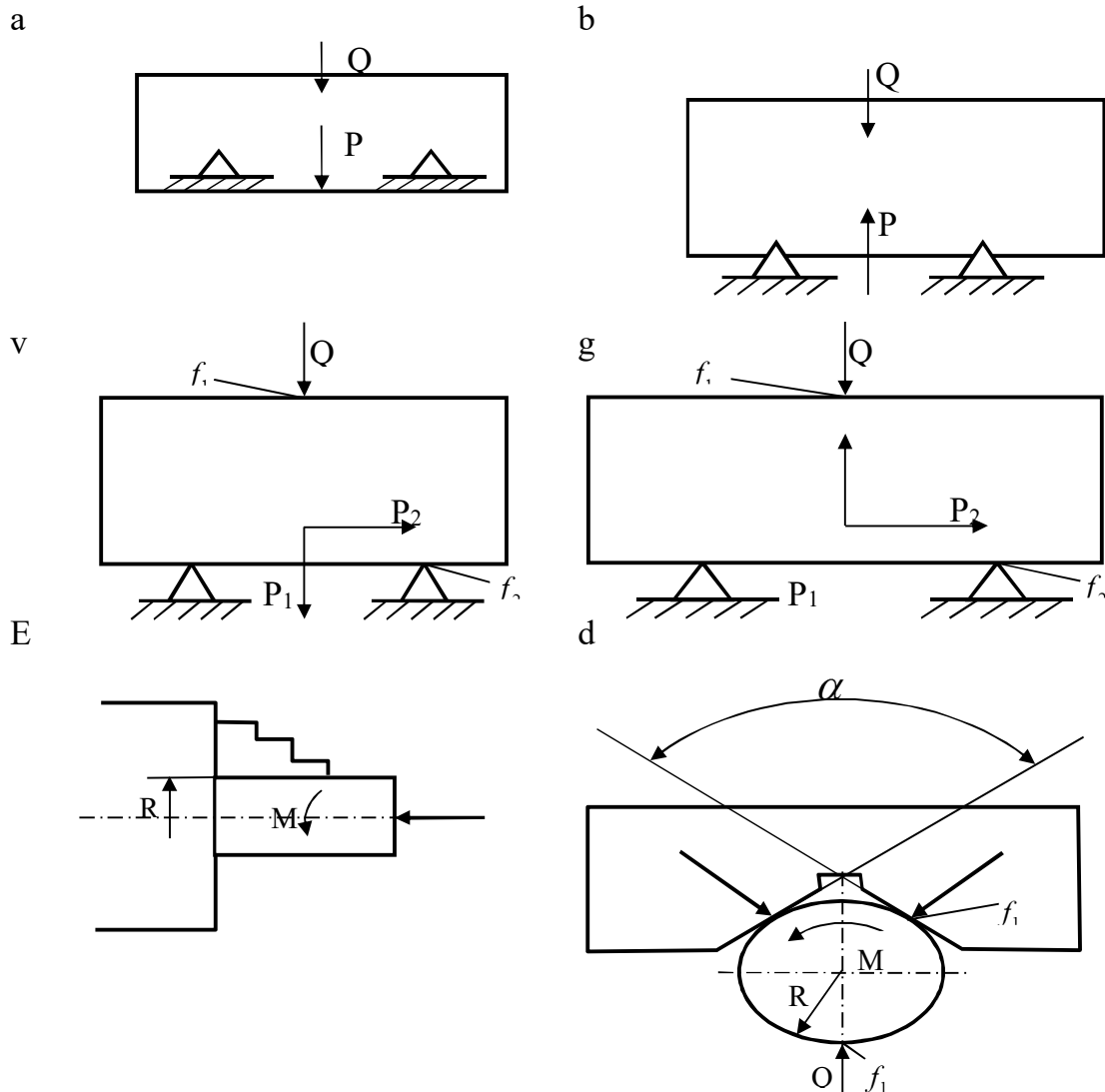
18.10-rasm. Qisuvchi kuchlarni hisoblash sxematari.
