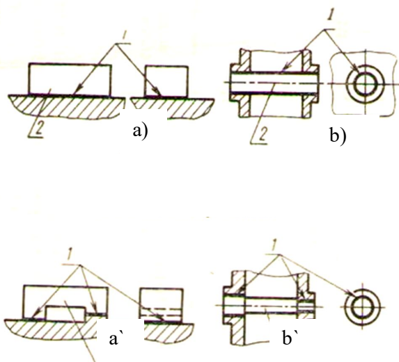
8.1- rasm. Asos turlari. 1-asoslar, 2- tayyorlama qismni.
