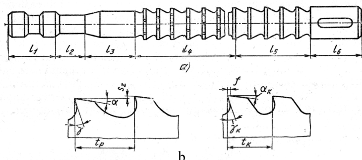
19.18- rasm. Protayjka konstruksiyasi.
