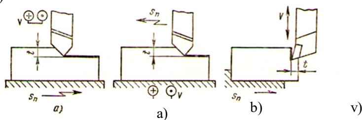
20.1-rasm. Kertish sxemalari.
