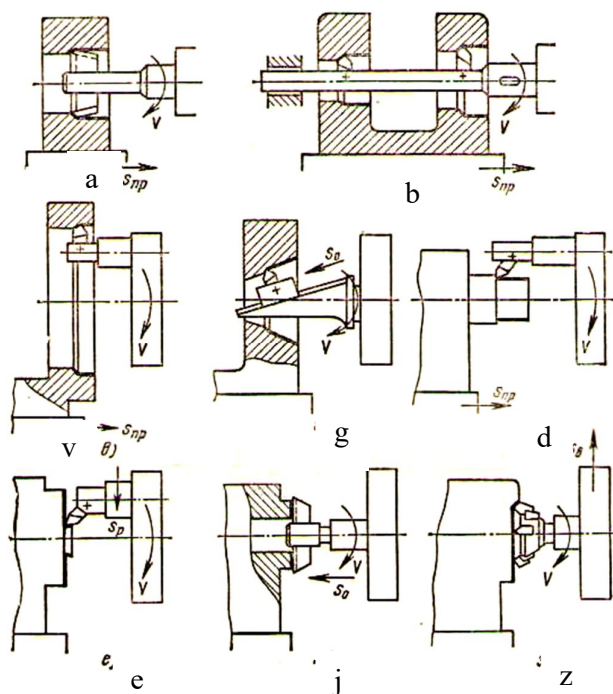
19.12-rasm. Yo'nib kengaytirish jarayoni sxemalari.
