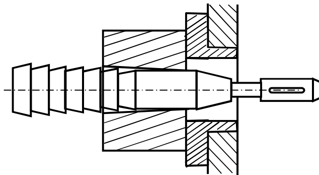
7.19-rasm. Tortib ishlov berishda detalni asoslash shemasi.
