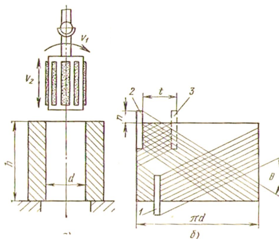
24.7-rasm. Xonlash jarayoni sxemalari.
