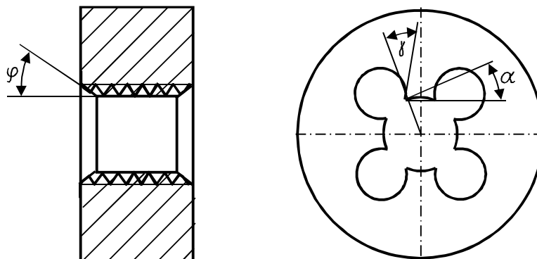
21.5-rasm. Plashkaning konstruktiv ko'rinishi.
