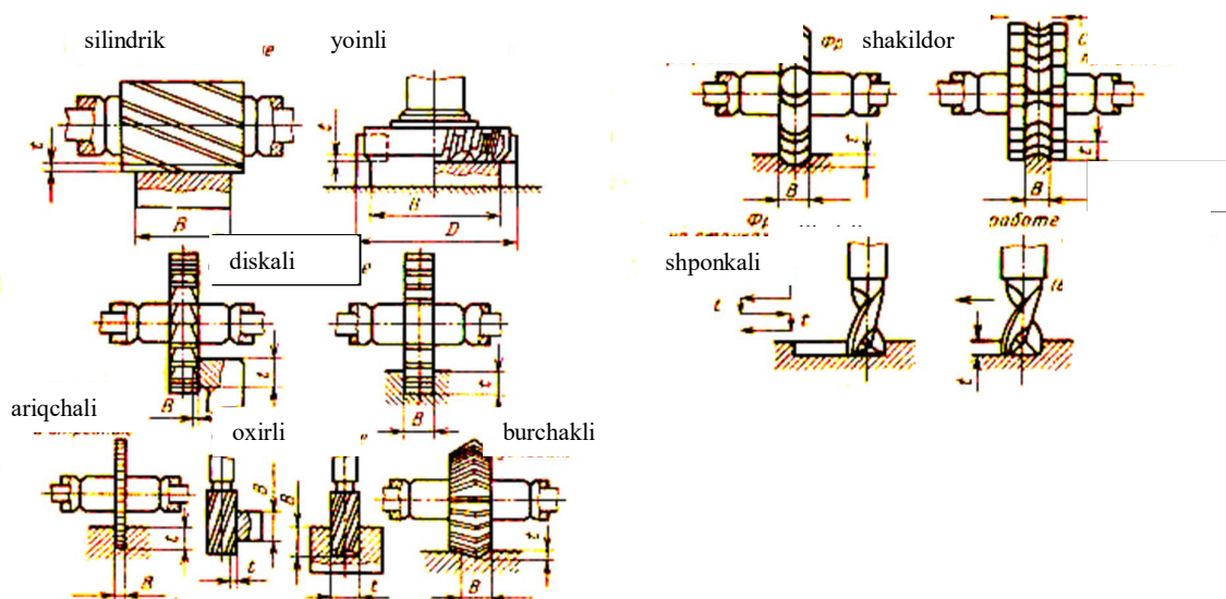
20.5 –rasm. Frezlashdagi kesish chuqurligi va ishlov berish enini aniqlash sxemalari
