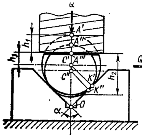
2.19-rasm. Silindrsimon tayyorlamani prizmaga o'rnatish
