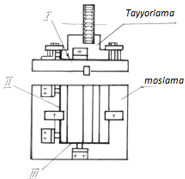
1.5-rasm. 1-tayyorlama; 2- moslama; 1-II-III -texnologik bazalar tuplami.
