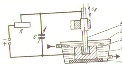
25.5-rasm. Elyekt uchqunida ishlov berish sxemasi.
