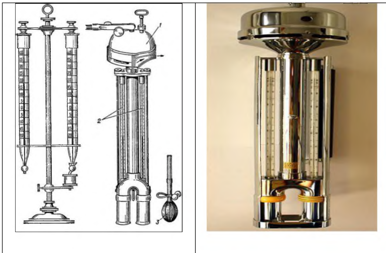
92-расм. Август психрометри ва Ассманн психрометри: 1-вентилятор, 2-психрометр термометри; 3-термометрни намлаш учун ишлатиладиган пипетка.
