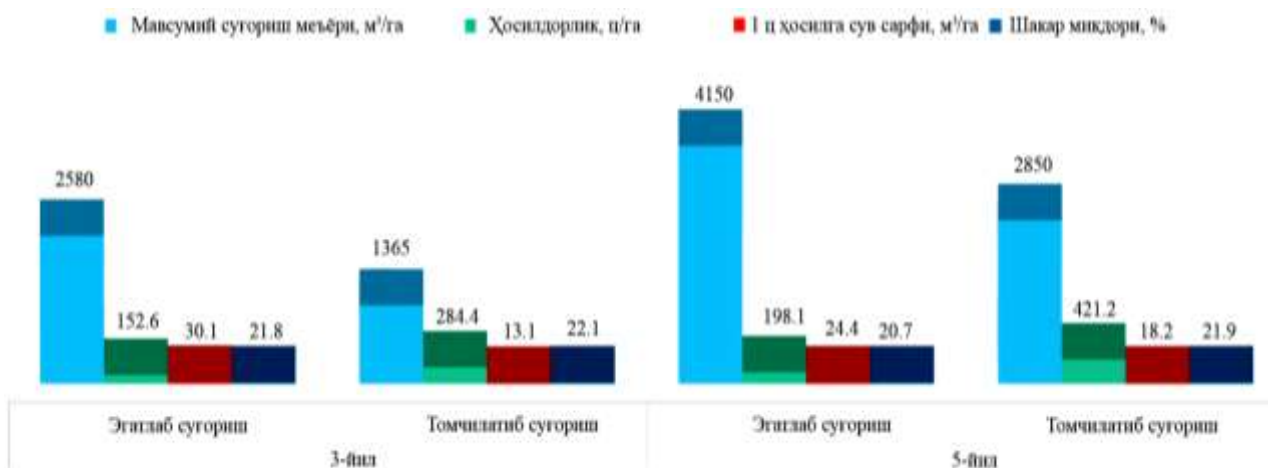
4-расм. Узумни томчилатиб суғоришда олинган натижаларнинг умумлаштирилган графиги
