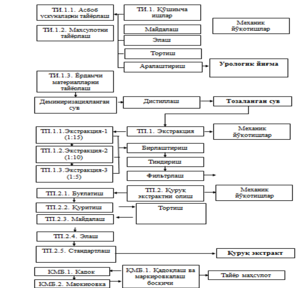
6-расм. Урологик йиғмадан қуруқ экстракт олиш технологик чизмаси
