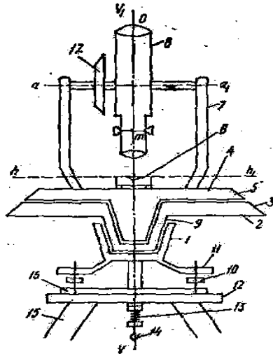
2-shakl. Teodolit sxemasi.
