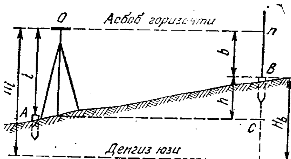
Oldinga nivelirlash.
