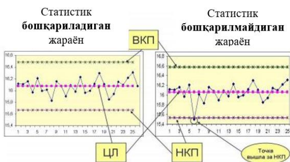
2-расм. Назорат карталари
