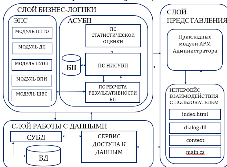
Рис. 7. Многоуровневая функционально-логическая структура программного комплекса автоматизированная интеллектуальная системы управления бизнес процессов
