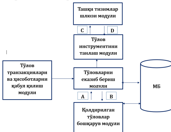
6-расм. Ташкилот электрон тўлов тизимининг структураси.
