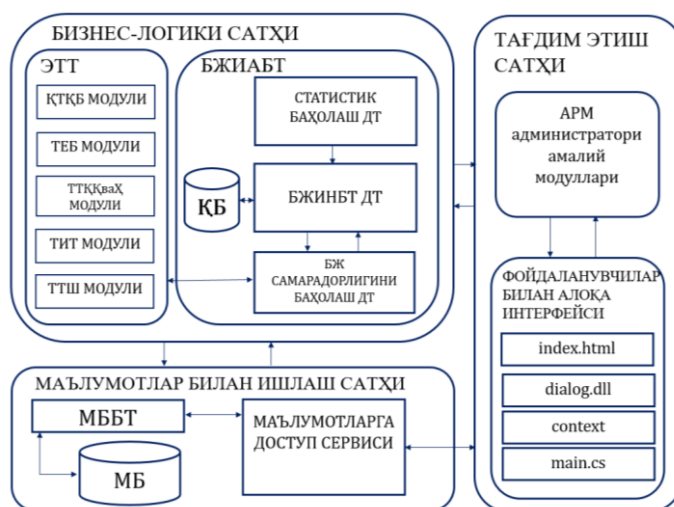
7-расм. Автоматлаштирилган бошқарув тизимининг дастурий мажмуасининг кўп даражали функционал ва мантиқий тузилиши
