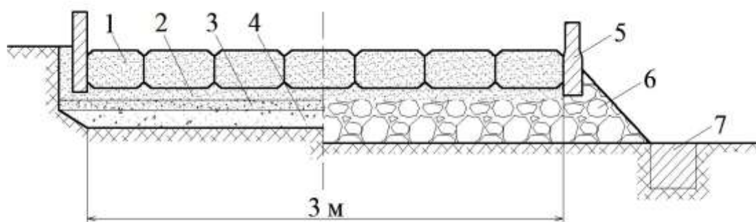
1.2-rasm. Yo'l to'shamasi ko'ndalang kesimi. 1-bazaltli plitalar 80x40x50sm; 2-10 va 15 sm shag'al qatlami; 3-15 sm loy aralashli chaqiq tosh; 4-sement bilan mustahkamlangan shag'al; 5-bardyr toshi 6-60 sm qalinlikdagi loy shag'al aralashmasi; 7-tayanch tosh.
