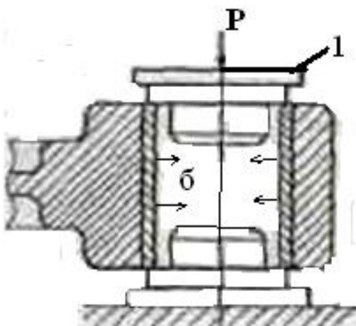
10.2-rasmda shatunning yuqori kallagidagi bronza vtulkani cho'ktirish sxemasi.
