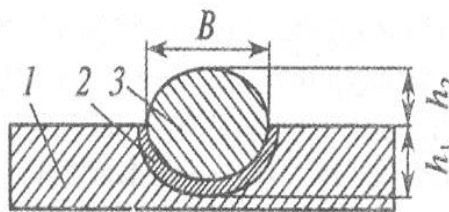
3-rasm. Payvand chok ko'ndalang kesim yuzasi:
