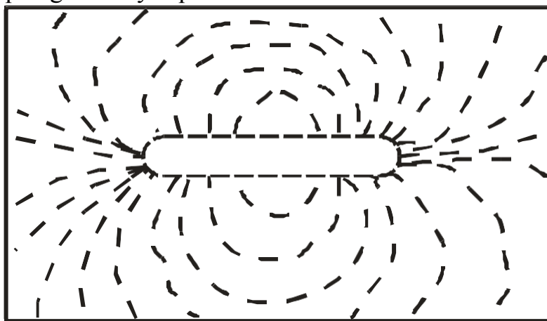
4.4- rasm. Darz bor joyning perimetri bo'yicha kukunli maydoncha hosil bo'lish sxemasi
