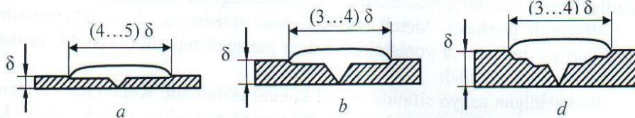
7.1-rasm. Qalinligi har xil bo'lgan cho'yan detallarni jez bilan kavsharlash uchun chok o'lchamlari:
