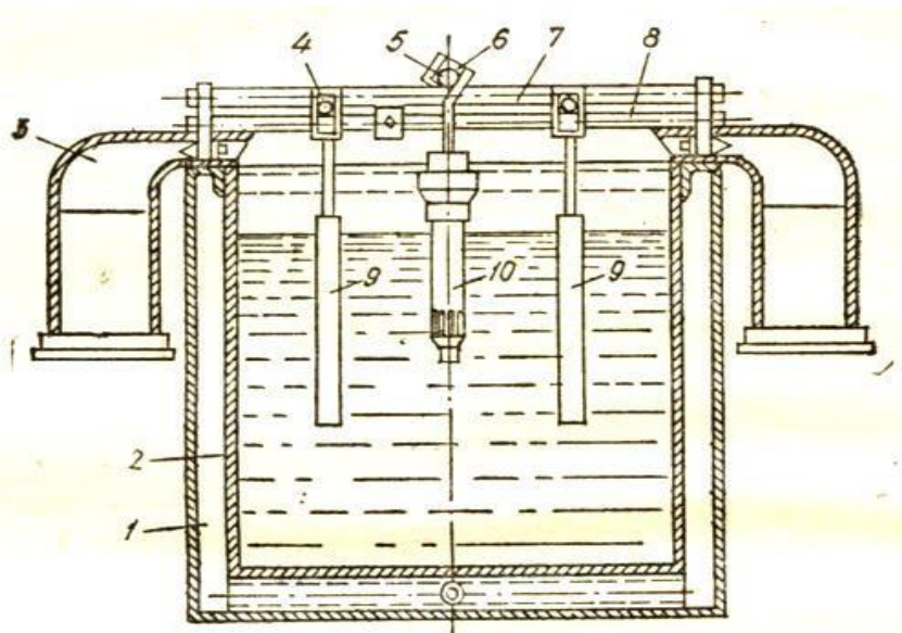
9.5-rasm. Detallarni xromlash vannasiga osish chizmasi.
