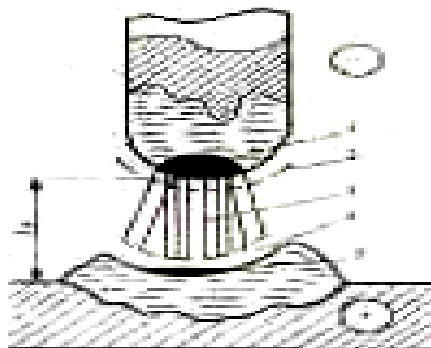
7-rasm. Payvandlashdagi etektr yoyining tuzilish sxemasi
