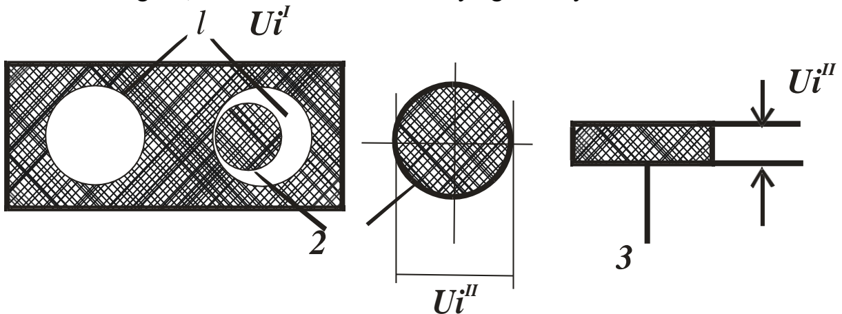
2.3- rasm. Detallar geometrik parametrlarining o'zgarish variantlari. 1 – bo'yincha (vtulka), 2 – val, 3 – disk; avtomobil ish jarayonida: U_i^I – kattalashadi; U_i^{II} – kichrayadi.
