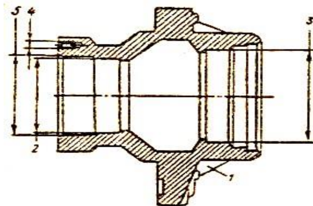
12.9-rasm. G'ildirak gupchagining nuqsonlari: 1-darzlar va sinishlar; 2,3- podshipnik; 4-rezbalni teshiklarning yeyilishi; 5-salnik turgan teshiklarning yeyilishi.
