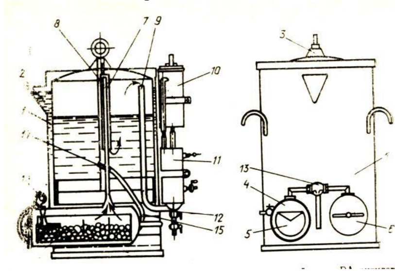
8.3-rasm. Karbidga suv ta'sir ettirish yo'li bilan ishlaydigan atsetilen generatori.
