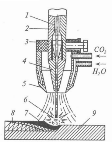
1-rasm. Karbonat angidrid gazi muhitida suyuqlantirib qoplama qoplash kallagining sxemasi:
