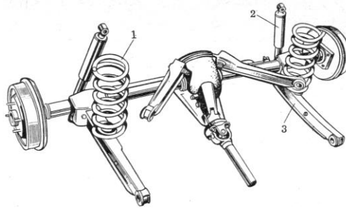
6.4-rasm. Prujinali nomustaqil osma 1-prujina; 2-amortizator; 3-shtanga.
