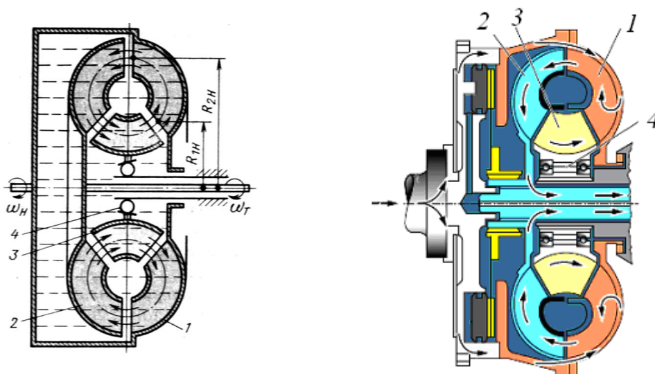
4.8-rasm. Gidrotransformator sxemasi va ishlash printsipi
