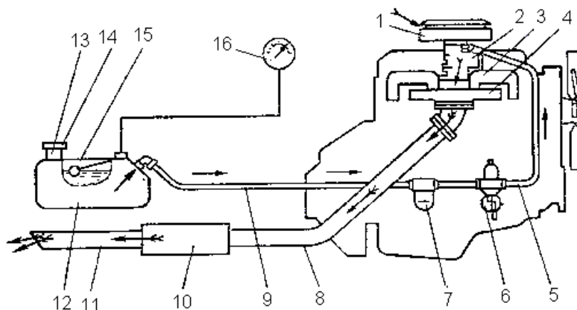
3.1-rasm. Karbyuratorli dvigatel ta'minlash tizimining sxemasi.
