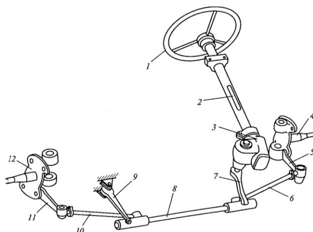
6.10-rasm. Mustaqil osmali avtomobil rul boshqarmasi sxemasi
