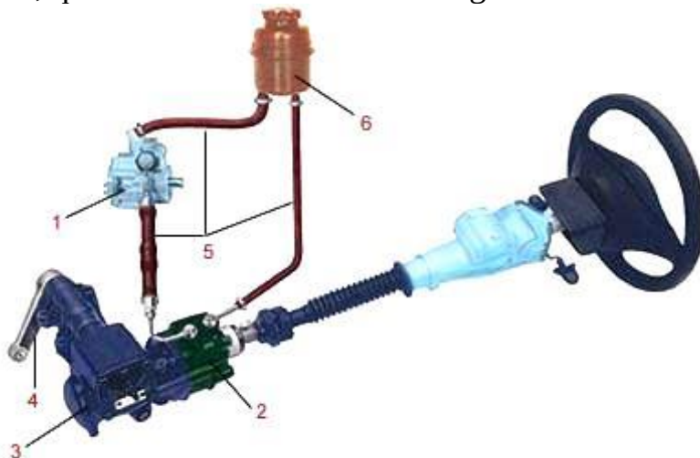
6.11-rasm. Gidrotsilindri rul mexanizmi bilan bir korpusda joylashgan gidrokuchaytirgich: 1 – nasos; 2 – taqsimlagich korpusi; 3 – rul mexanizmi; 4 – rul soshkasi; 5 – shlanglar; 6 – bachok.
