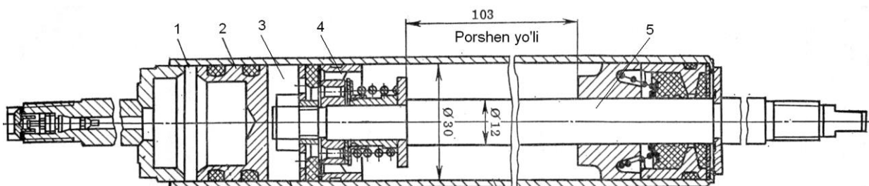
6.6-rasm. Bir trubali teleskopik amortizator:
