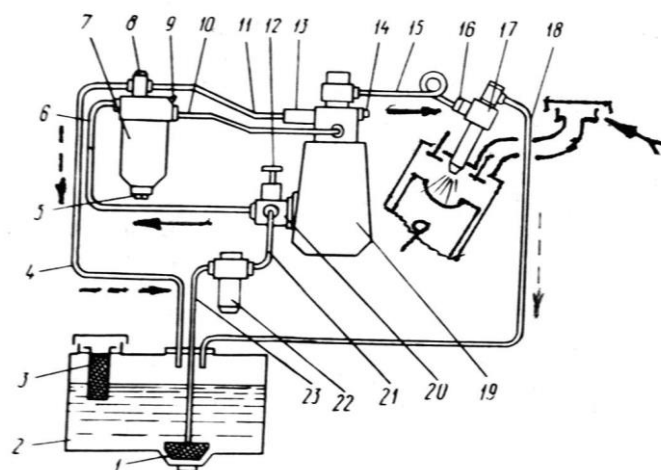
3.7-rasm. Dizel ta'minlash tizimining umumiy sxemasi.
