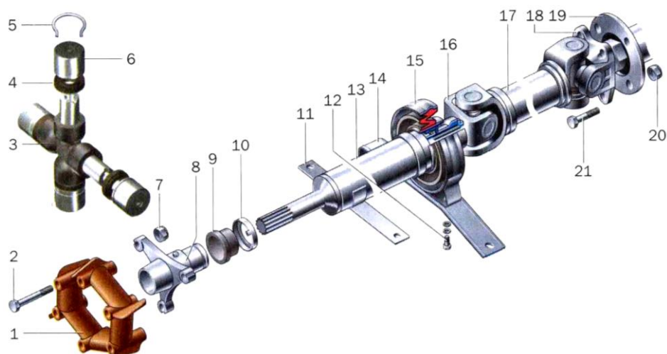
5.2-rasm. Kardanli uzatma: 1- elastik mufta; 3- krestovina; 4- sal'nik; 5- cheklagich xalqa; 6- krestovina podshipnigi; 8- elastik mufta flanetsi; 13- oldi kardan vali; 15- oraliq tayanch; 16- oldi kardan vali vilkasi; 17- ketingi kardan vali; 18- ketingi kardan vali vilkasi; 19- asosiy uzatma yetakchi valining flanetsi.
