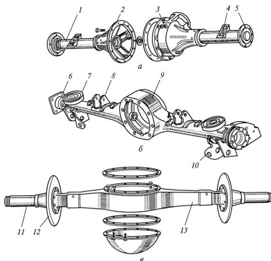
6.1-rasm. Yetakchi ko'priklar:
