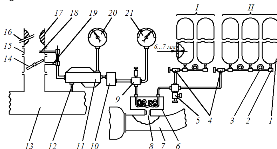
3.3-rasm. Gaz ballonli qurilmaning printsipl sxemasi.
