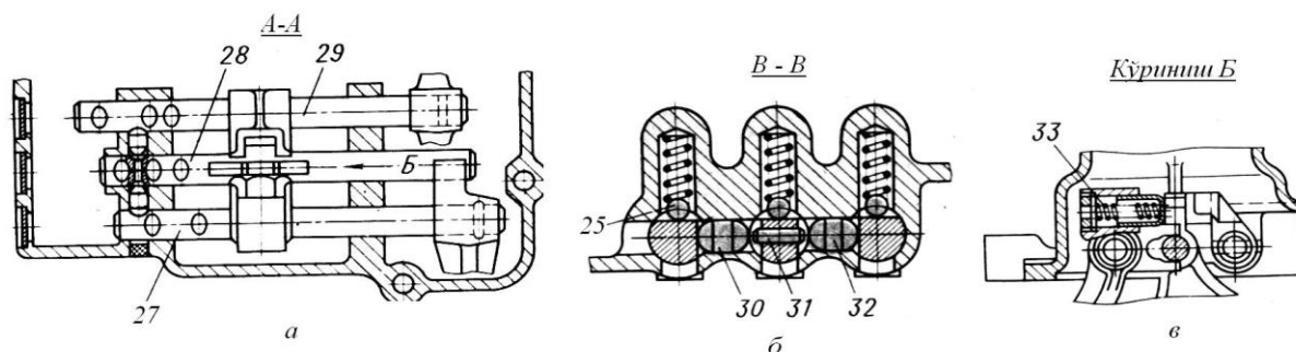
4.7-rasm. Uch pog'onali uzatmalar qutisi pog'ona almashtirish mexanizm qismlari
