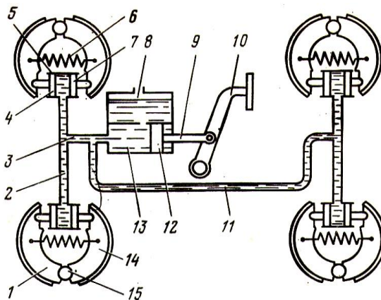
7.12-rasm. Gidravlik tormoz yuritmasining soddalashtirilgan sxemasi:
