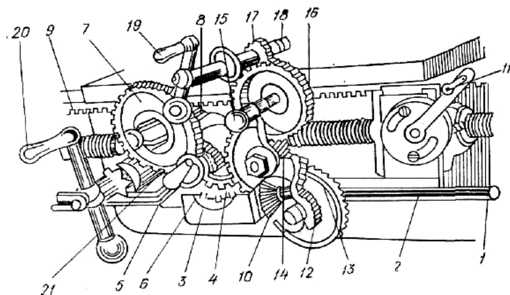
68-рasm. Станок фартути.
