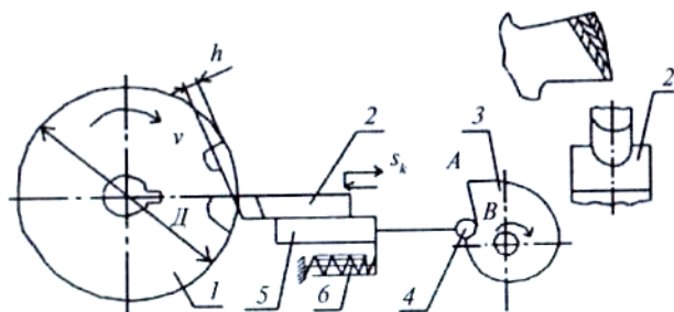
1-rasm. Freza orqa yuzasini gardanlash sxemasi.
