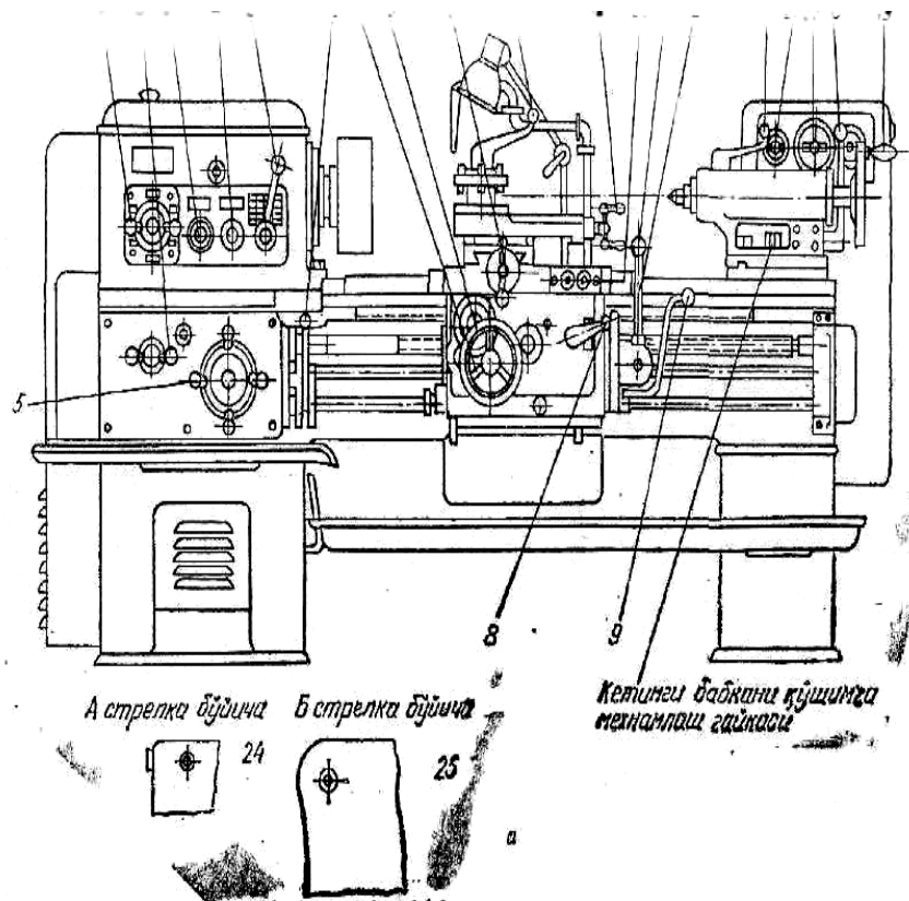
64-расм. 1К62-моделли токарлик винт қирқар станогининг умумий кўриниши (а) ва кинематик схемаси. (б) 1,2 — шпинделни айлантирилари сонини ростлаш дасталари; 3 — нормал ва опирилган қадамли резбобалар кесинида ростловчи дастаси; 4 — ўнақай ёки чалақай резбоба қирқинида ростлаш дастаси; 5 — кесиладиган резбоба қадамини суриш тезлигини ростлаш дастаси; 6 — резбоба кесинида тегишли тезликка юргизиш винтини улаш дастаси; 7 — суппортни буйлама юрадиган салазка маховикчаси; 8 — юргизиш винтга ажраладиган гайка улаш ёки ажратувчи дастаси; 9, 10 — шпинделни айлантириш ва айланиш томонини ўзгартувчи дасталари; 11 — суппорт салазкаларини буйлама ва кўндаланг йўналишларга жадал юргизиш кнопчаси; 12 — суппортни буйлама ва кўндалангига юрадиган салазкаларининг
