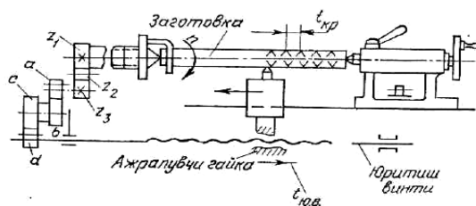
75-расм. Токарлик станокда шпинделдан юргизиш винтига ҳаракат узатиш схемаси.
