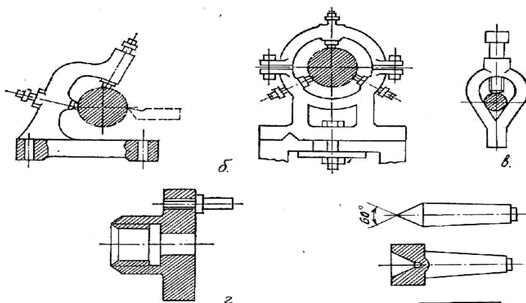
а — үч кулачокли патрон ва план шайба; б — люнет; в — хомут; г — оправка; д — маркалар.
