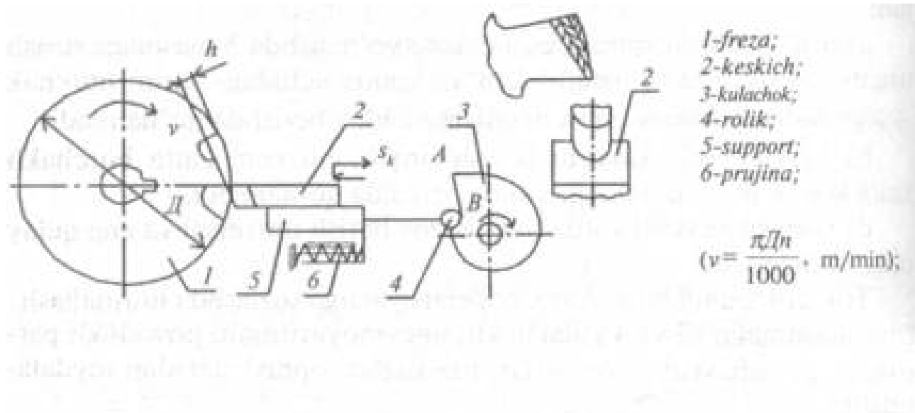
I-rasm. Freza orqa yuzasini gardanlash sxemasi.
