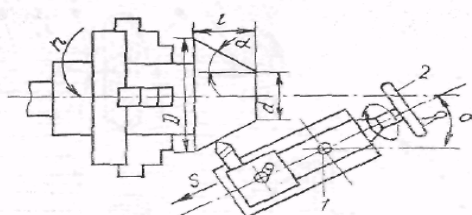
71- рasm. Суппорт устки салазаксини бурни билан конусавий юзларни йўниш: 1 — устки салазка; 2 — даста.
