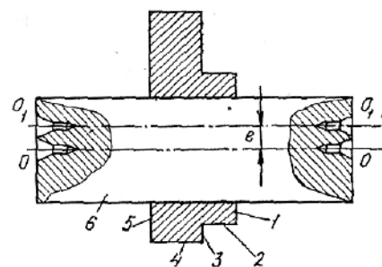
73-расм. Доирaviй эксцентрик юзалар-ни ишлашда заготувканинг ишлаш схе-маси.
