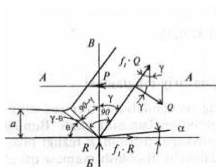
4.4-rasm. Keskich tig'iga ta'sir etuvchi kuchlar sxemasi.
