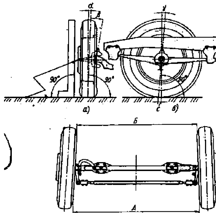
52-rasm. Boshqariladigan g'ildiraklarni o'rnatish shakli: a-og'ish \alpha va shkvorenning ko'ndalang qiyalik R burchaklari; b-shkvorenning bo'ylama qiyalik u burchagi; v-g'ildiraklarning yaqinlashuv masofasi
