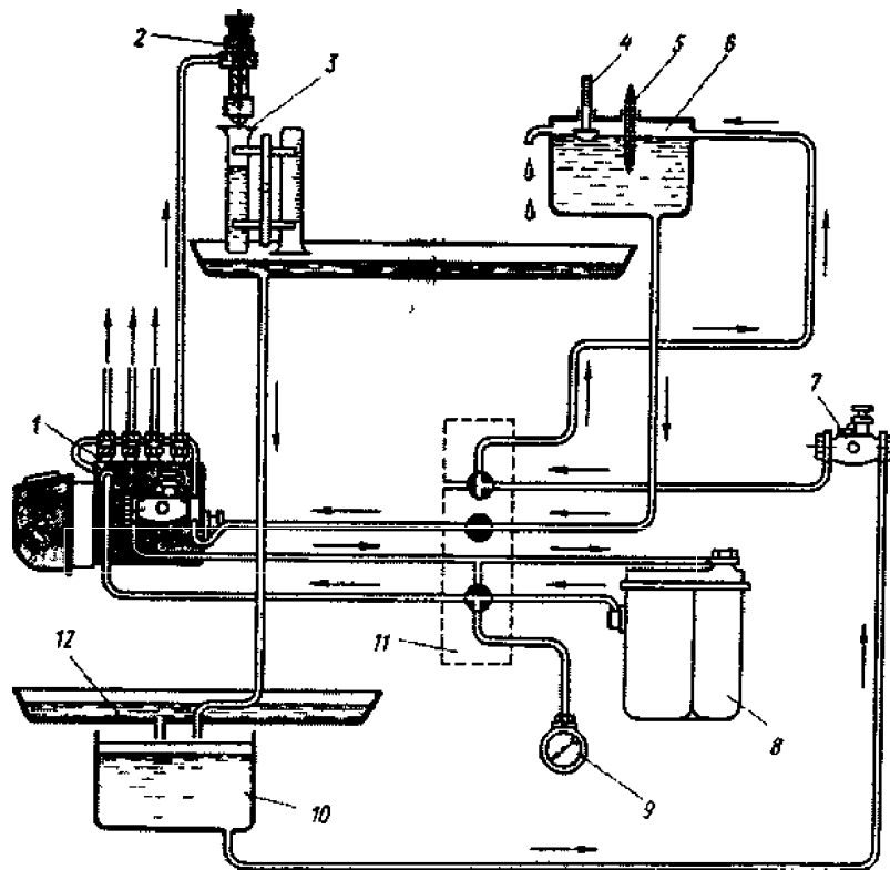
38-rasm. Yonilg'i nasoslarini tekshirish jihozining ishlash shakli: 1-yuqori bosimli yonilg'i nasosi, 2-etalon forsunka, 3-menzurka, 4-yonilg'i sathini ko'rsatkich, 5-termometr, 6, 10-yonilg'i bakchalari, 7-jihozning yonilg'i haydash nasosi, 8-filtr, 9-manometr, 11-kranlar, 12-yonilg'ini to'plovchi vanna
