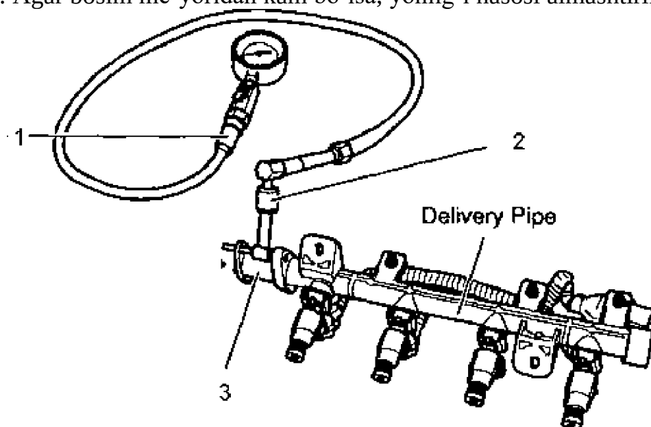
35-rasm. Yonilgʻi taʼminot tizimidagi bosimni tekshirish: 1-manometr; 2- ulagich; 3-quvuroʻtkazgich.
