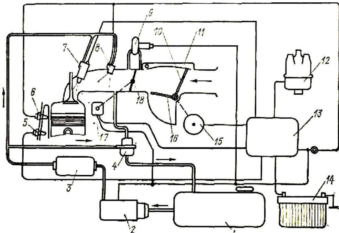
33-rasm. Benzinli purkash (injektorli) ta'minot tizimi sxemasi 1-yonilg'i baki; 2-elektr benzin nasosi; 3-filʼtr; 4-reduksion klapan; 5-temperatura datchigi; 6-temperatura datchigi; 7-elektromagnit klapani (injektor); 8-ishga tushirish elektromagnit klapani; 9-qayta o'tkazish klapani; 10-buriluvchi plastinka; 11-baypas kanali; 12-o't oldirish tizimi; 13-elektron blok; 14-akkumulyator batareyasi; 15-
