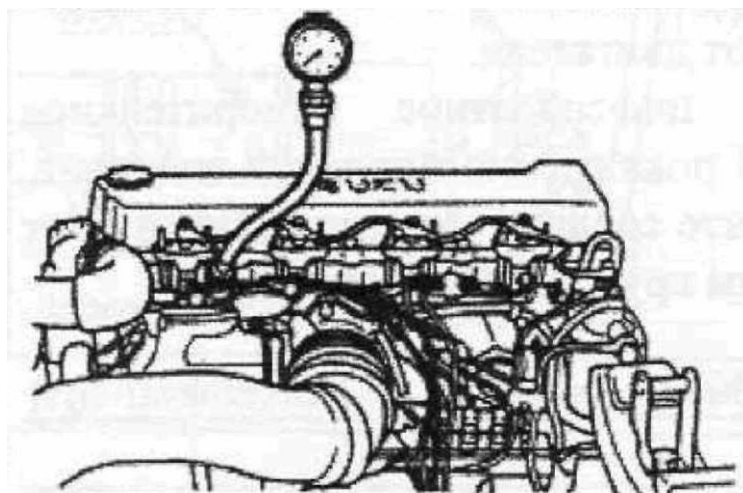
14-Rasm. Manometrli (a) va o'zi yozuvchi (b) kompressometrlar hamda Isuzu avtomobili dvigateling kompressiyasini o'lchash shakli (s).
