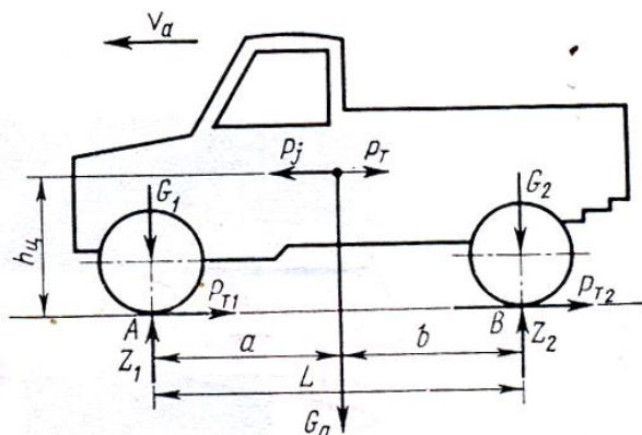
11.1-rasm. Avtomobilning yelkanlik markazining koordinatalari.
