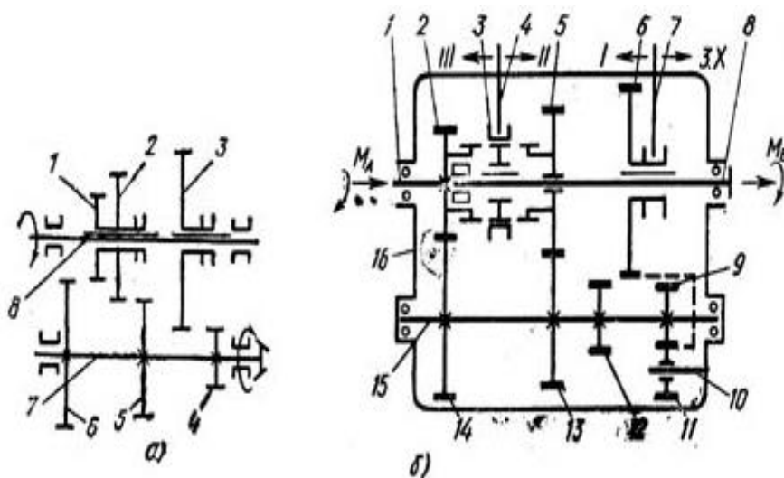
4.3-rasm. Uzatmalar qutisining tasviri chizmasi.
