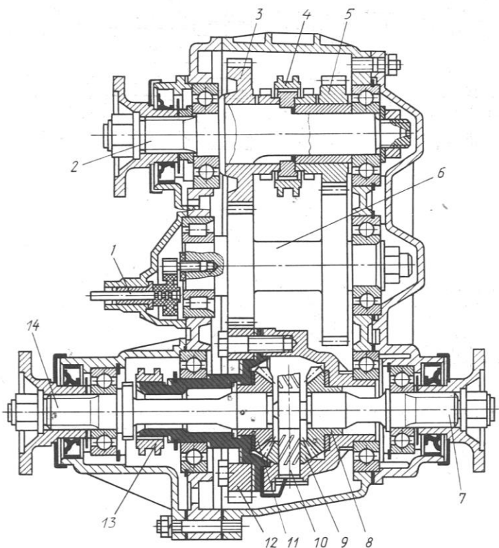
12.5-rasm. VAZ-2121 «Niva» avtomobilining taqsimlash qutisi: 1-spider yuritmasi; 2-etkachi val; 3-yuqori uzatma shesternyasi; 4-uzatmalarni qo'shish muftasi; 5-quyi uzatma shesternyasi; 6-oraliq val; 7-orqa ko'prikn yuritmasi vali; 8 va 11-differentsial shesternyasi; 9-differentsial satelliti; 10-satellit o'qi; 12-differentsial korpusi tishli g'ildiragi; 13-differentsial blokirovkasi muftasi; 14-old ko'prikn yuritmasi vali.
