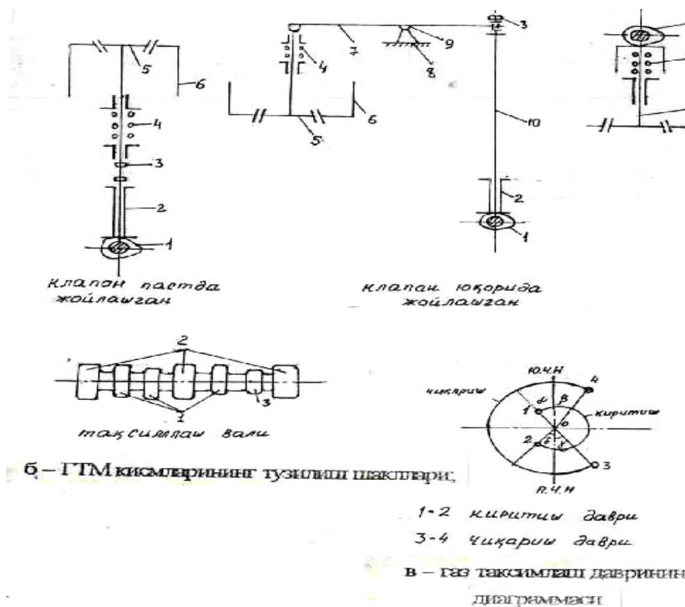
2.2-rasm. GTM qismlarining shakllari va gaz taqsimlash davrining diagramasi.
