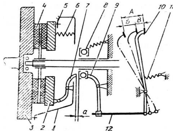
4.1-rasm. Bir diskali friktsion quymali ilashish muftasining tasviriy chizmasi.
