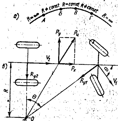
24.3-rasm. Avtomobilning burilishi. a) burilish jarayoni davrlari; b) burilishda ta'sir etuvchi kuchlar.
