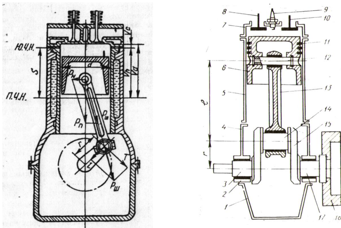
3.2-rasm. Porshenli ichki yonuv dvigatelning tuzilishi. A- ko'ndalang ko'rinish, B-bo'ylama ko'rinish.
