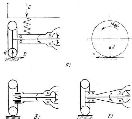
14.7-rasm. Yarim o'qlarning orqa ko'prikda joylanish usullari a – yarim yuksizlantrilgan, b – \frac{3}{4} qismi yuksizlantirilgan, v – to'la yuksizlantrilgan
