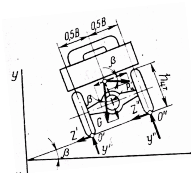
24.7-rasm. Ko'ndalang qiya tekislikda harakatlanayotgan avtomobilga ta'sir etuvchi kuchlar
