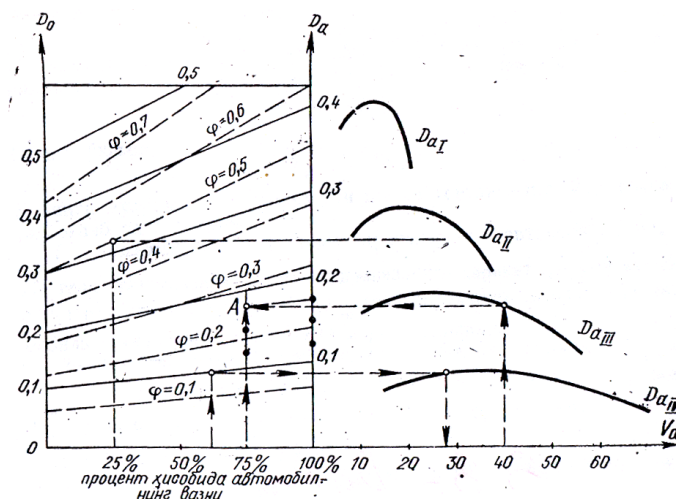
5.1-rasm. Avtomobilning dinamik pasporti grafifi.
