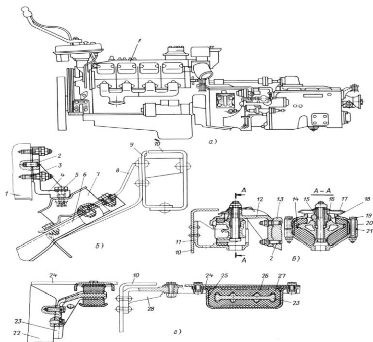
4.6-rasm. KamAZ-5320 avtomobili dvigatelinig maxkamlanishi: a-dvigatel; b-old tayanch; v-orqa tayanch; g-ushlab turuvchi tayanch; 1-tsilindrlar bloki; 2-shtift; 3-shpilka; 4,8,23 va 28-kronshteynlar; 5,15 va 19-boltlar; 6-tortgich; 7,14 va 27-rezina yostiqlar; 9-ustun; 10-rama lonjeroni; 11-orqa tayanch kronshteyni; 12-dvigatel kronshteyni; 13-maxovik karteri; 16-barmog; 17-himoya qalpog'i; 18-vtulka; 20-qopqog; 24-rostlovchi qistirma; 22-uzatmalar qutisi karteri; 24-ko'ndalang list; 25-yostiqlarning oboymasi; 26-yostiqlarning nakladkasi.
