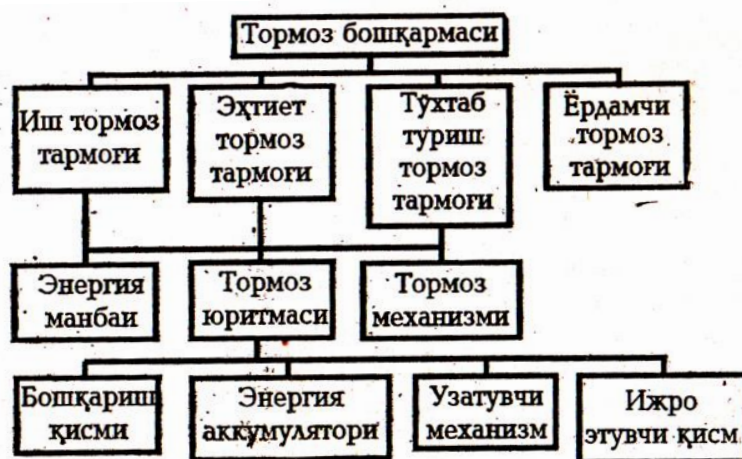
8.1-rasm.Tormoz boshqarmasini muvofiqlashtirilgan tasviriyl chizmasi
