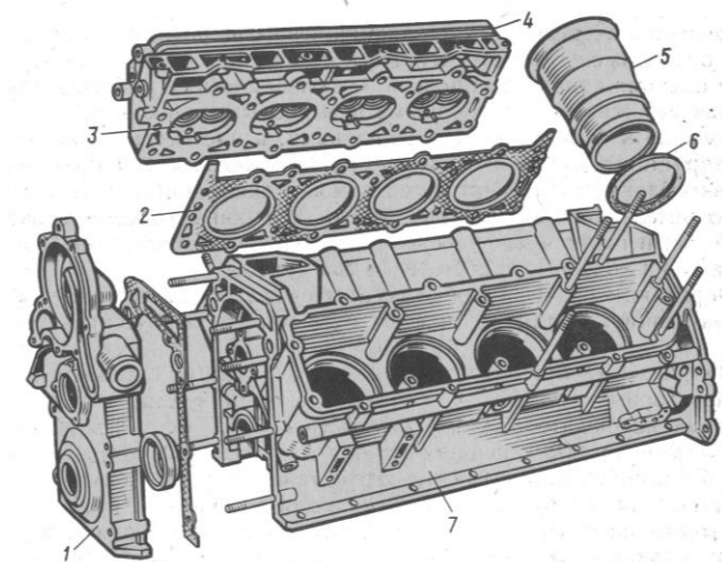
4.5-chizma. V-simon dvigatelning blok karteri va tsilindrlar bloki kopkog'i.
