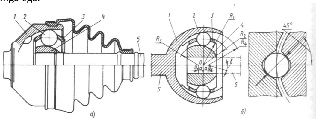
13.4-rasm. (Birfil turidagi) Olti sharikli kardan sharniri: a – konstruksiyasi; b – sxemasi; 1-korpus; 2-shariklar; 3-separator; 4-mushtcha; 5-val.
