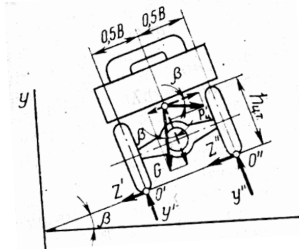
24.9-rasm. Avtomobilni qiyalikda burilish paytidagi turg'unligi.
