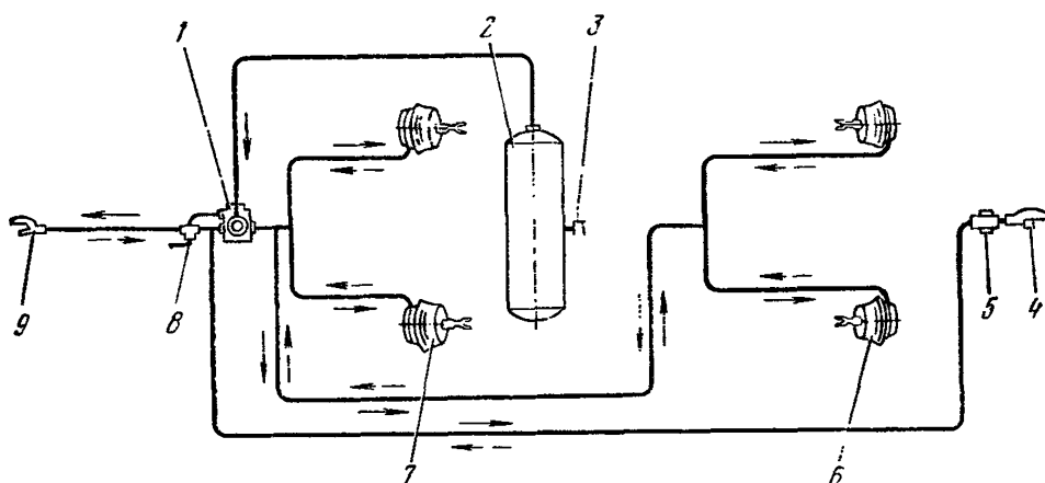
10.1-rasm. Tirkamaning pnevmatik tormoz tizimi sxemasi
