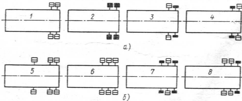
7.2-rasm Yarim tirkamalarning komponovka sxemalari.
