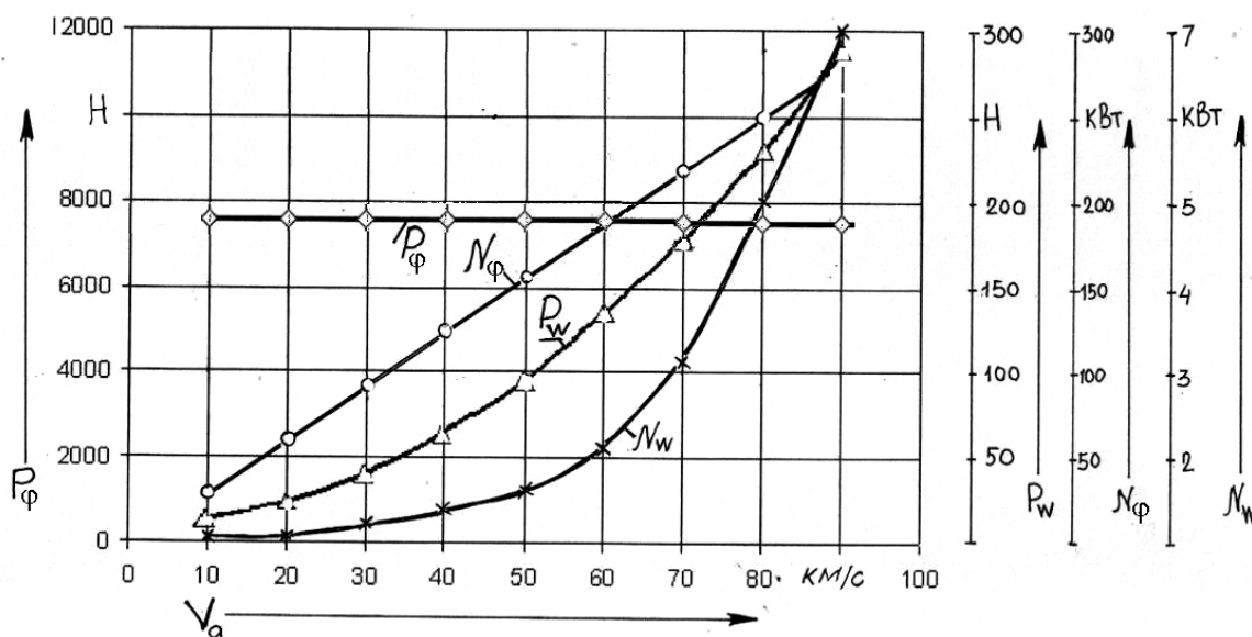
6-rasm. Avtomobilga ta'sir qiluvchi kuch va saflanayotgan quvvatlar 9.2 Avtomobilning 100 km yo'lga sarflaydigan yonilg'i sarfi
